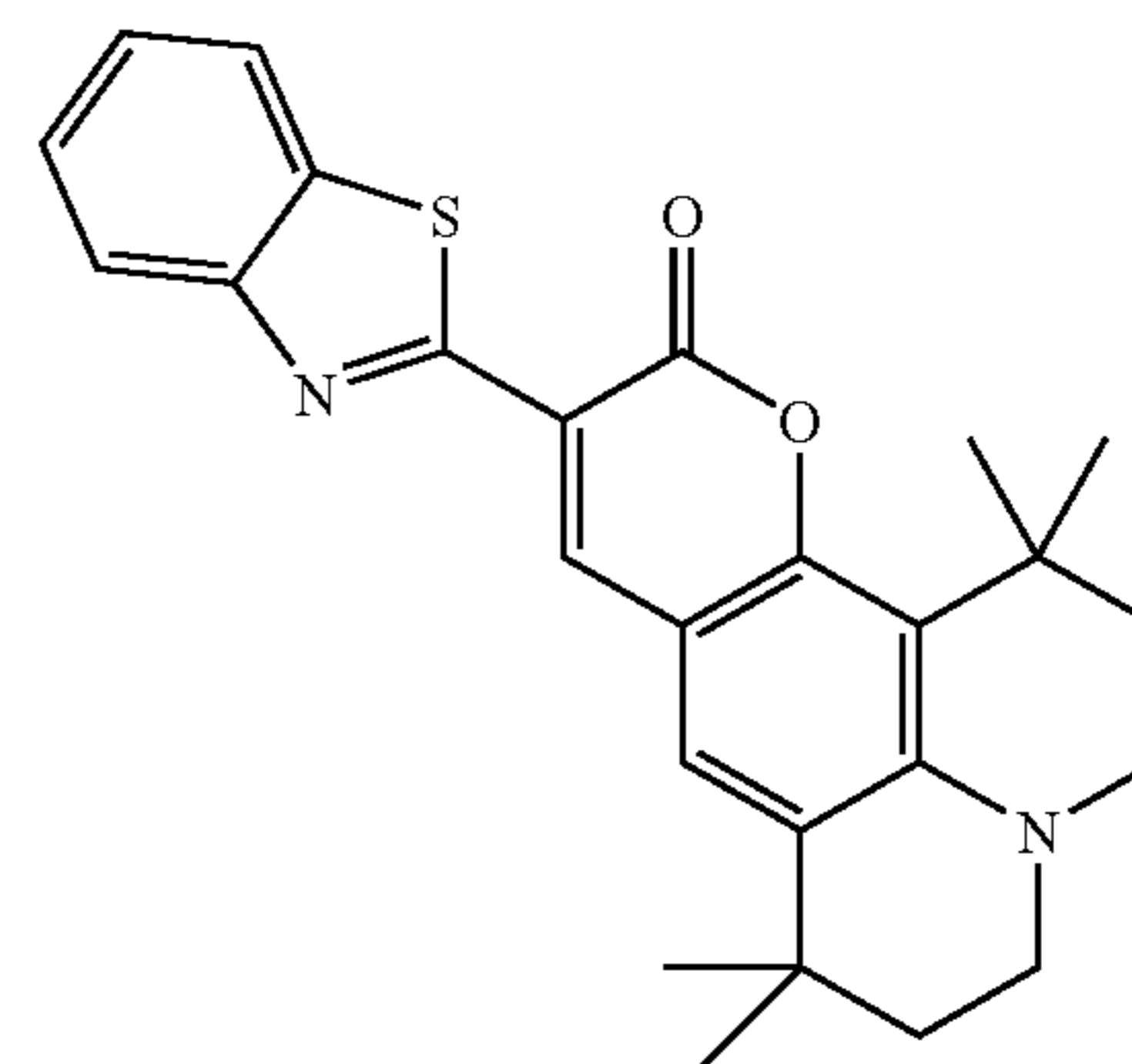
C-545T
