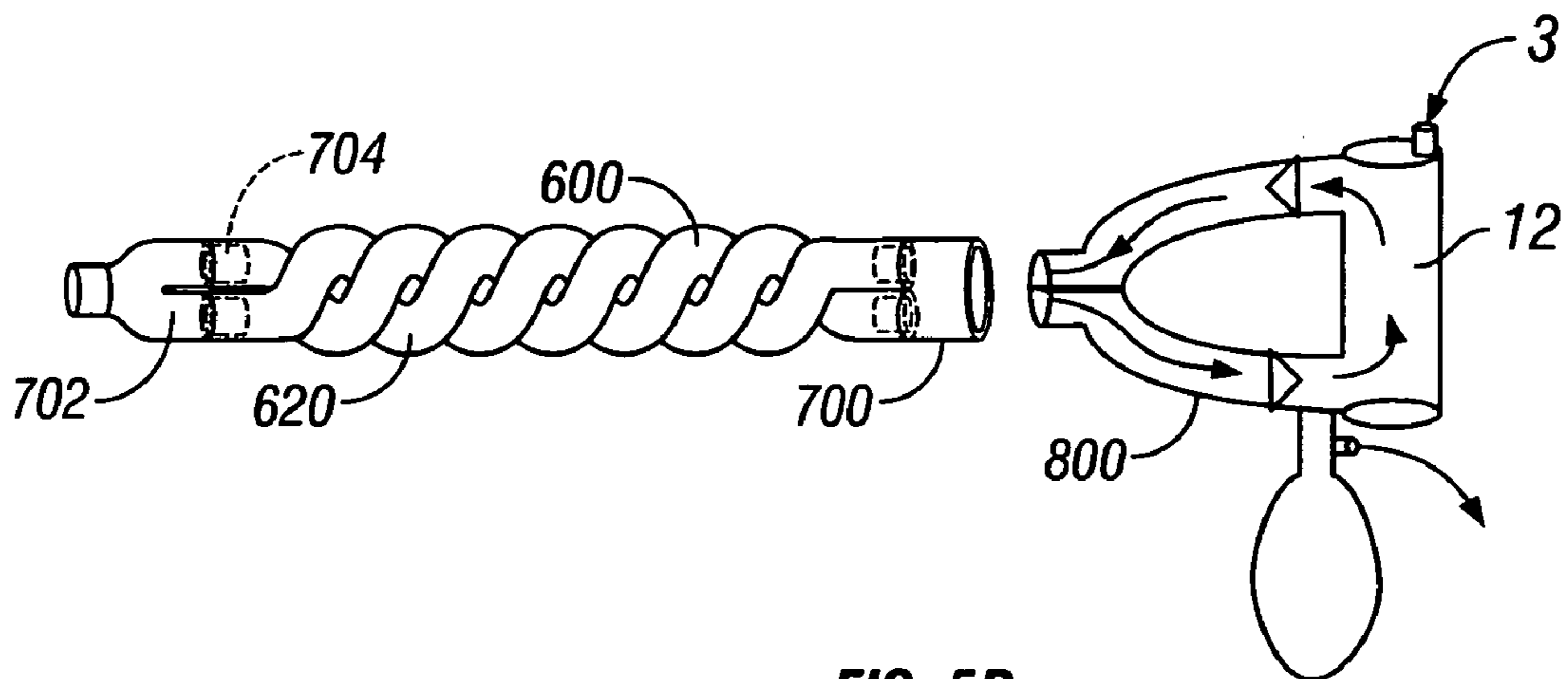
FIG. 5D
