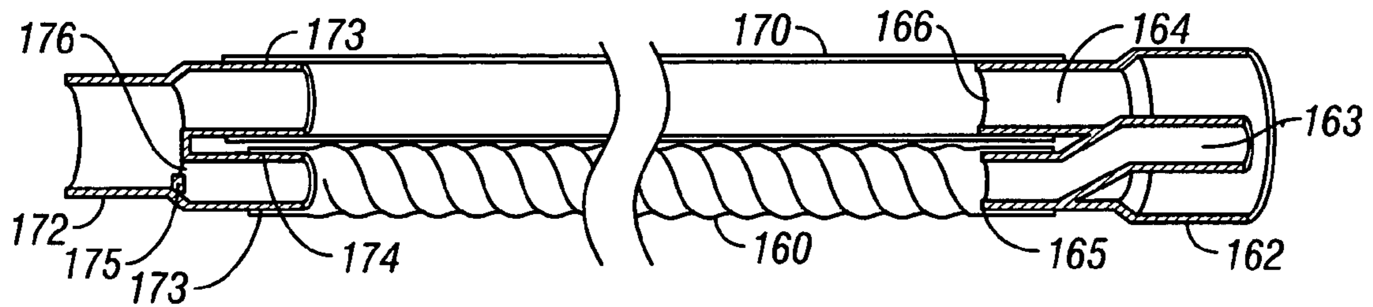
FIG. 11
