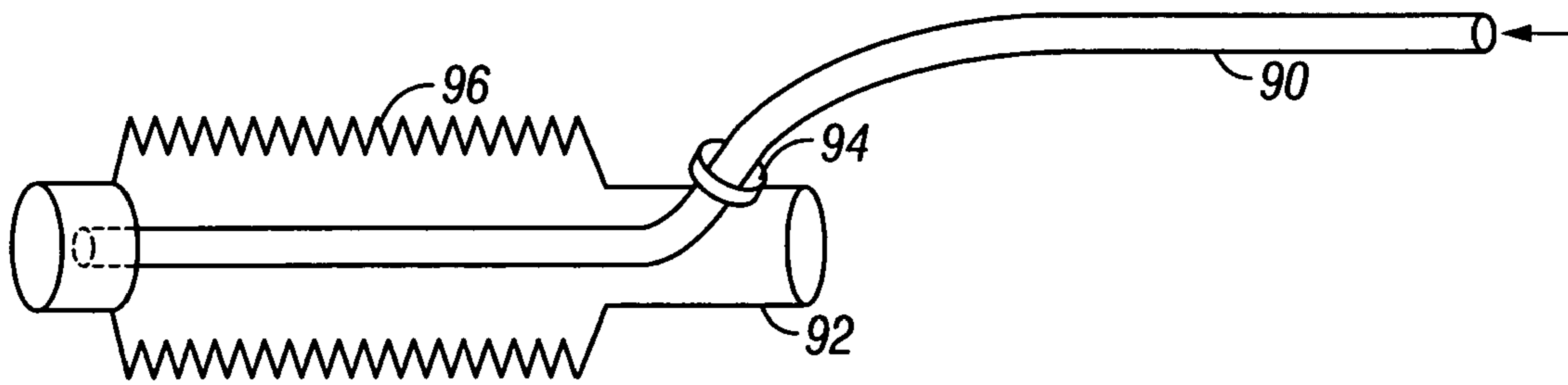
FIG. 6A
