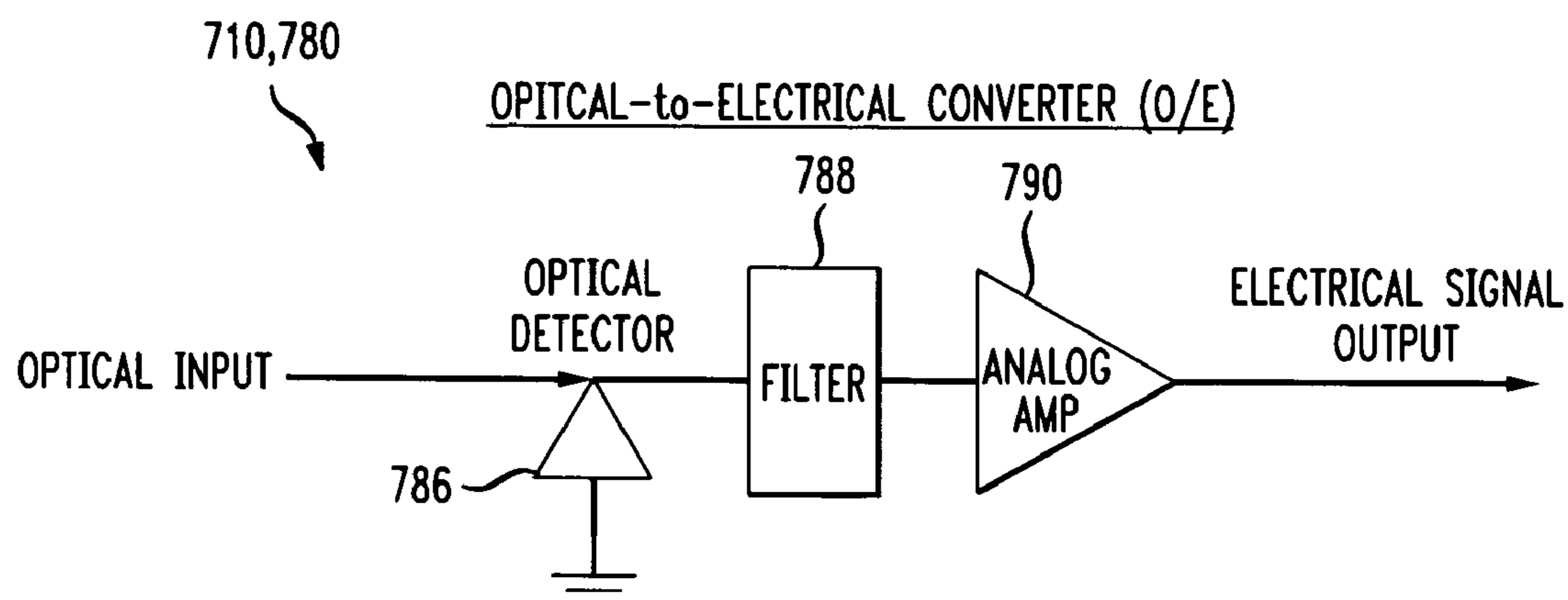
FIG. 10A
