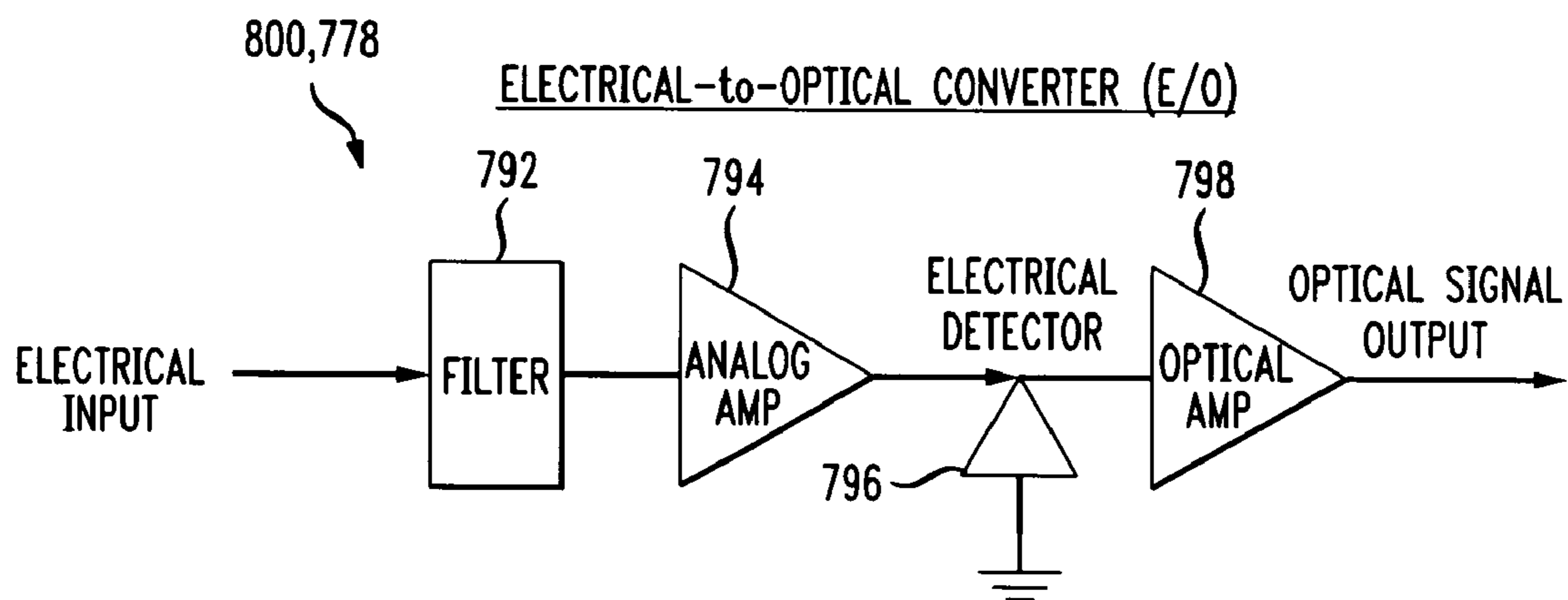
FIG. 10B
