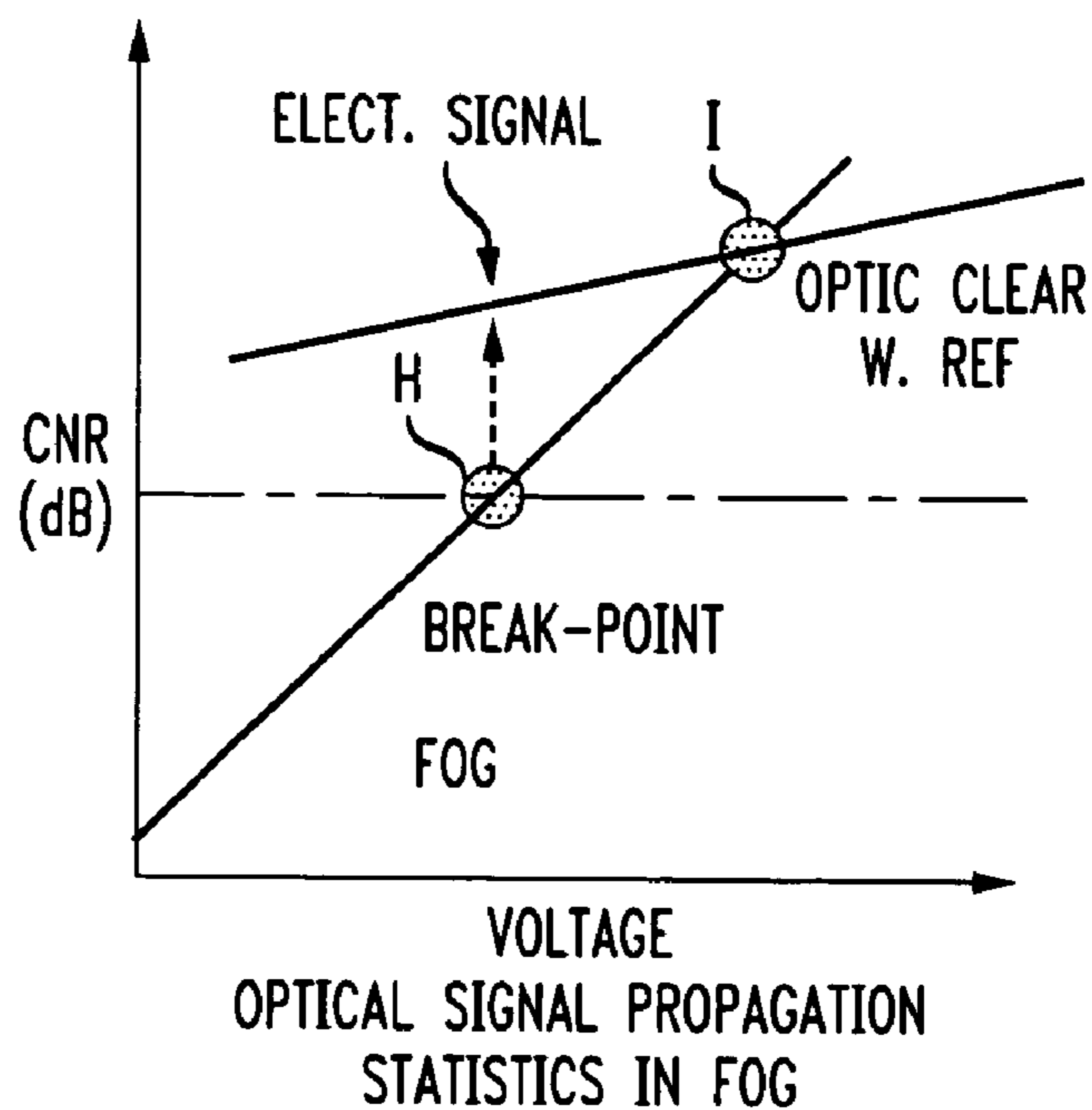
FIG. 8B
