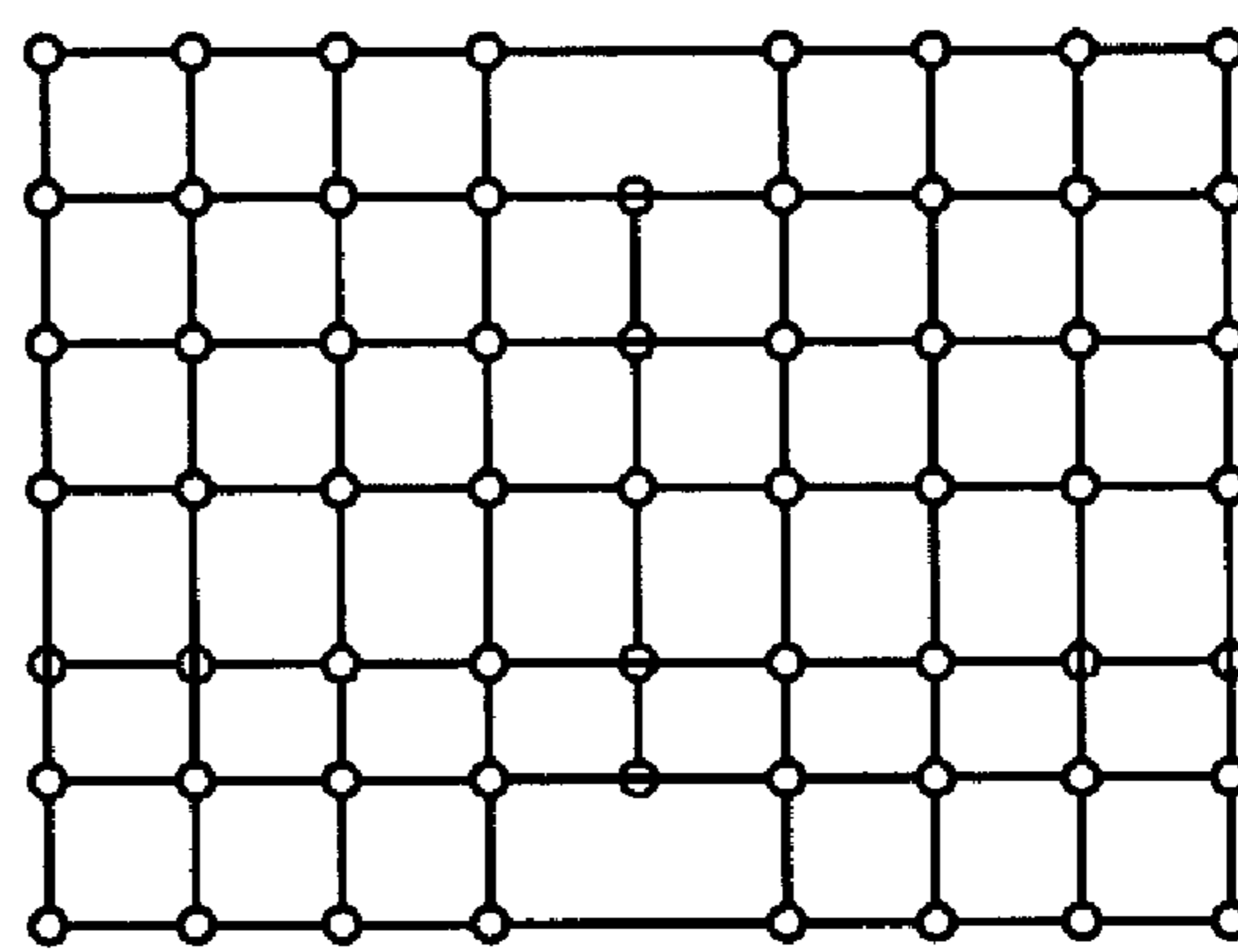
b. Bezier domains.
