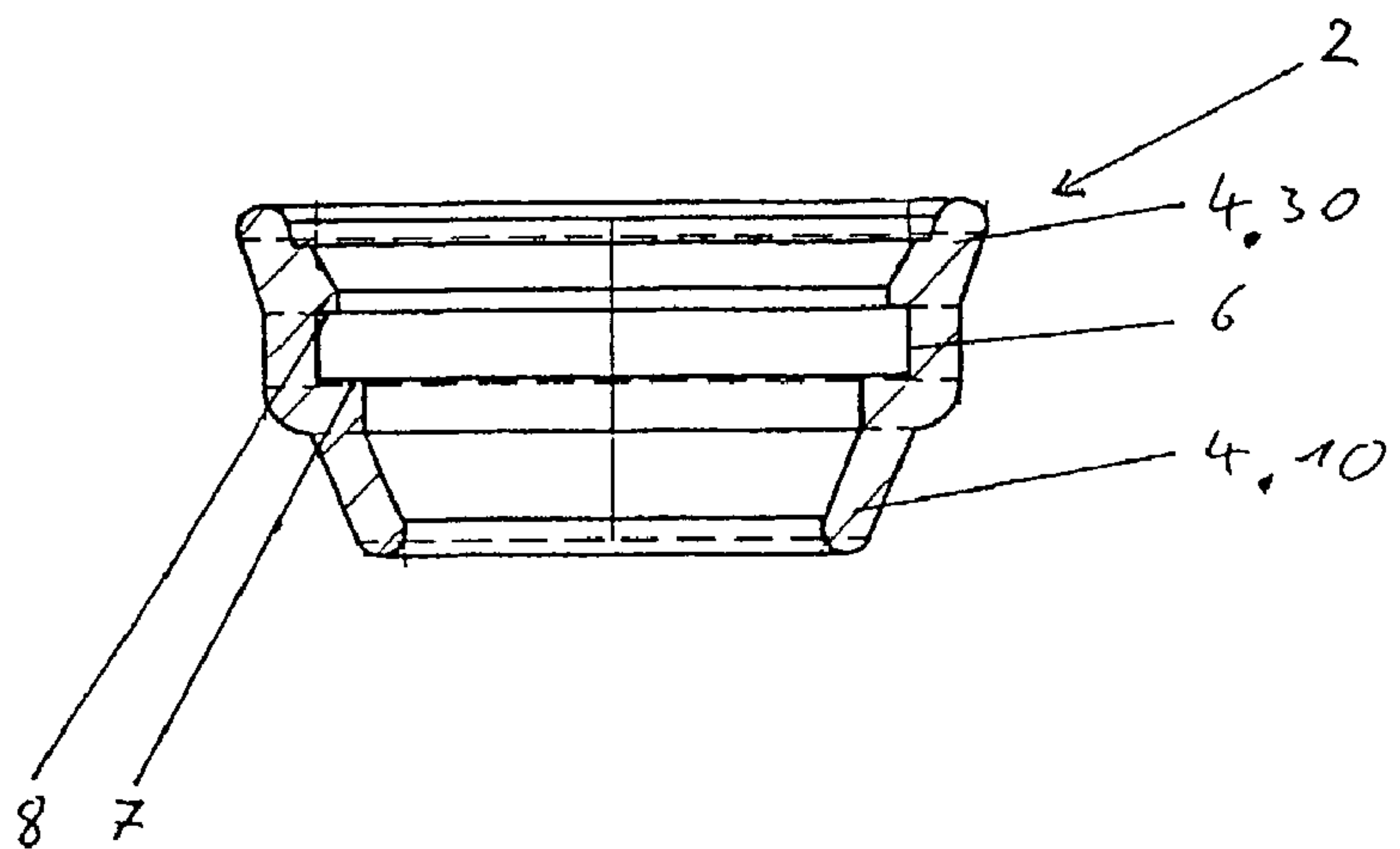
Schnitt A-A
