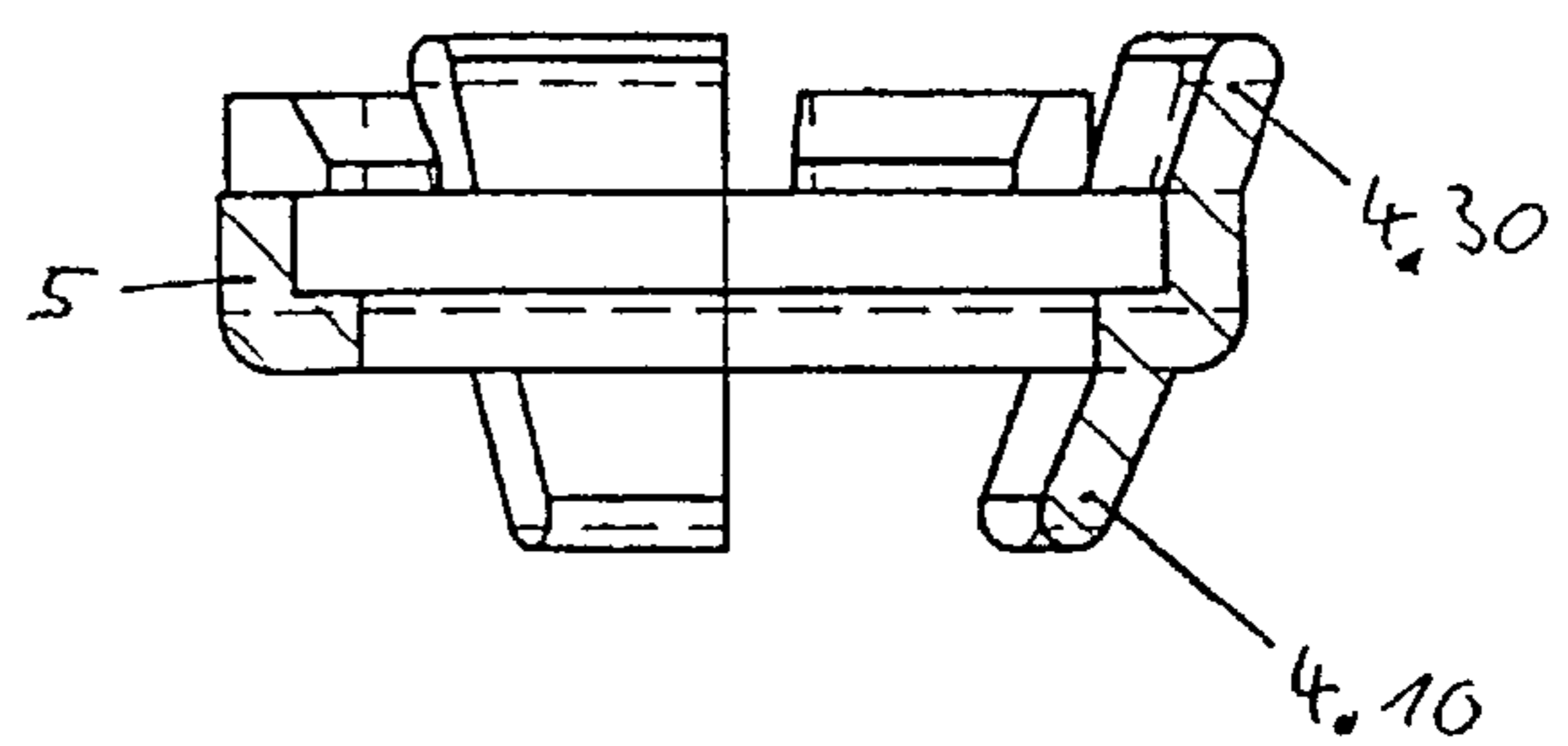
Schnitt C-C
