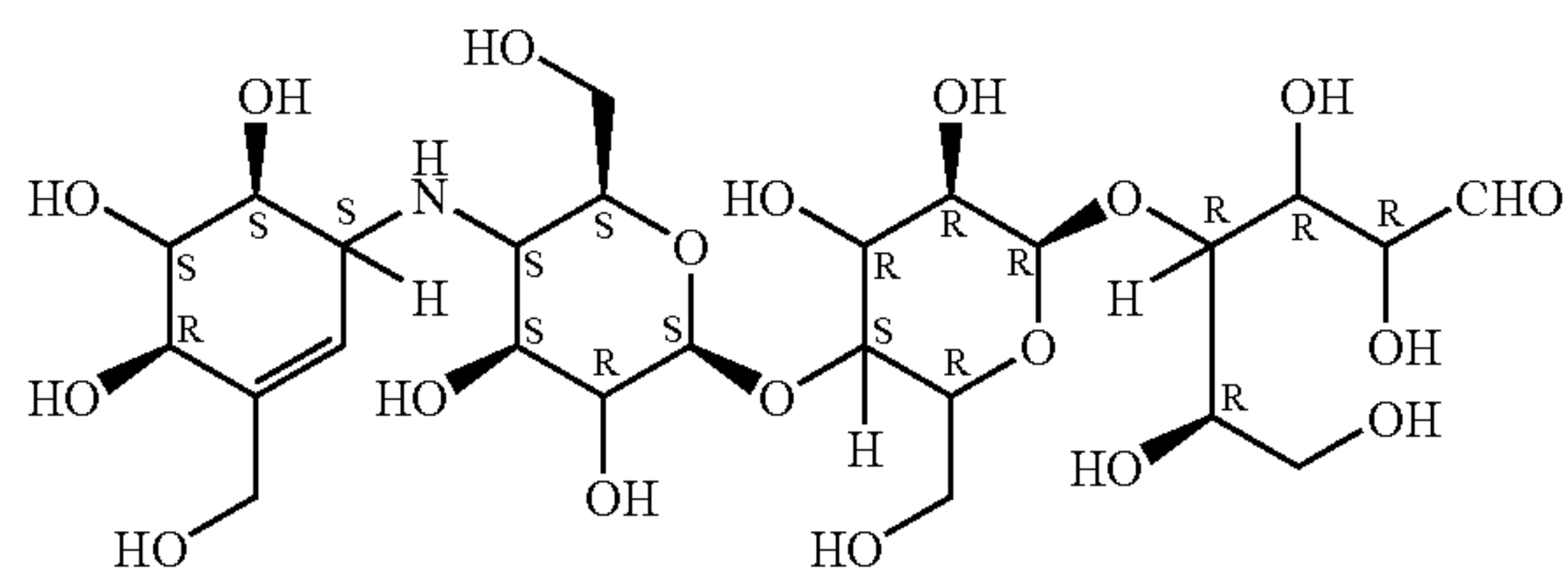
adiposin-2
