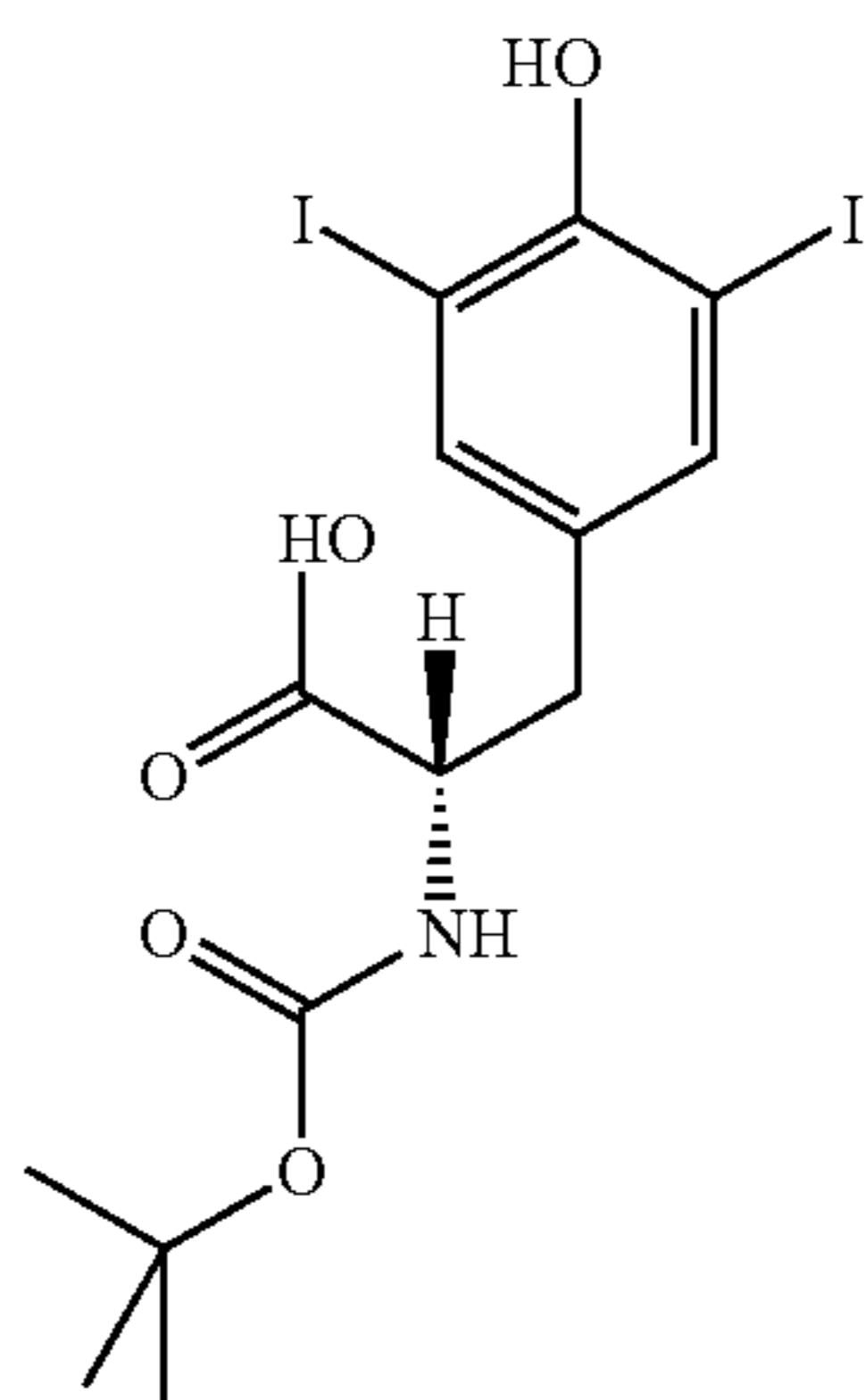
N-tert-butylloxycarbonyl-3,5-diiodo-L-tyrosine
