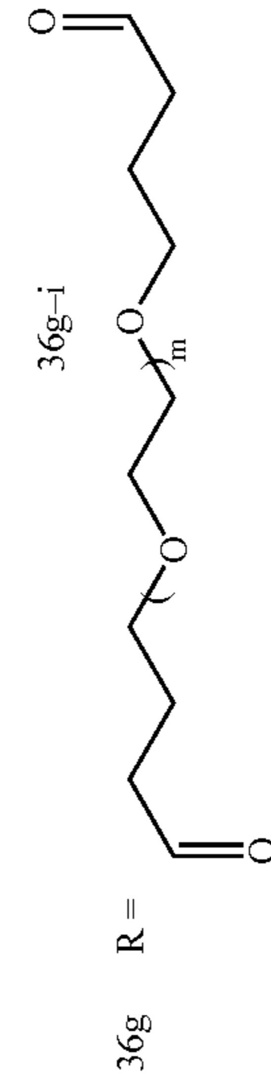
Poly(CDDCys-BA-PEG)
