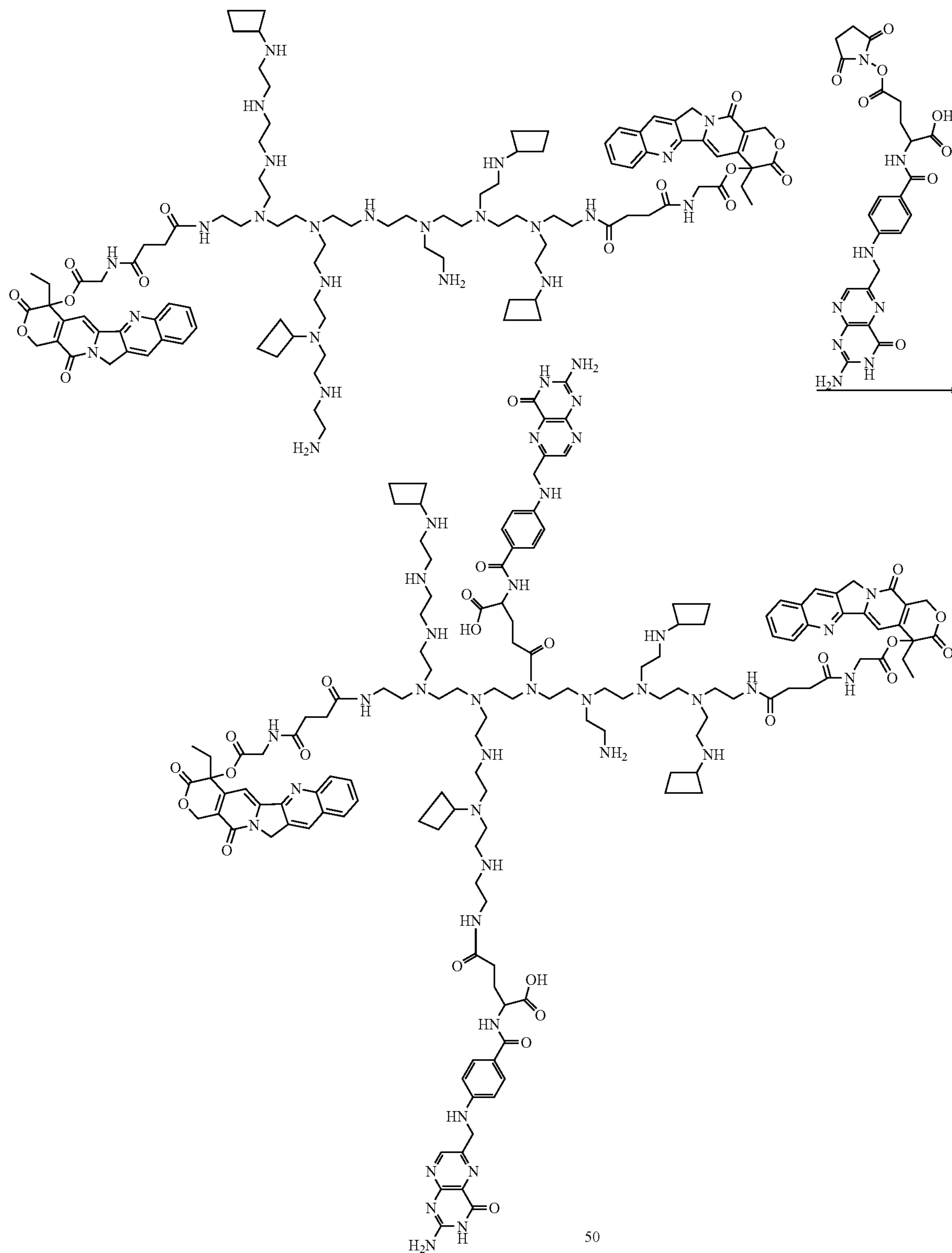
Scheme LI
