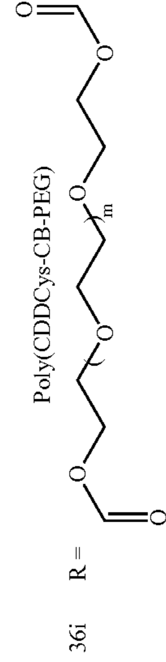
Poly(CDDCys-CB-PEG)
