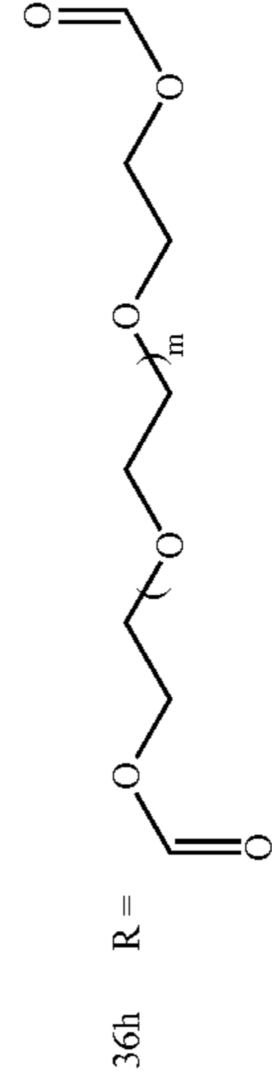
Poly(CDDCys-BA-PEG)
