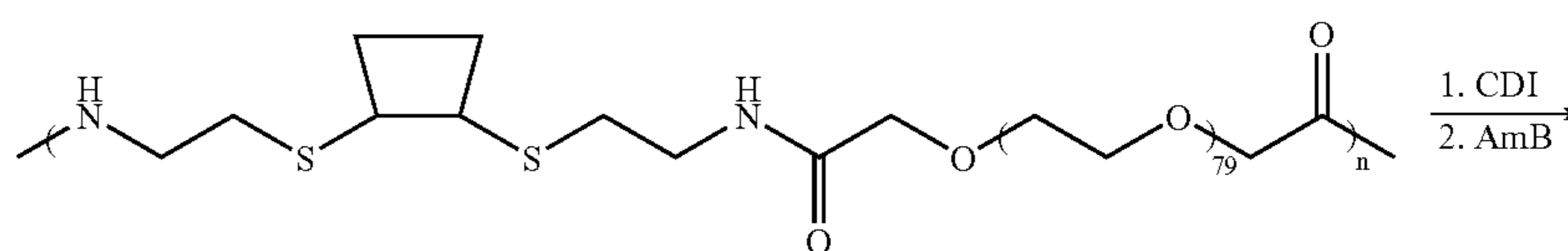
Scheme LII
