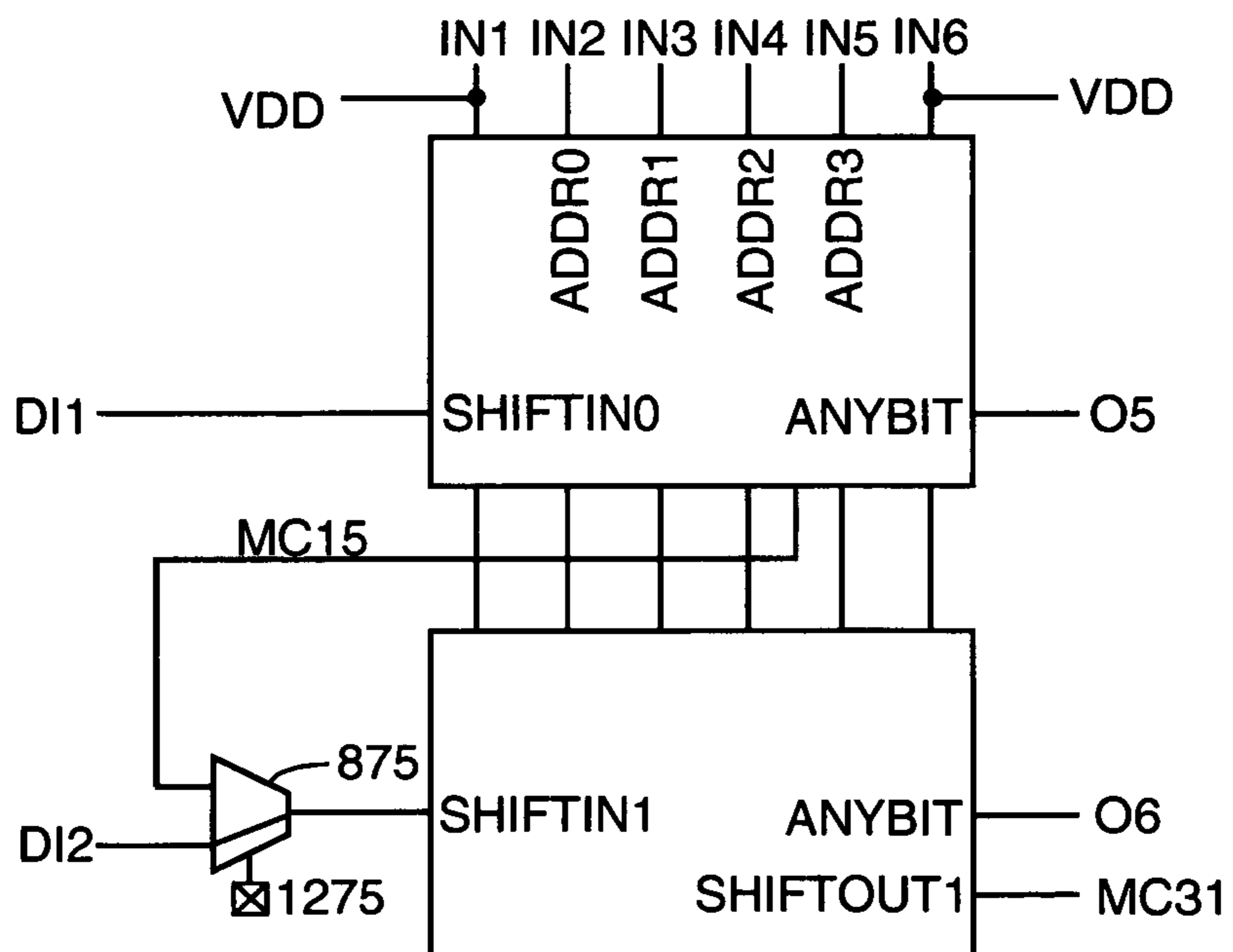
FIG. 13 (16x2 SRL)
