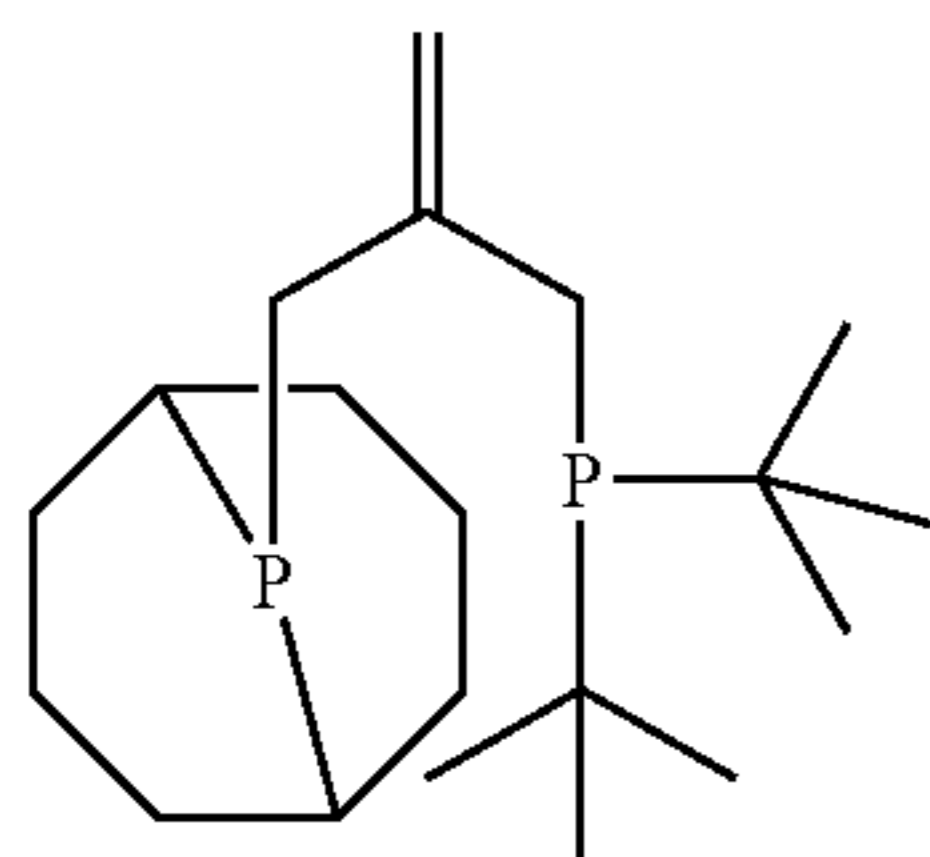
FIG. 1: 9-(2-[[di(tert-butyl)phosphino]methyl]-2-propenyl)-9-phosphabicyclo[3.3.1]nonane
