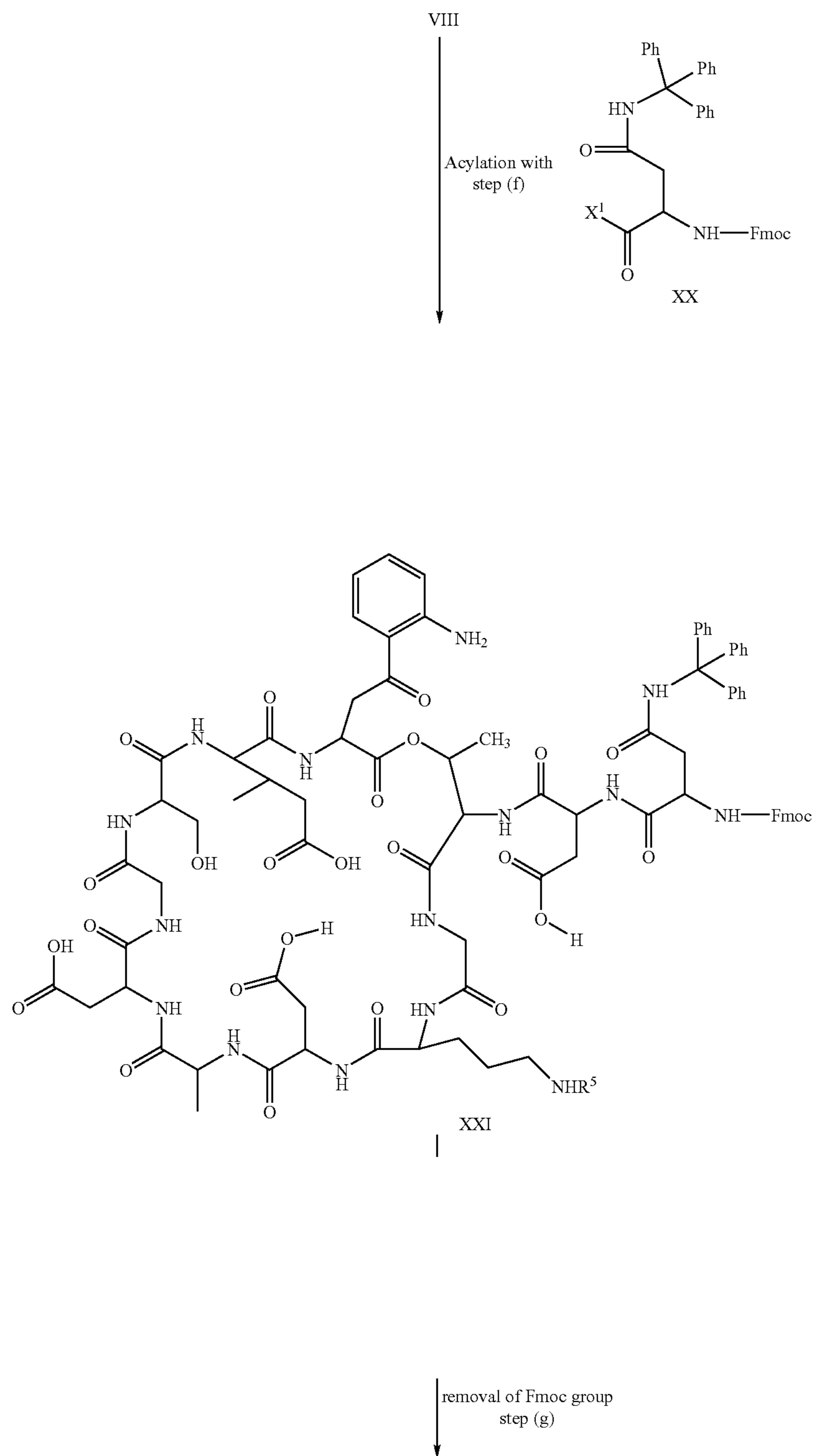
Scheme VI
