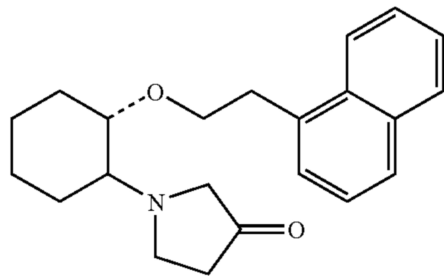
(1R,2R)/(1S,2S)-2-(3-ketopyrrolidinyl)-1-(1-naphthenethoxy)cyclohexane
