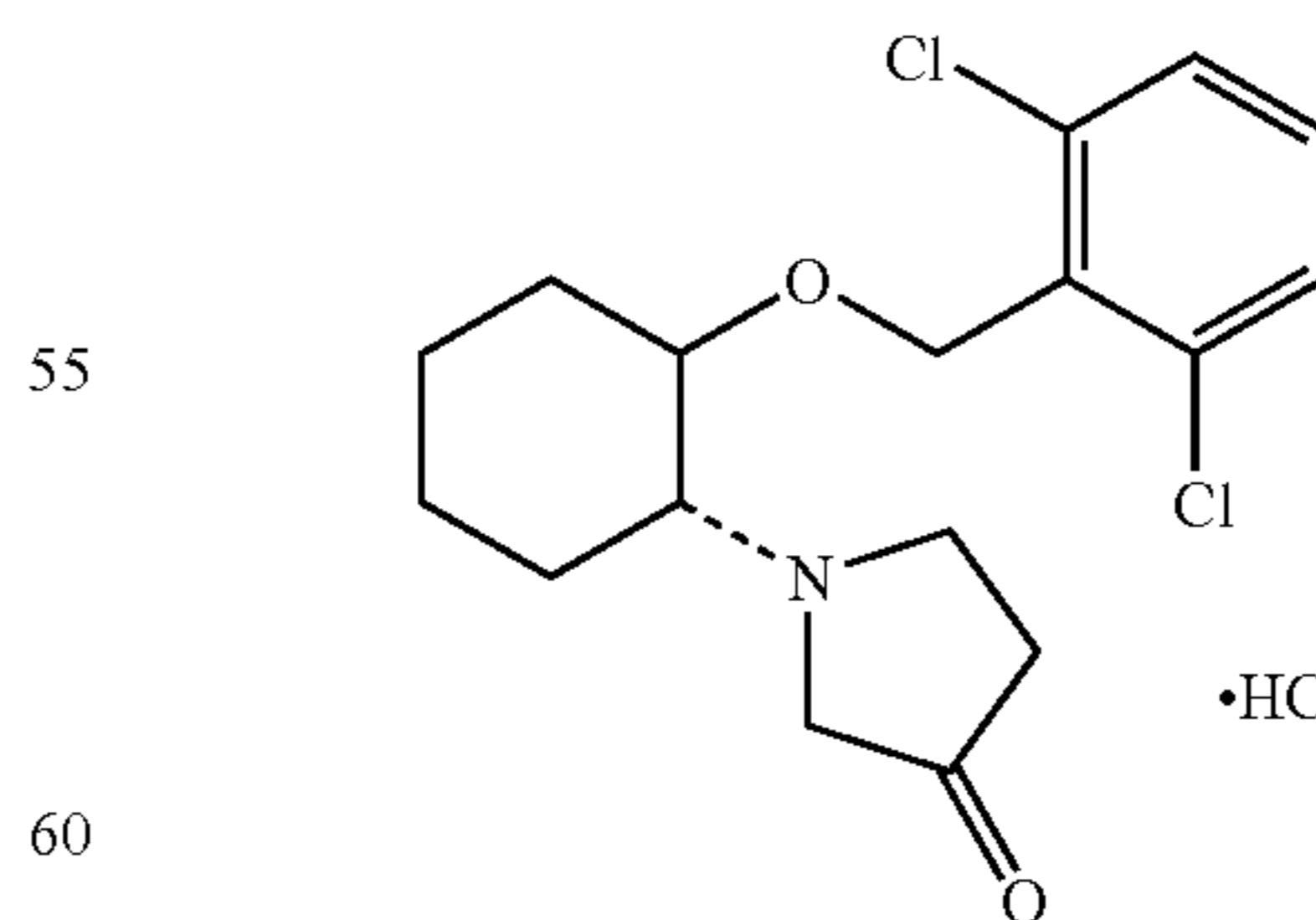
(1R,2R)/(1S,2S)-2-(3-ketopyrrolidinyl)-1-[(2,6-dichlorophenyl)methoxy]cyclohexane monohydrochloride
