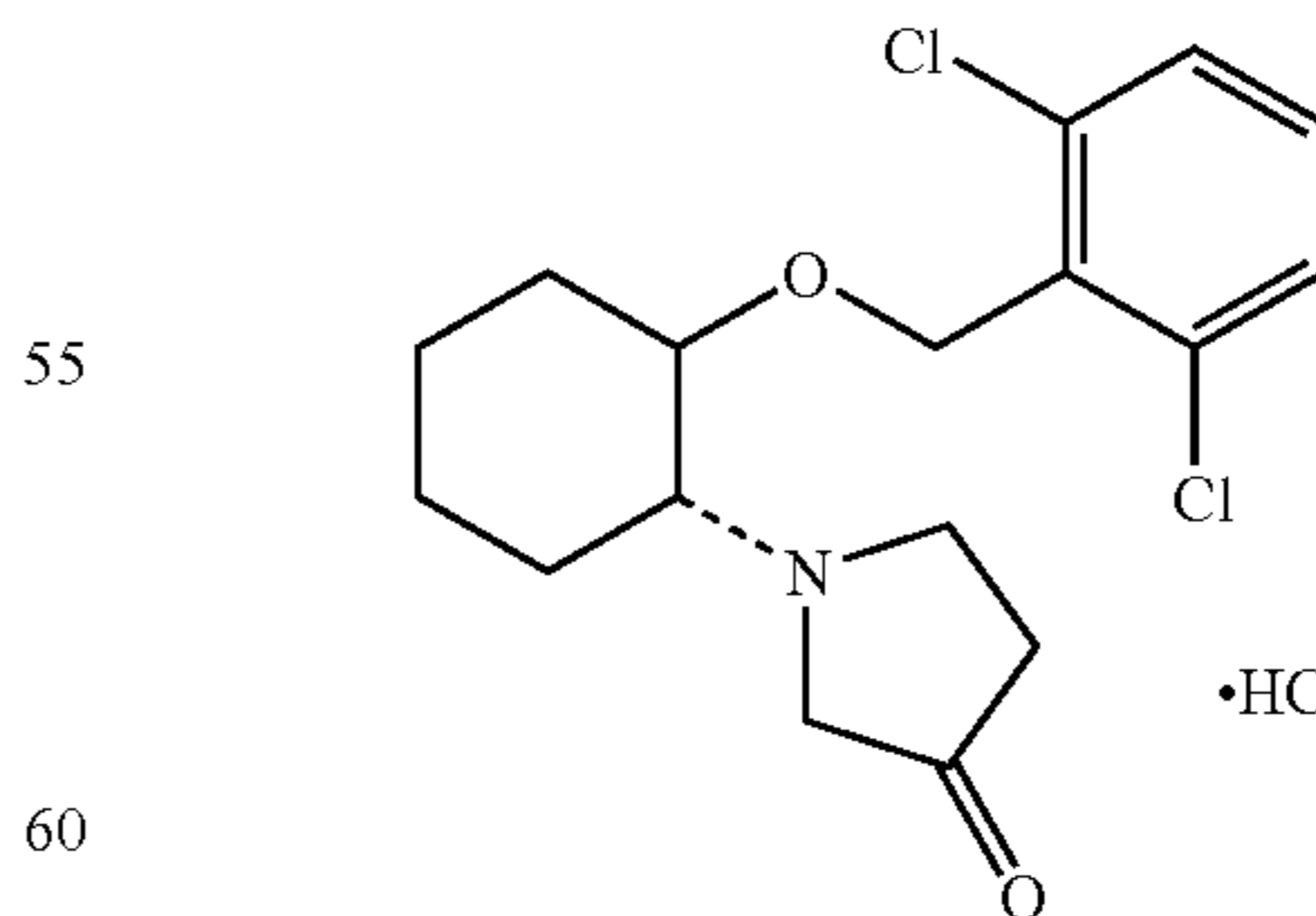
(1R,2R)/(1S,2S)-2-(3-ketopyrrolidinyl)-1-[(2,6-dichlorophenyl)methoxy]cyclohexane monohydrochloride
