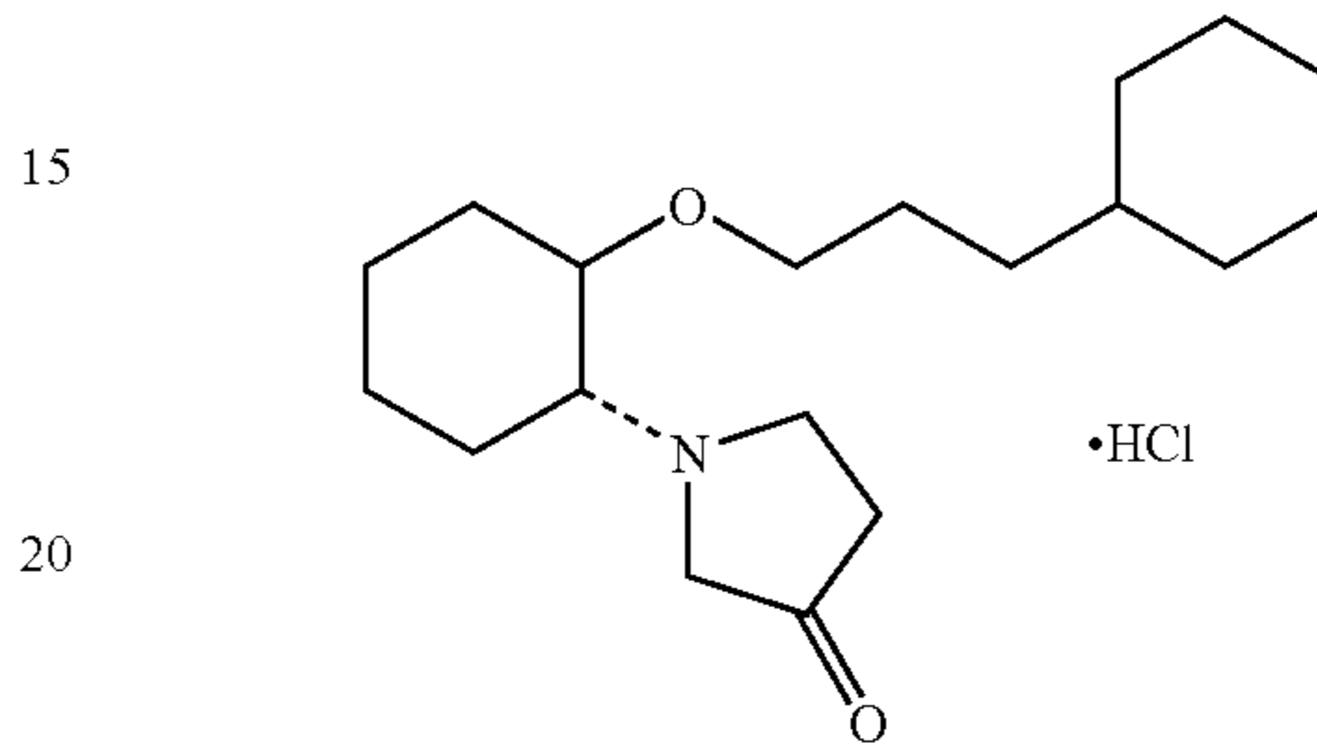
(1R,2R)/(1S,2S)-2-(3-ketopyrrolidinyl)-1-[3-(cyclohexyl)propoxy]cyclohexane monohydrochloride
