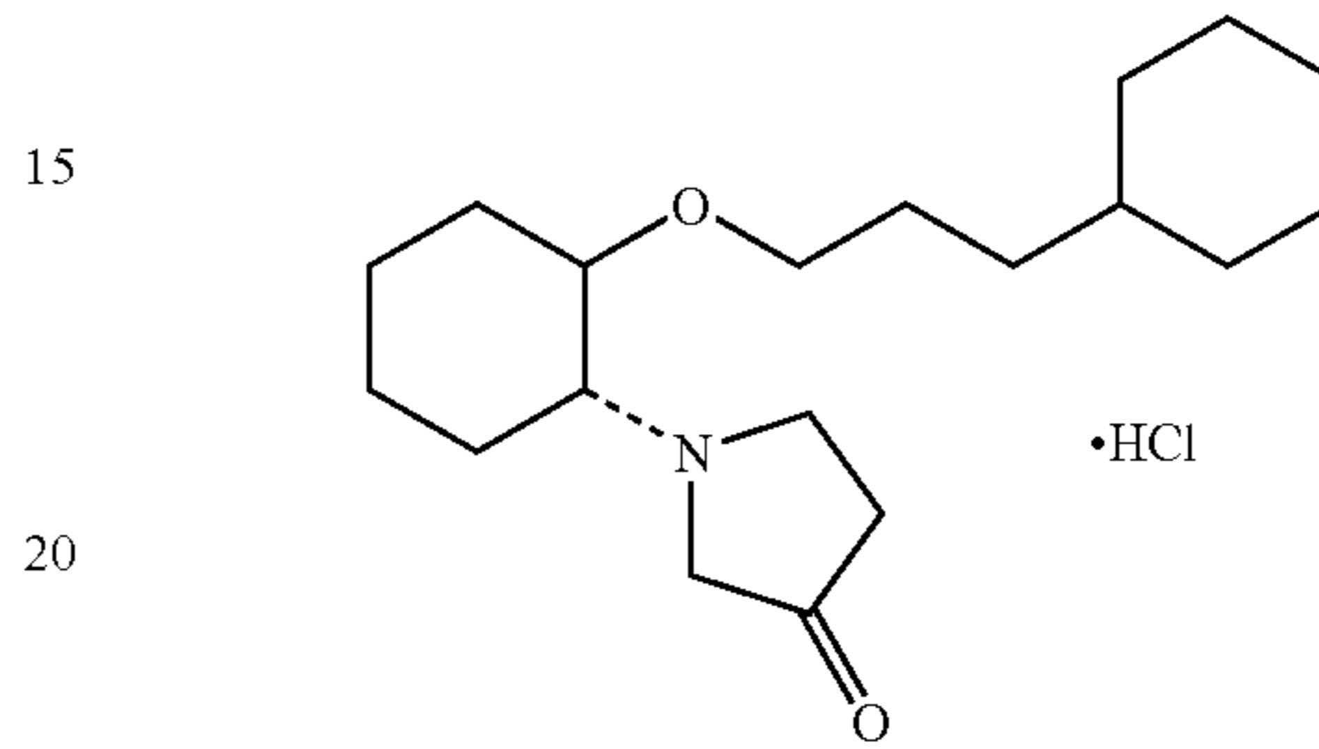
(1R,2R)/(1S,2S)-2-(3-ketopyrrolidinyl)-1-[3-(cyclohexyl)propoxy]cyclohexane monohydrochloride
