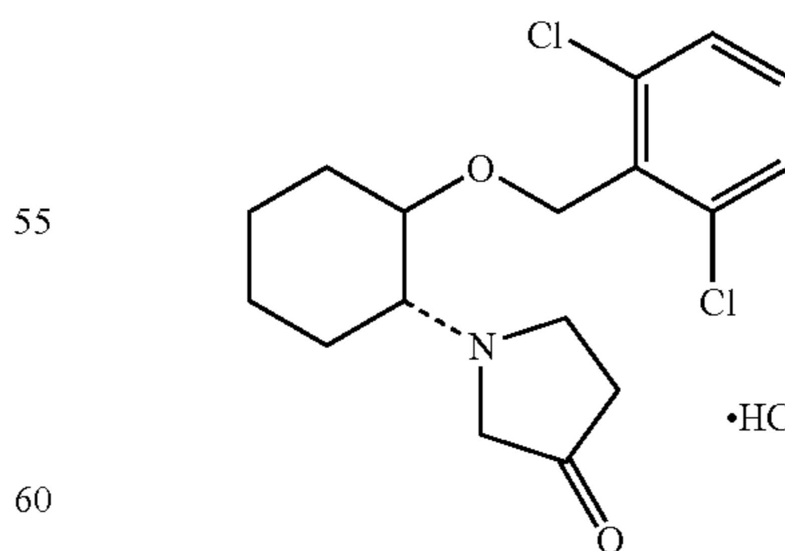
(1R,2R)/(1S,2S)-2-(3-ketopyrrolidinyl)-1-[(2,6-dichlorophenyl)methoxy]cyclohexane monohydrochloride
