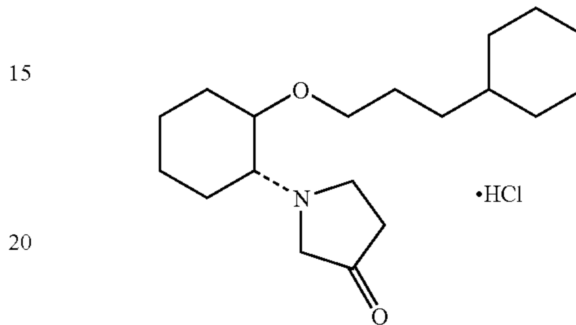
(1R,2R)/(1S,2S)-2-(3-ketopyrrolidinyl)-1-[3-(cyclohexyl)propoxy]cyclohexane monohydrochloride
