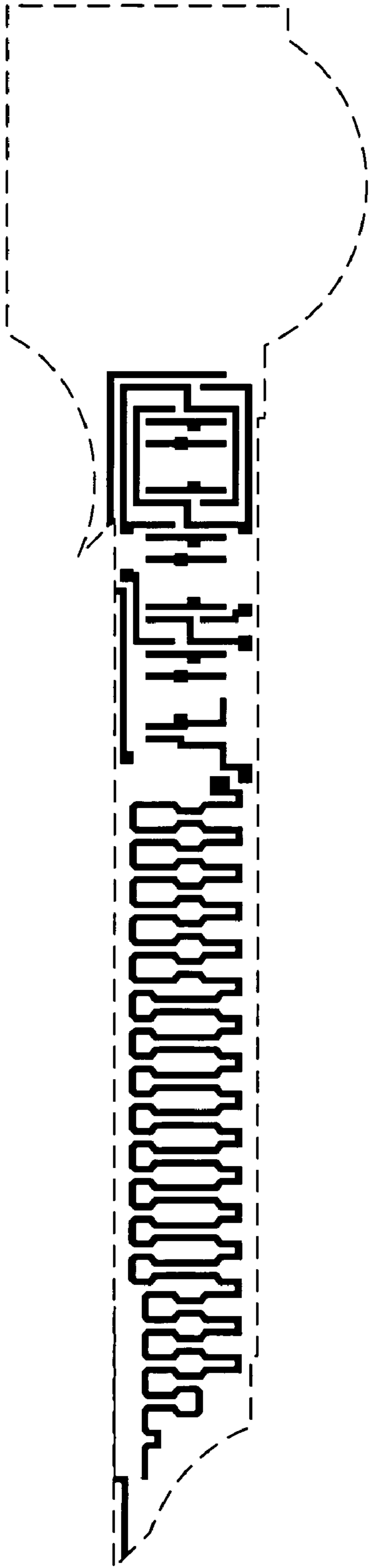
Poly mask
