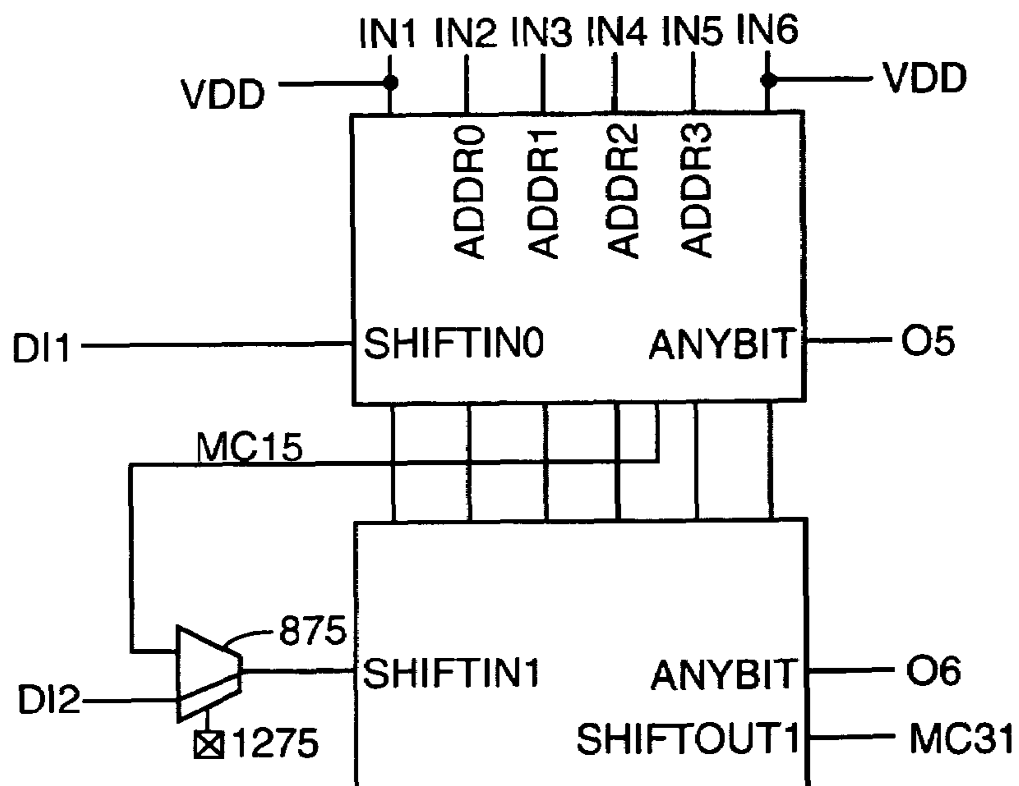
FIG. 13 (16x2 SRL)
