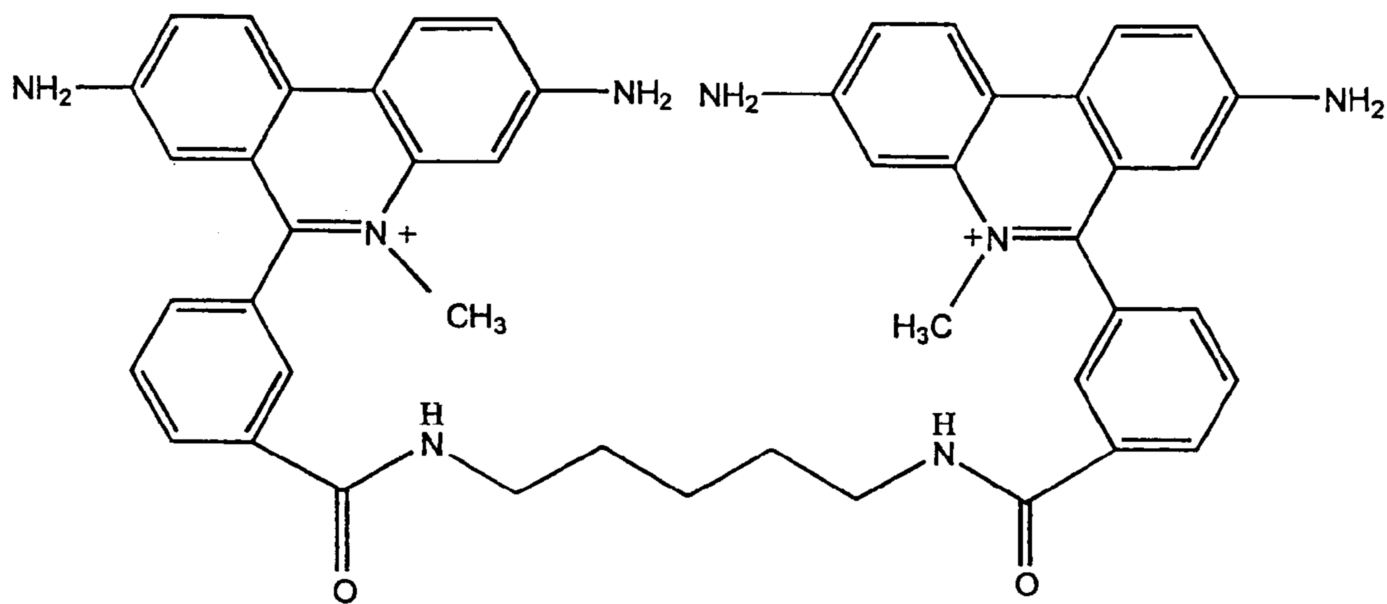
meta -EthD
