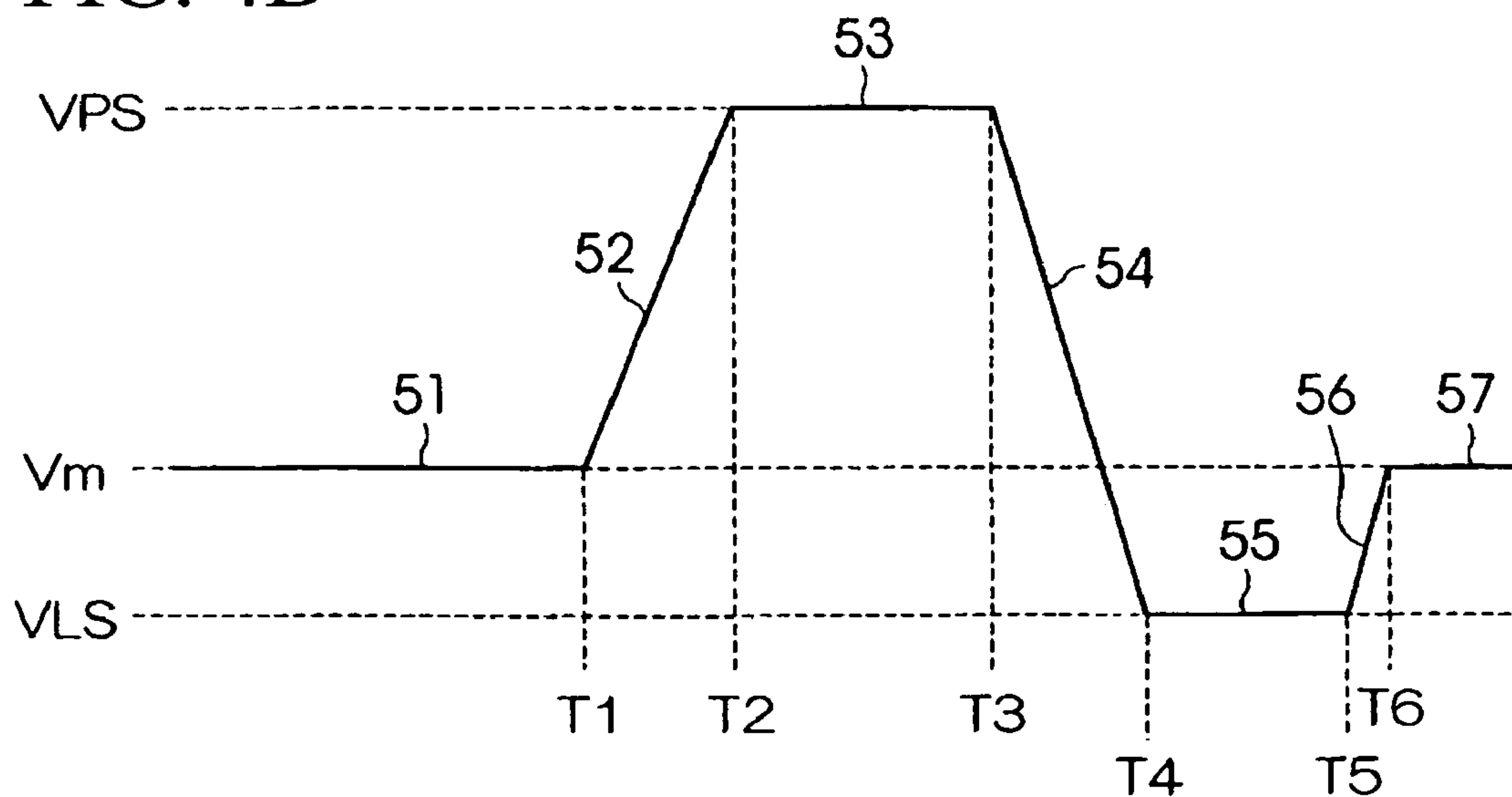
FIG. 4B
