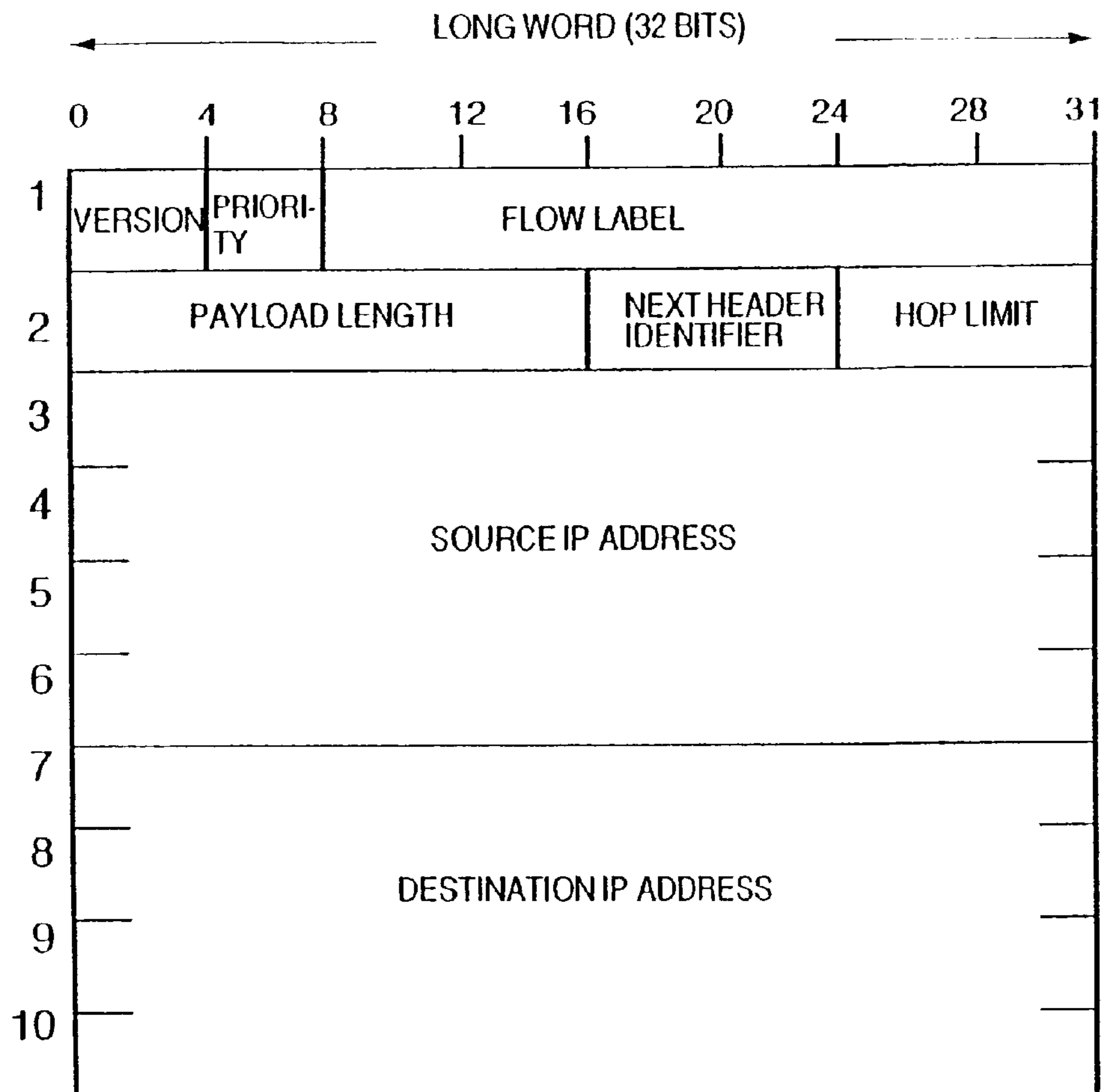
FIG. 11A IPv6 HEADER FORMAT
