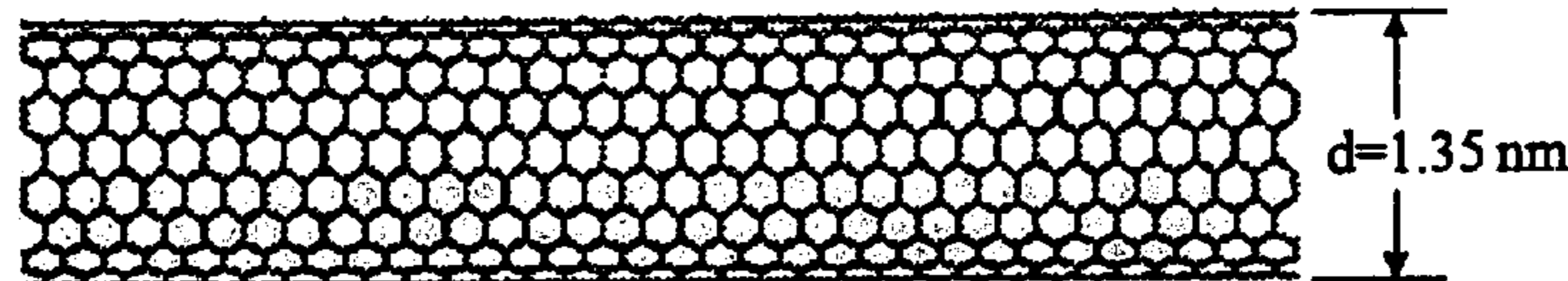
10,10 nanotube
