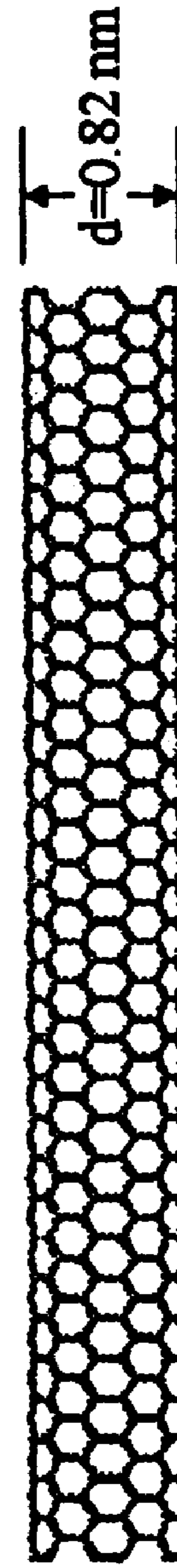
6,6 nanotube
