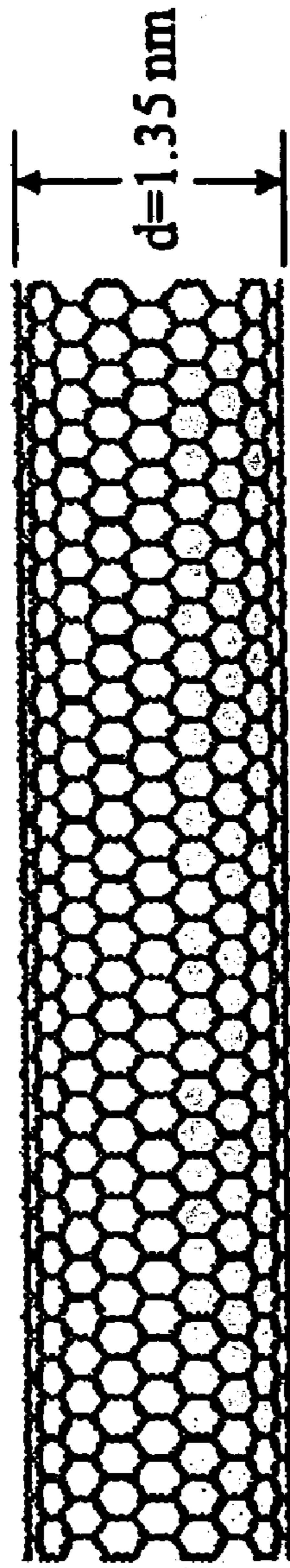
10,10 nanotube
