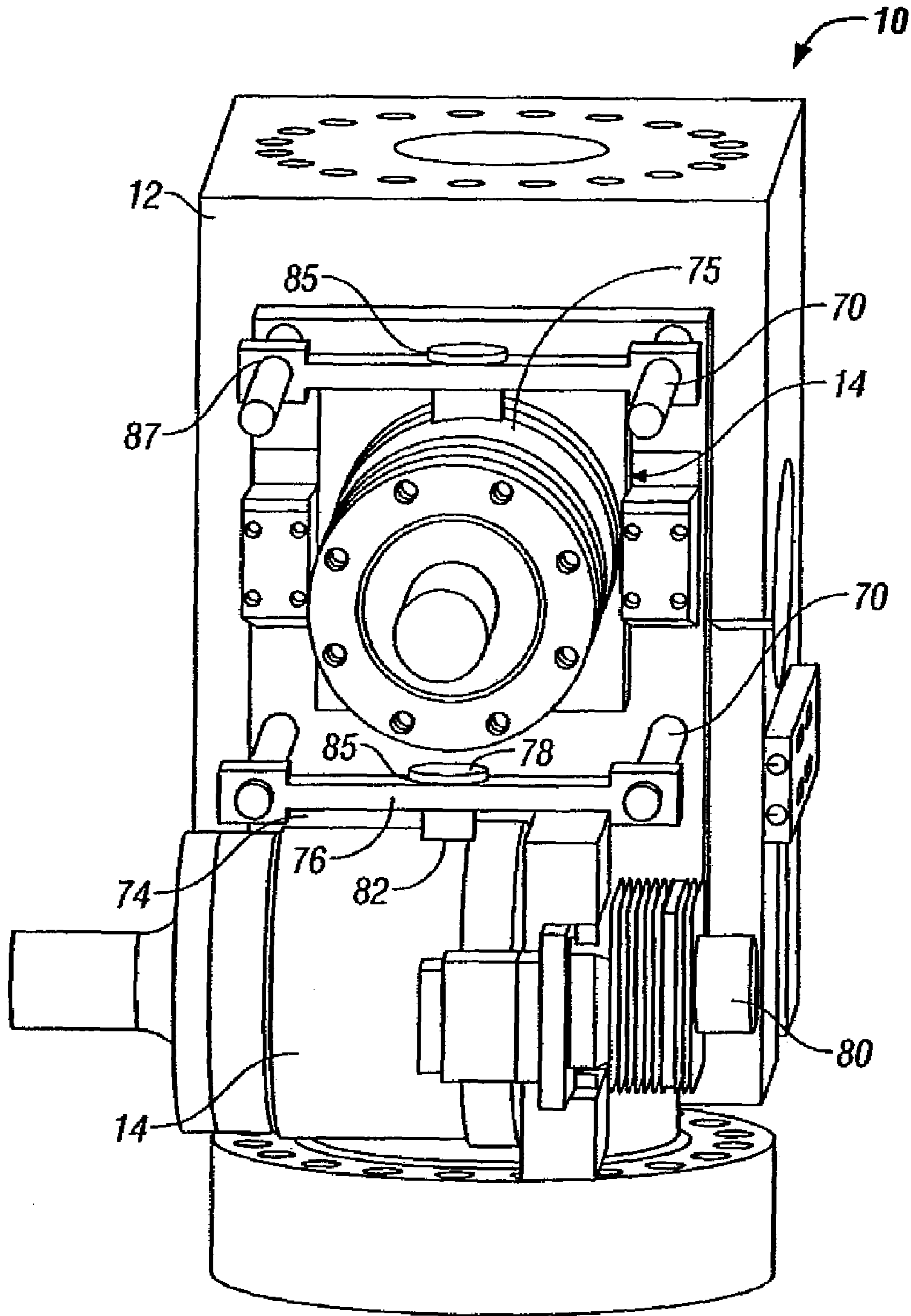
FIG. 23
