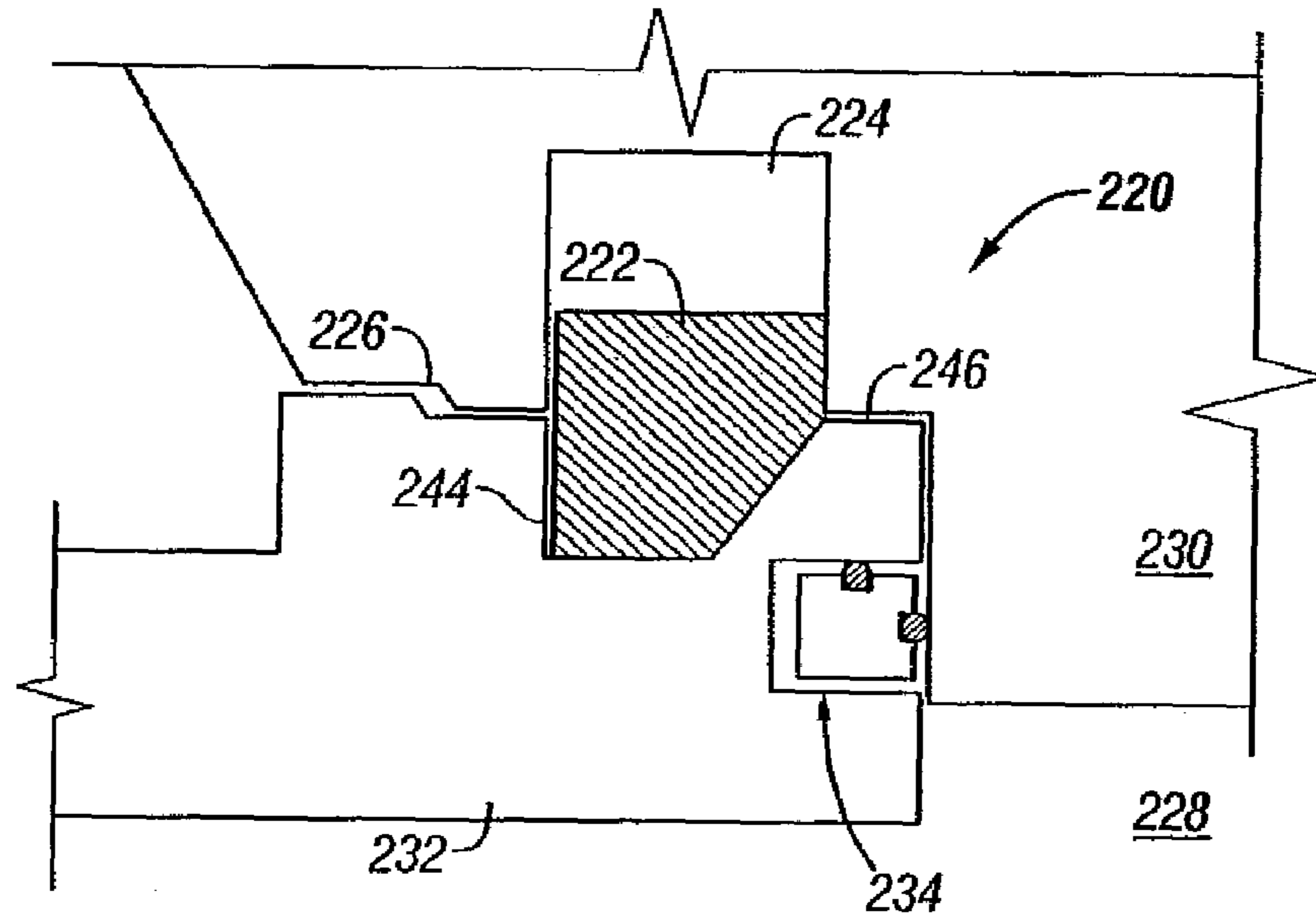
FIG. 18
