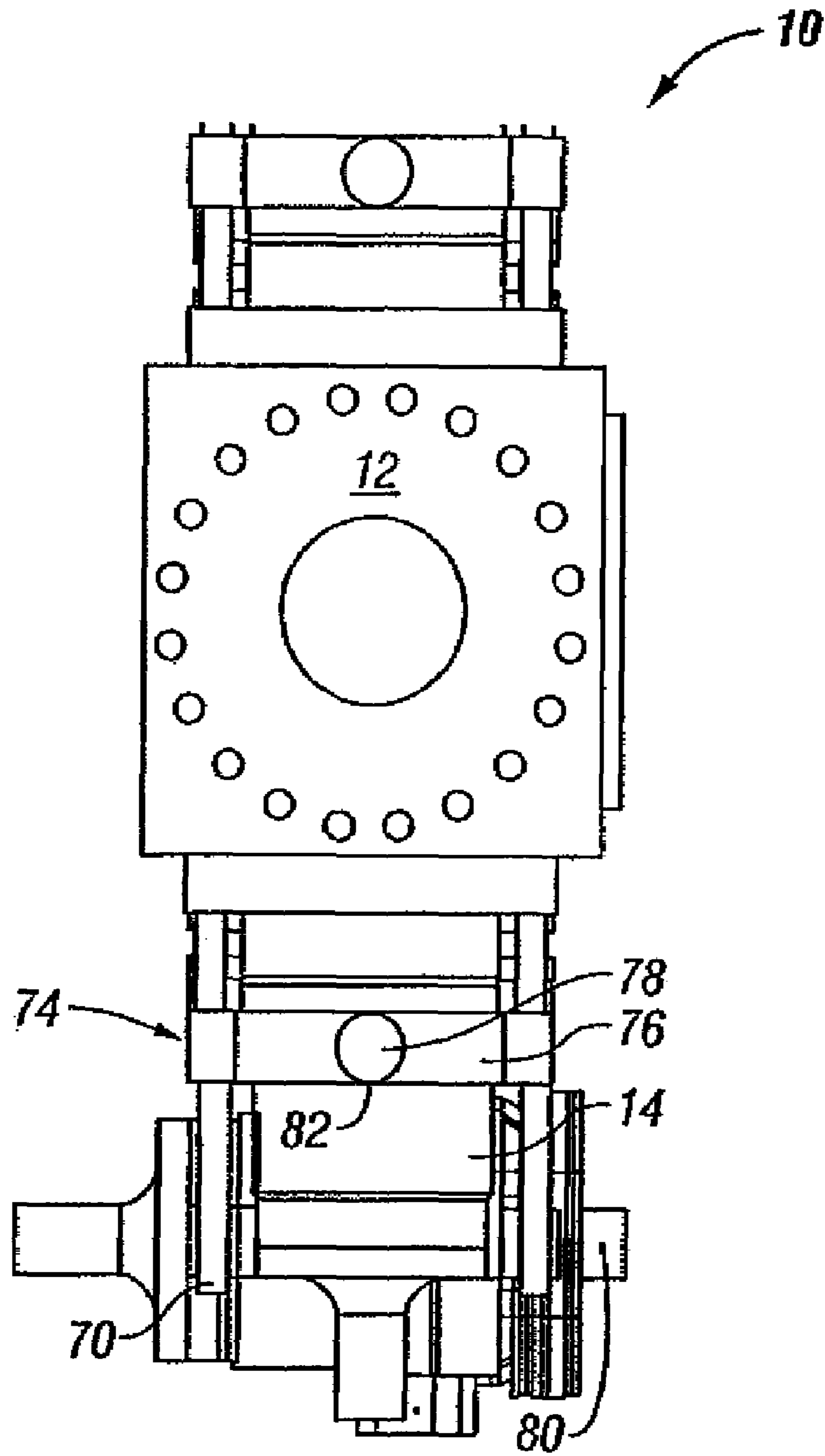
FIG. 25
