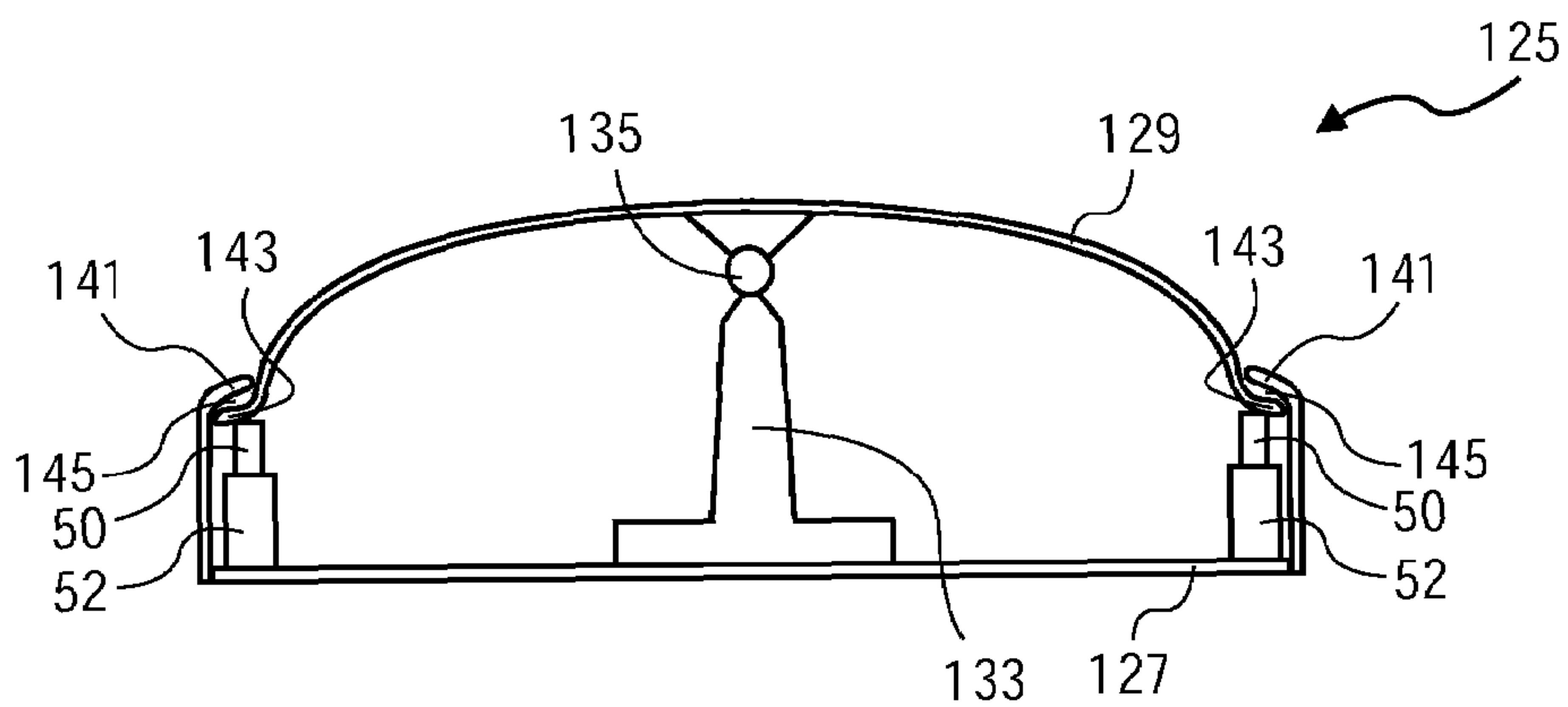
FIG. 10B
