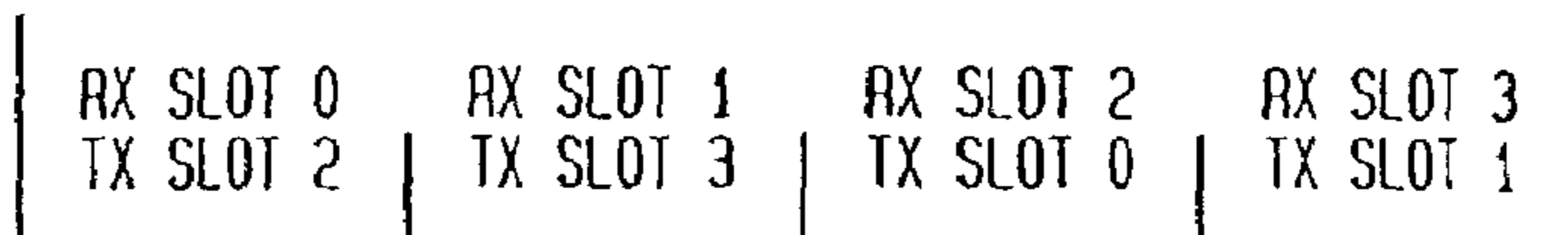
FIG. 2B (16 PSK)
