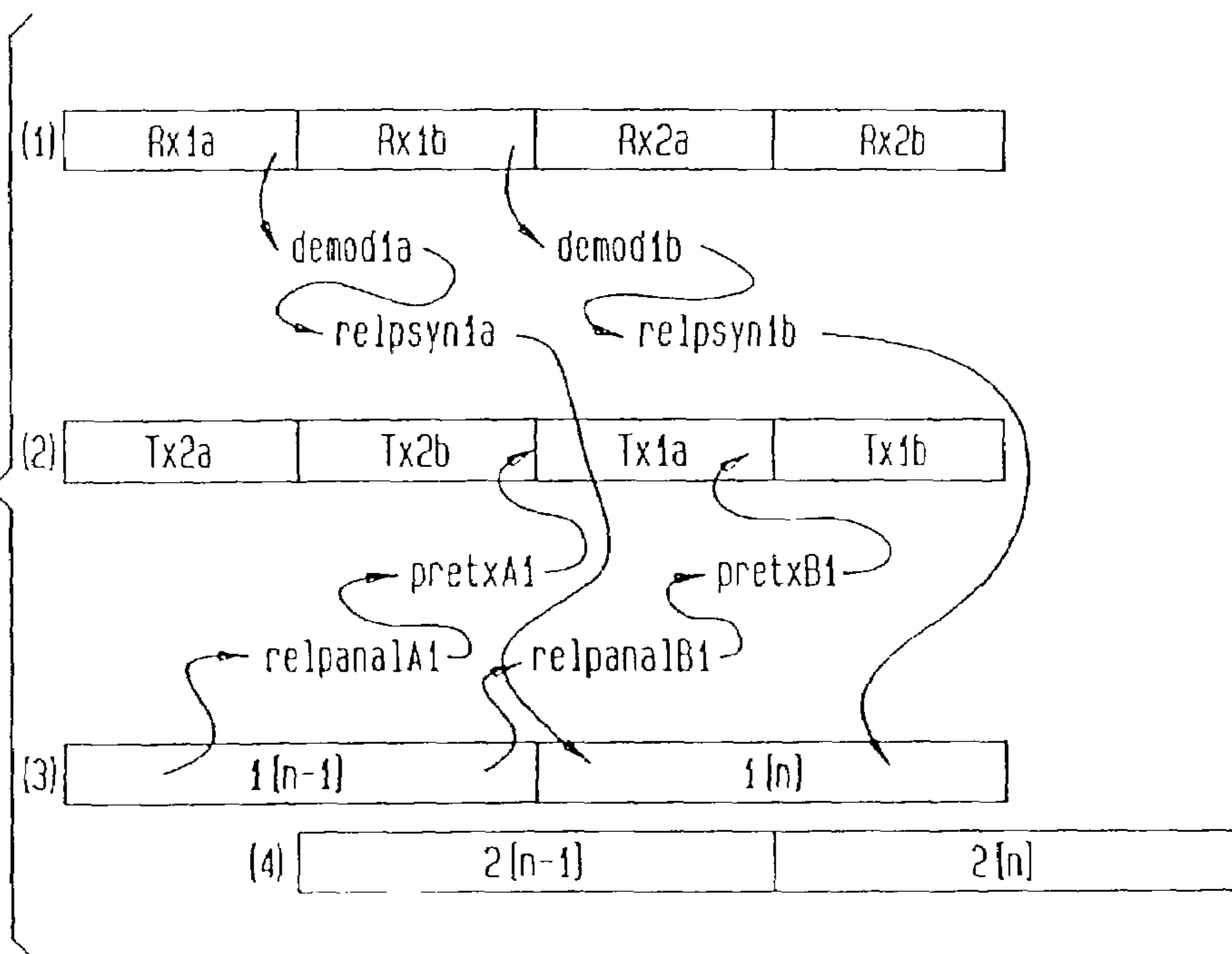
FIG. 2D (QPSK)
