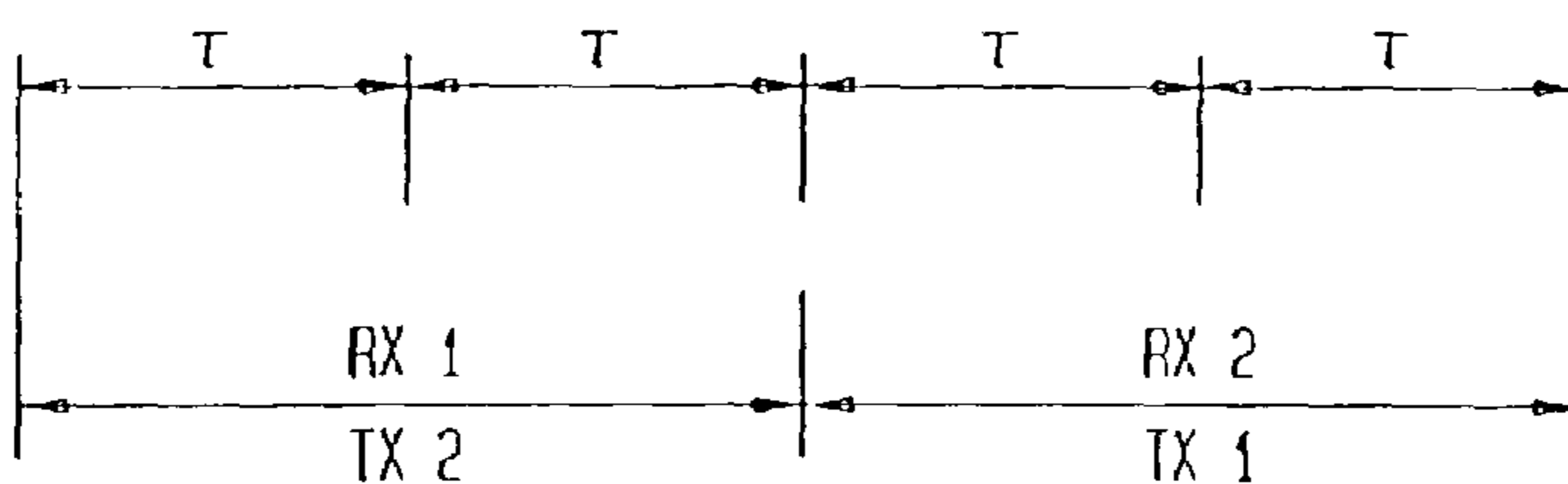
FIG. 2C (QPSK)
