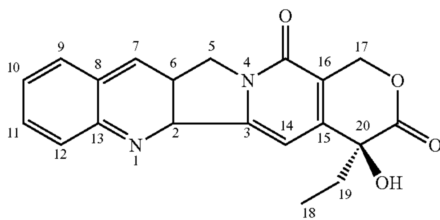
FIG. 1 - Camptothecin
