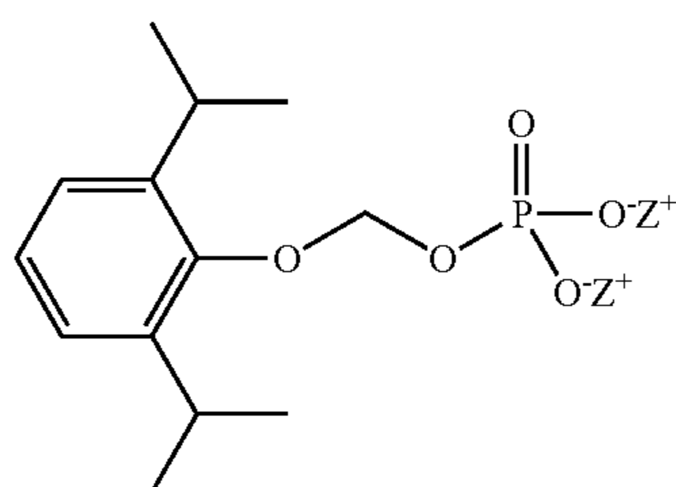
Propofol Prodrug
