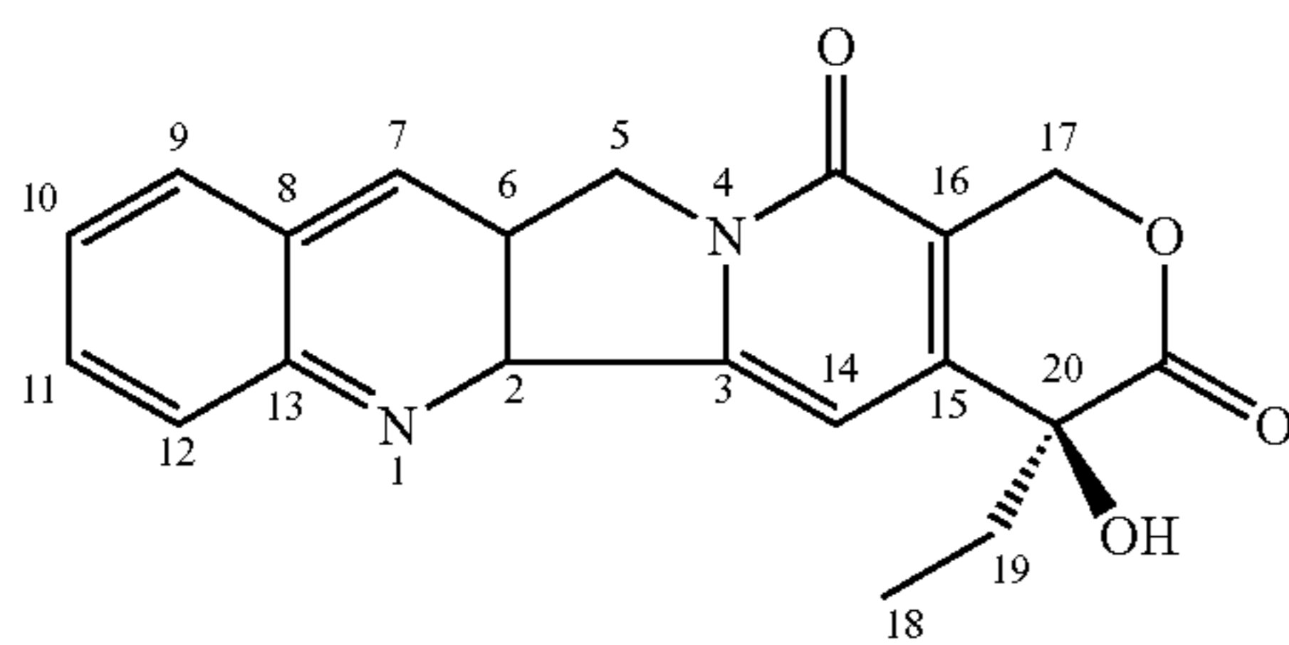
FIG. 1 - Camptothecin
