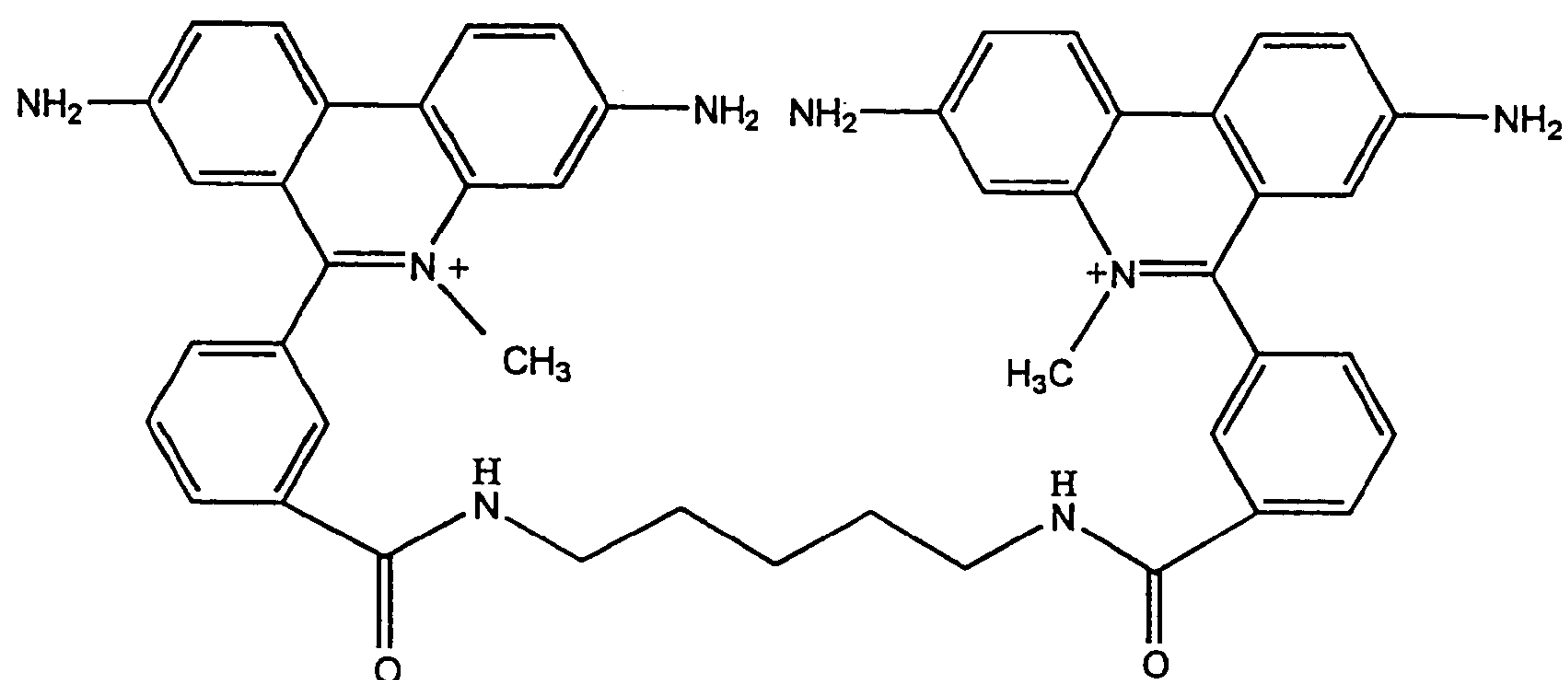
meta -EthD
