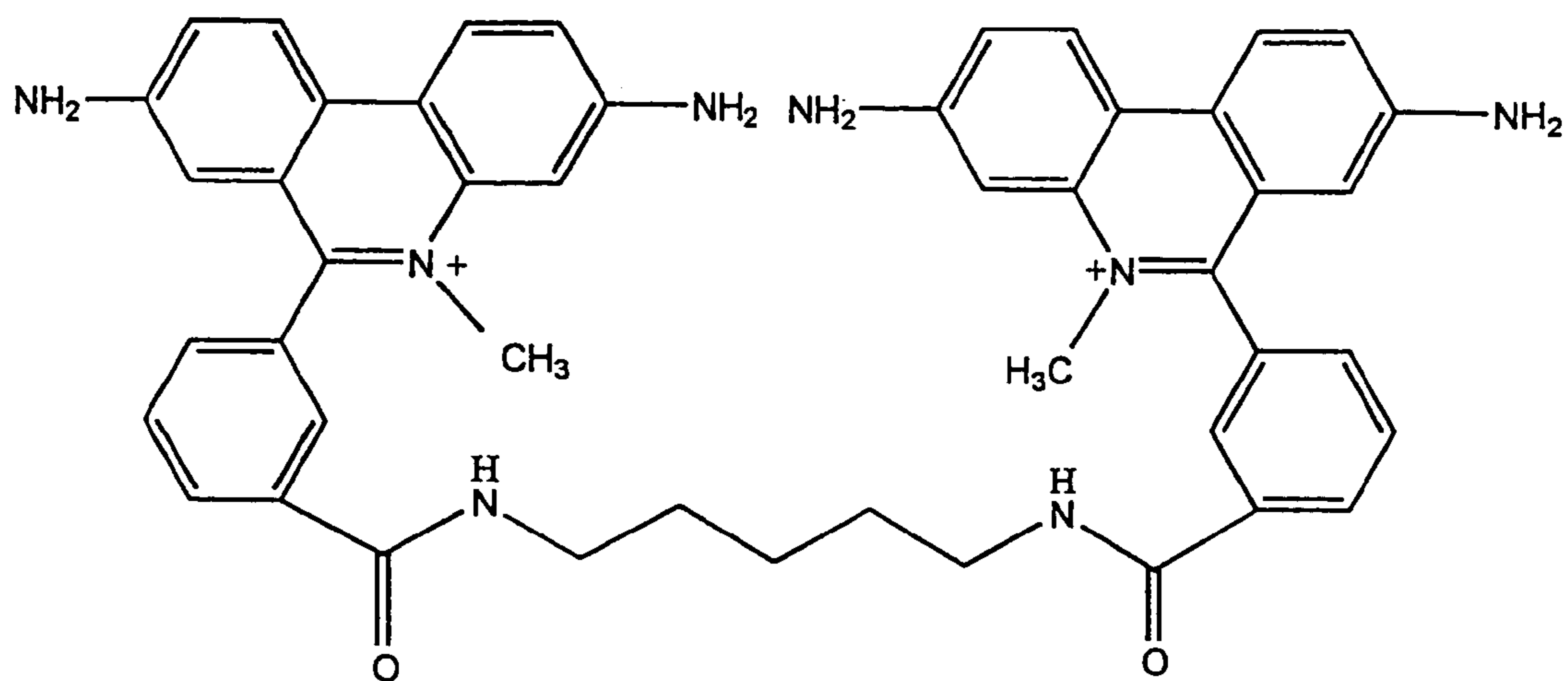
meta -EthD
