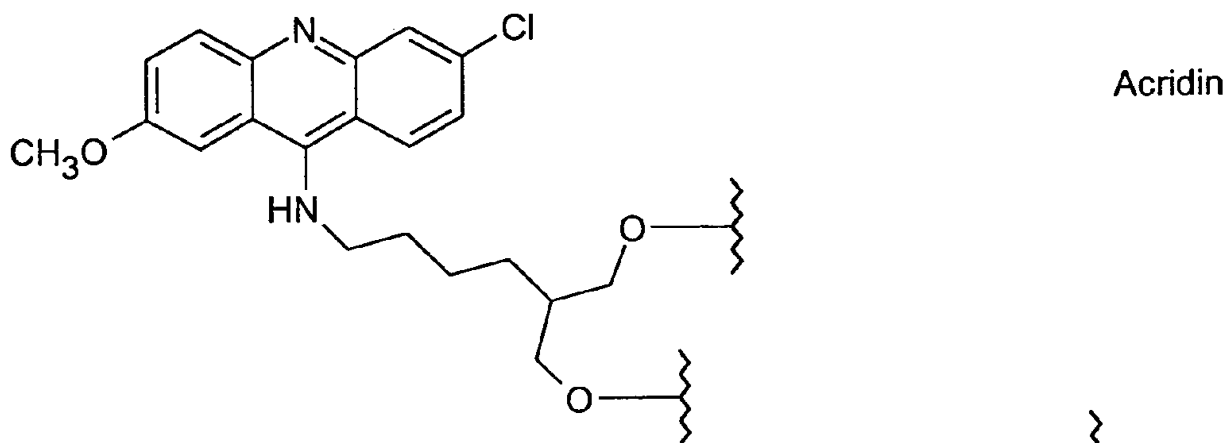
DNP
