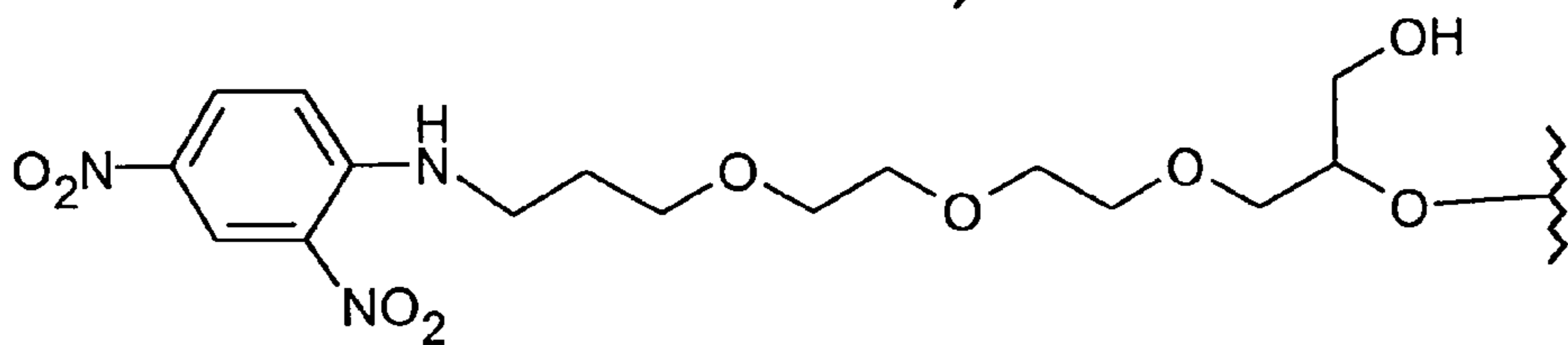
DNP
