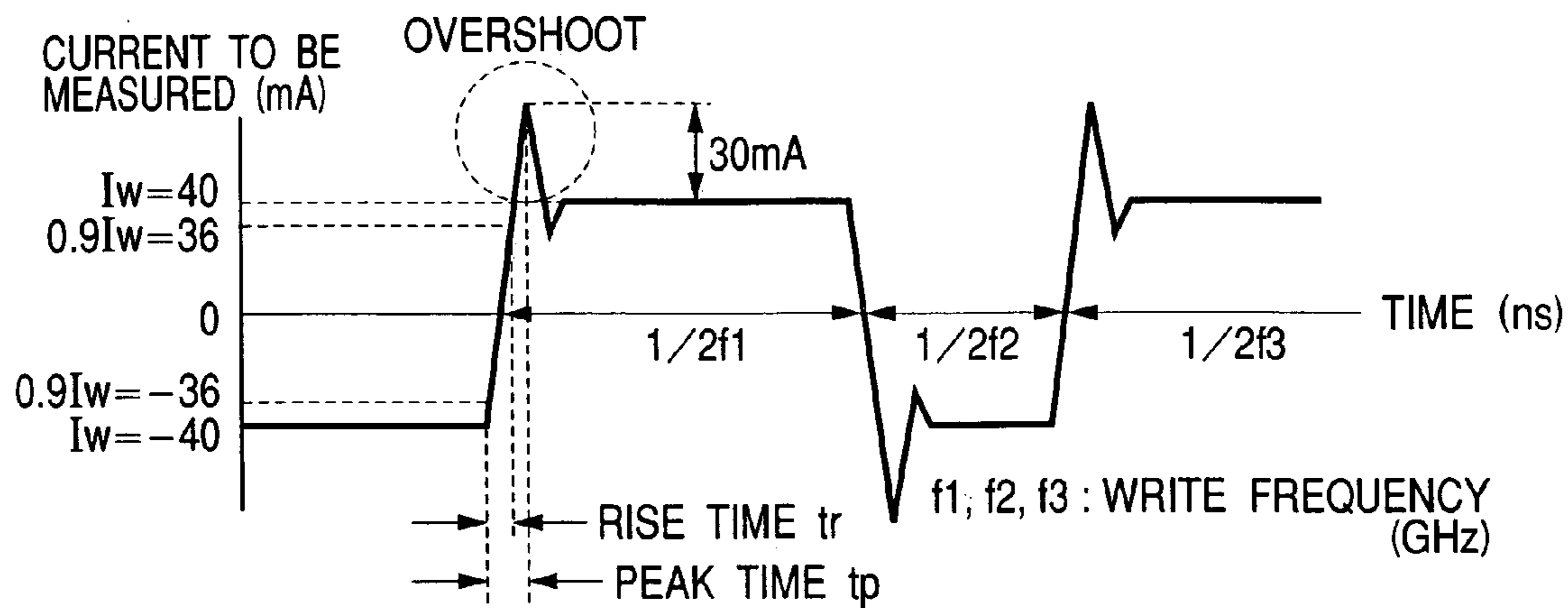
FIG. 8A
