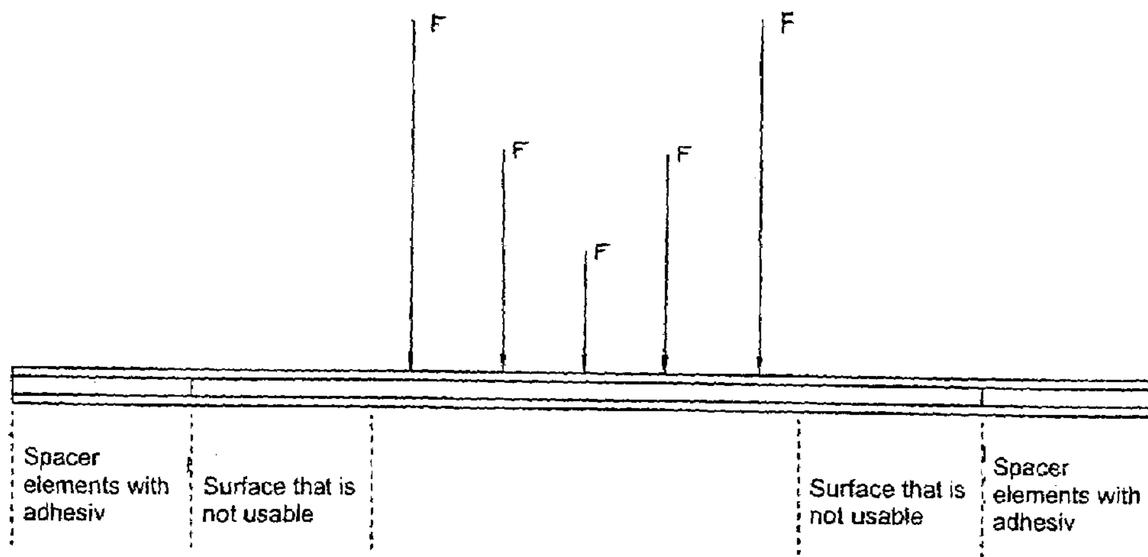
Fig 11b
