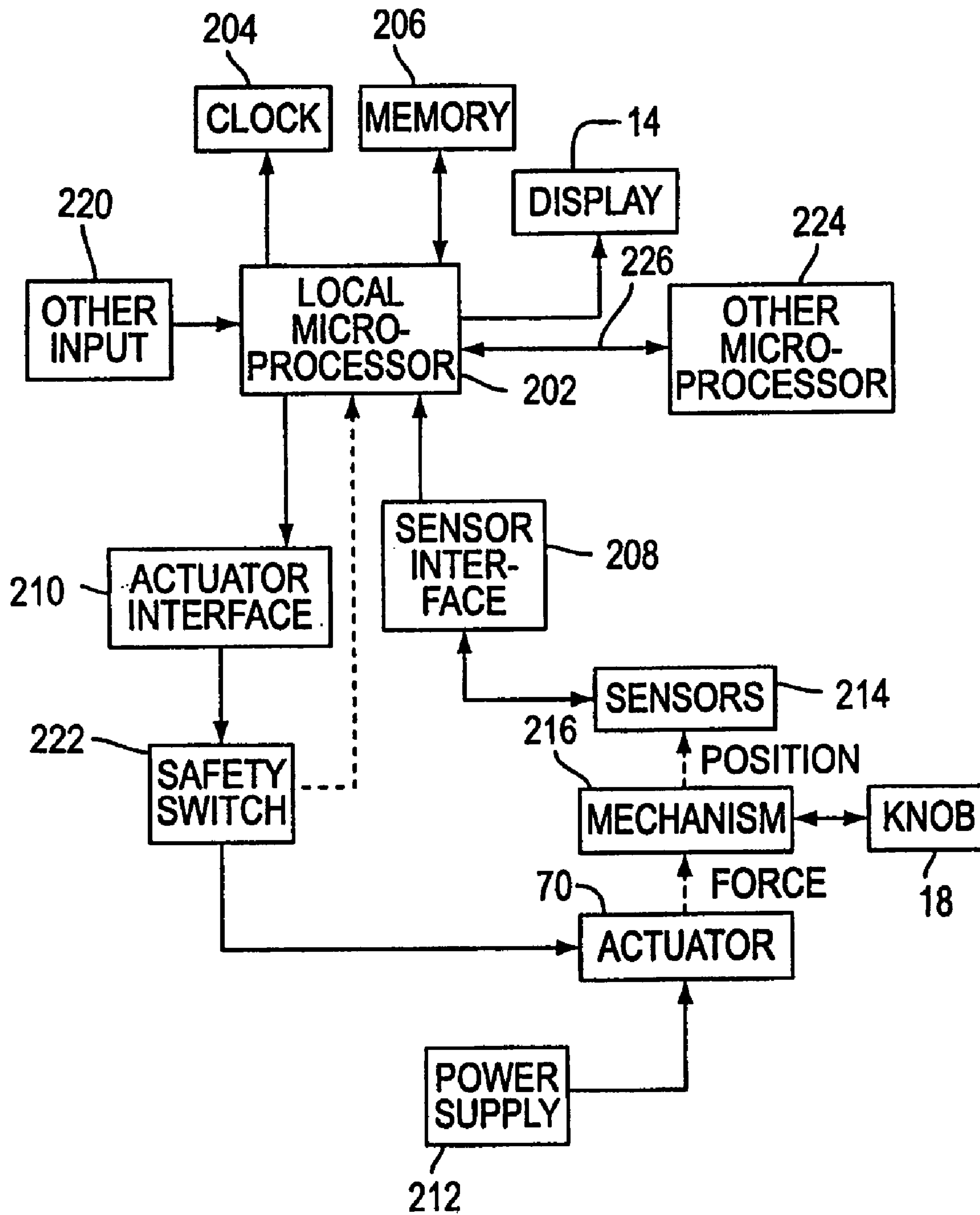
FIG. 8
