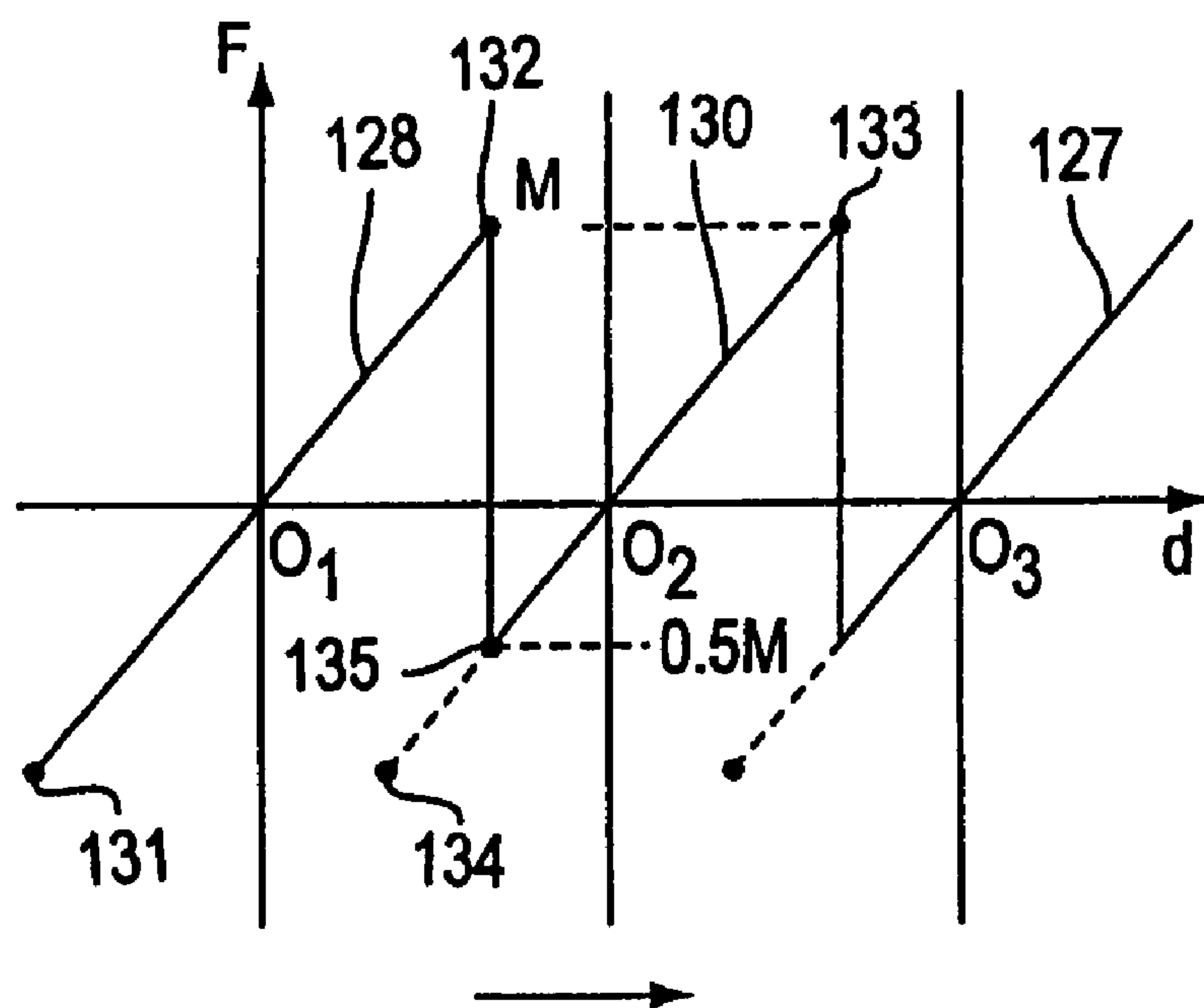
FIG. 6C
