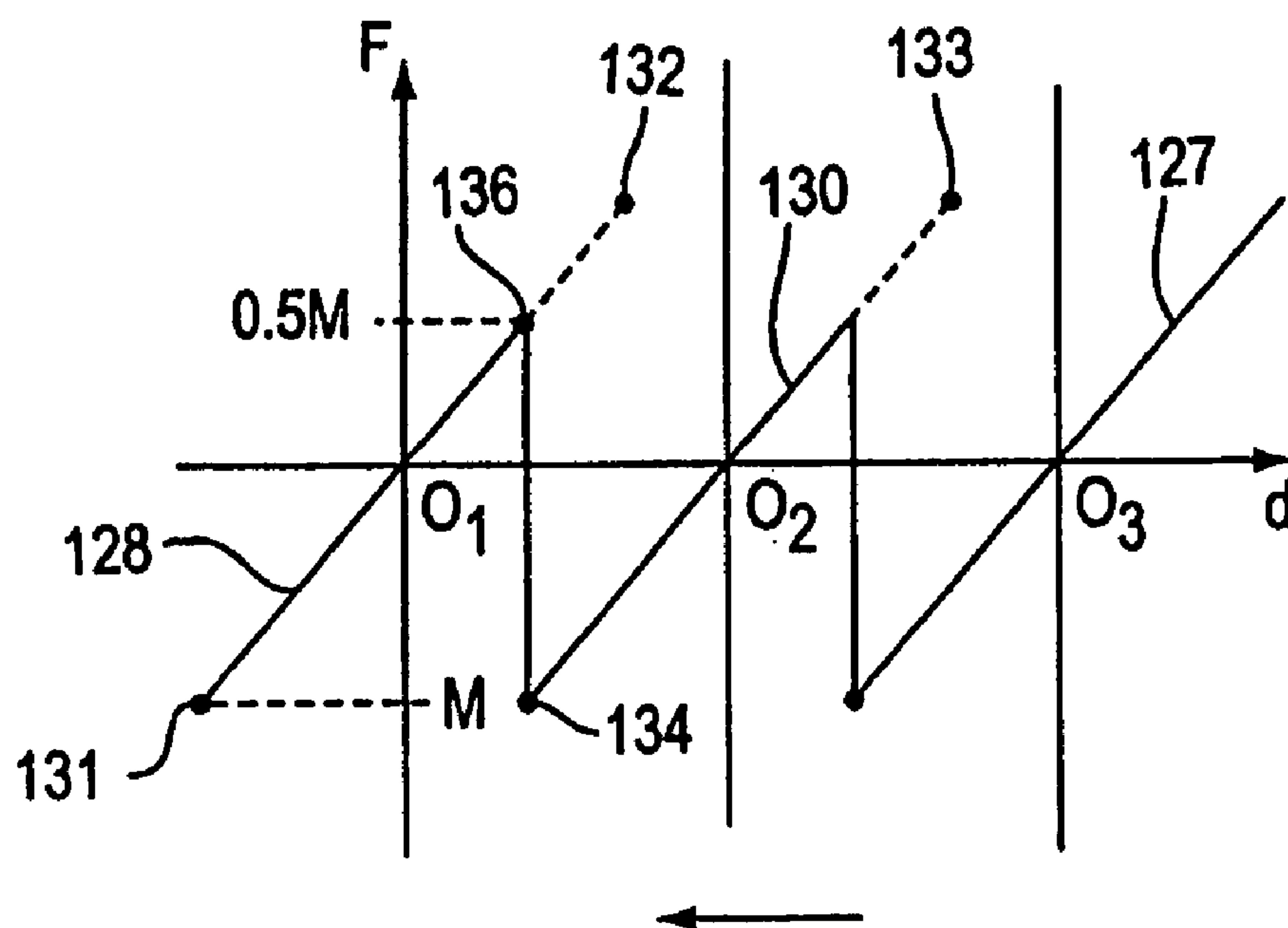
FIG. 6D
