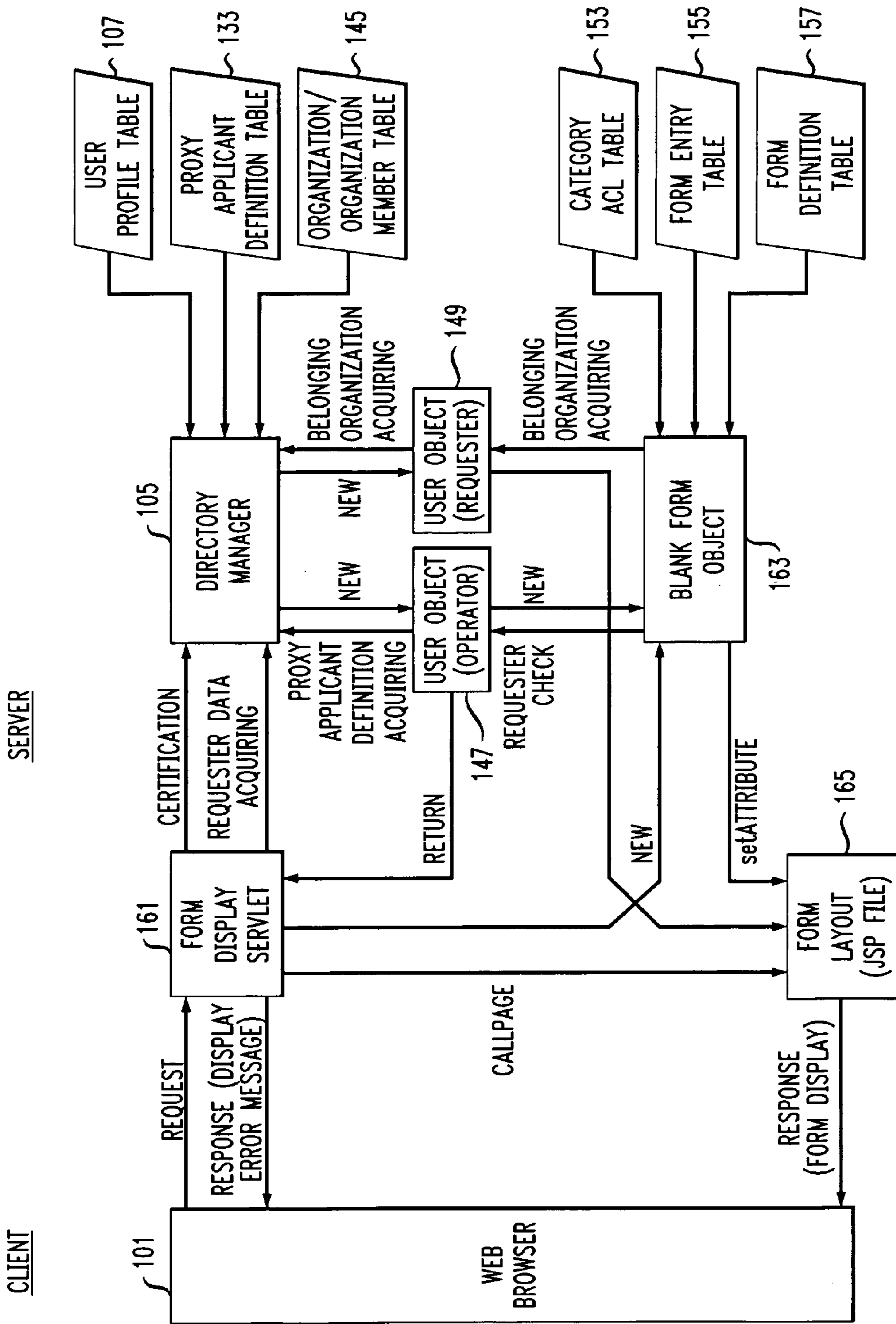
FIG. 6 FORM DISPLAY
