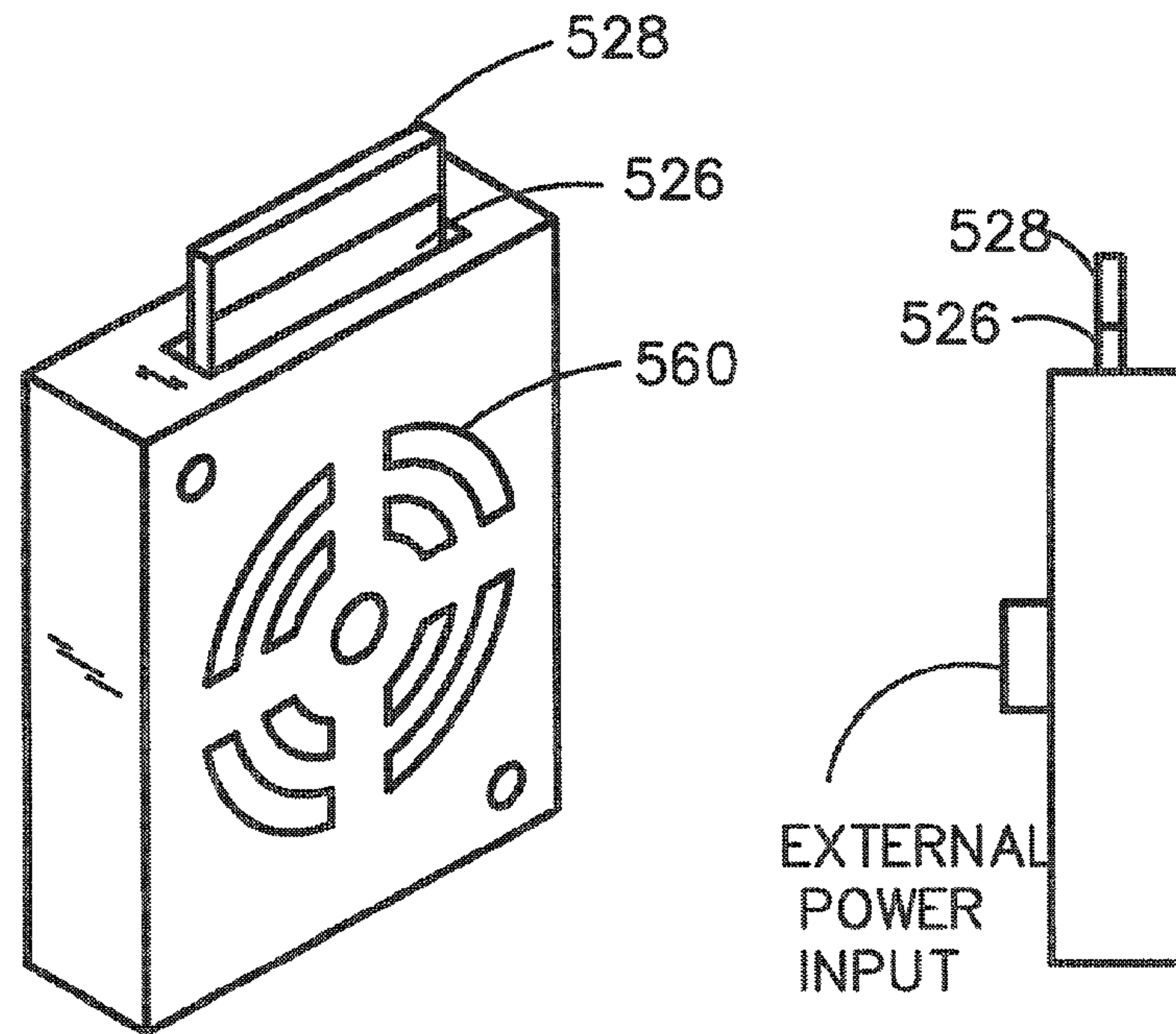
SIREN
