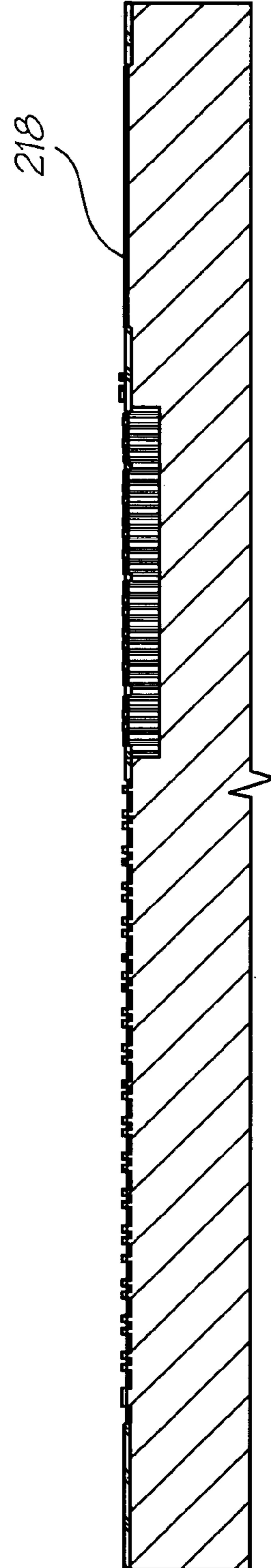
p+ implant
