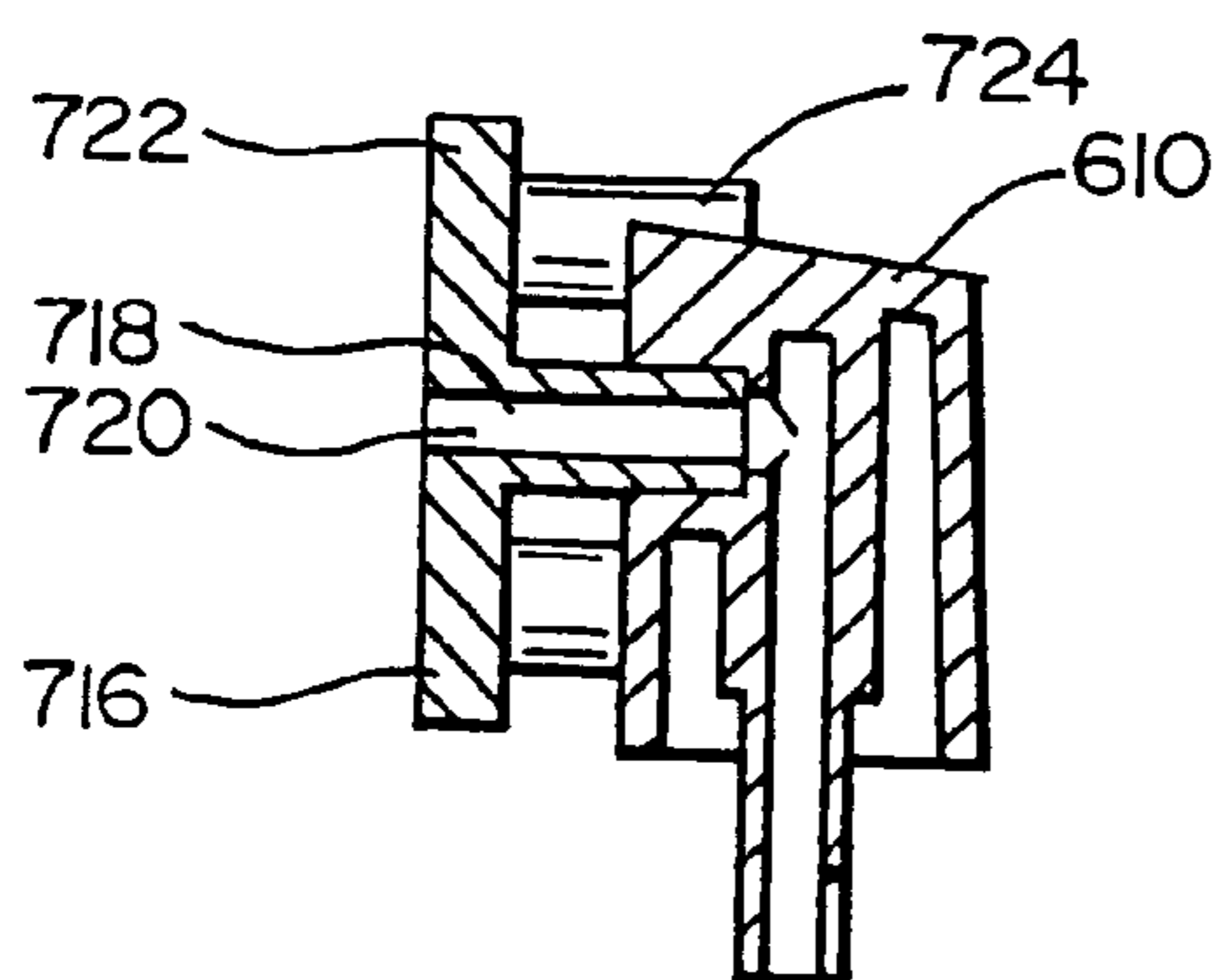
FIG. 38A
