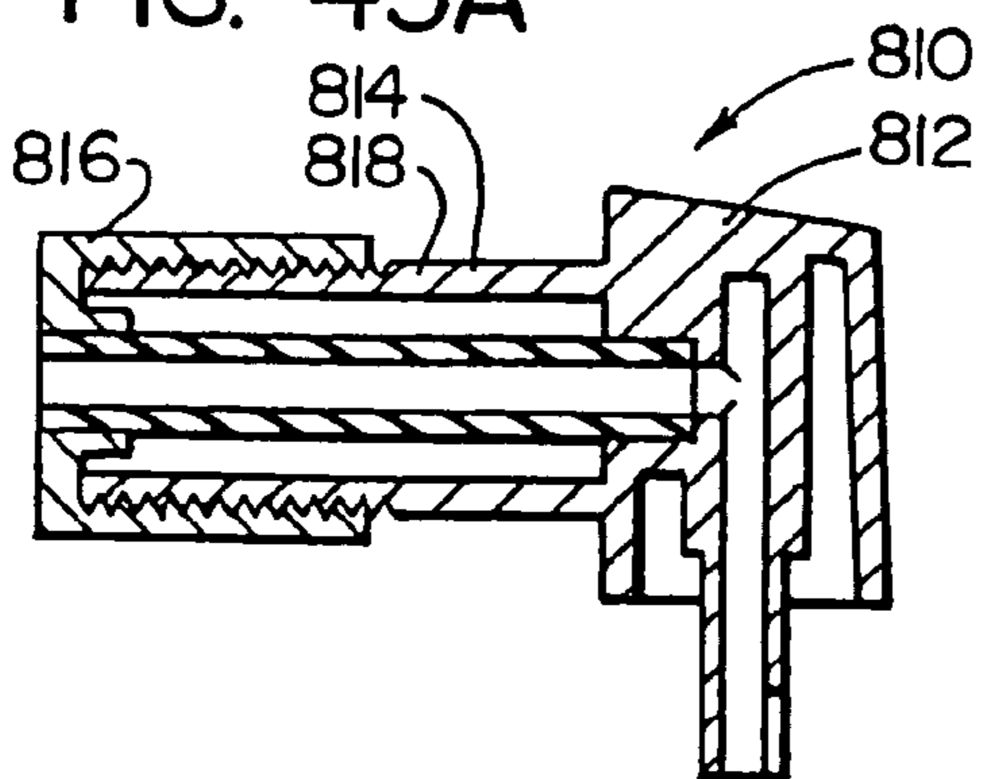
FIG. 43A
