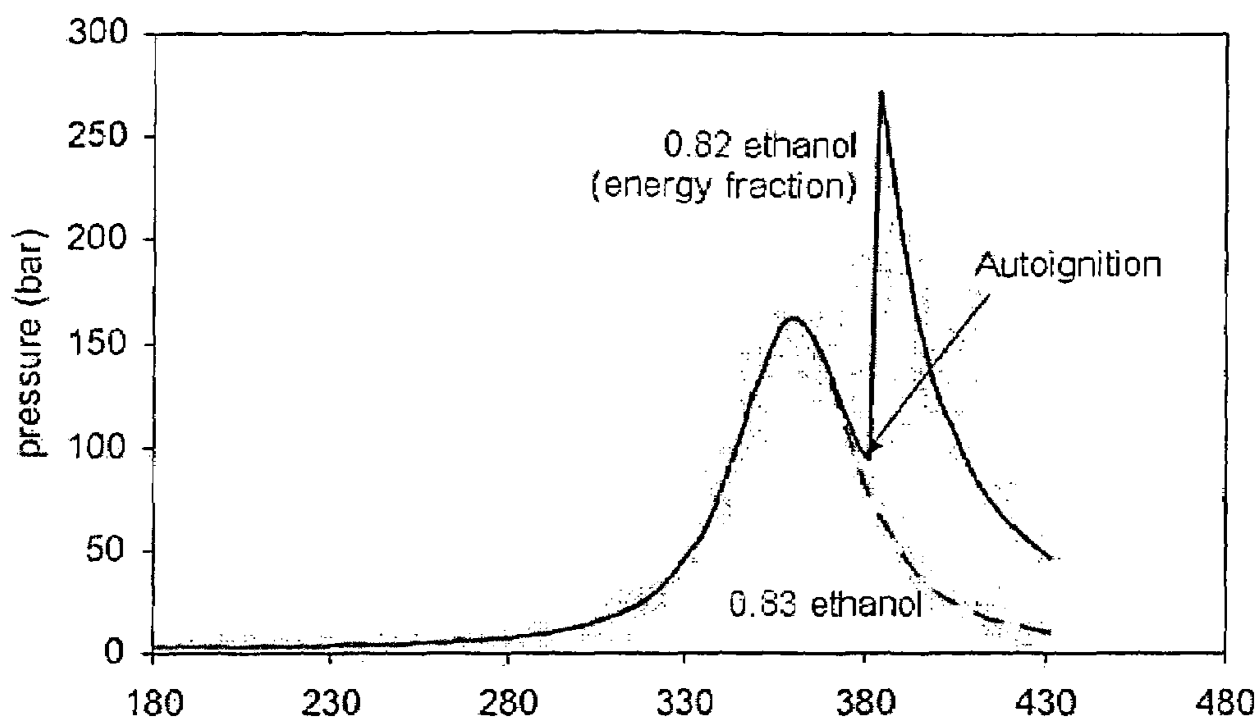
FIG. 2a Crank angle
