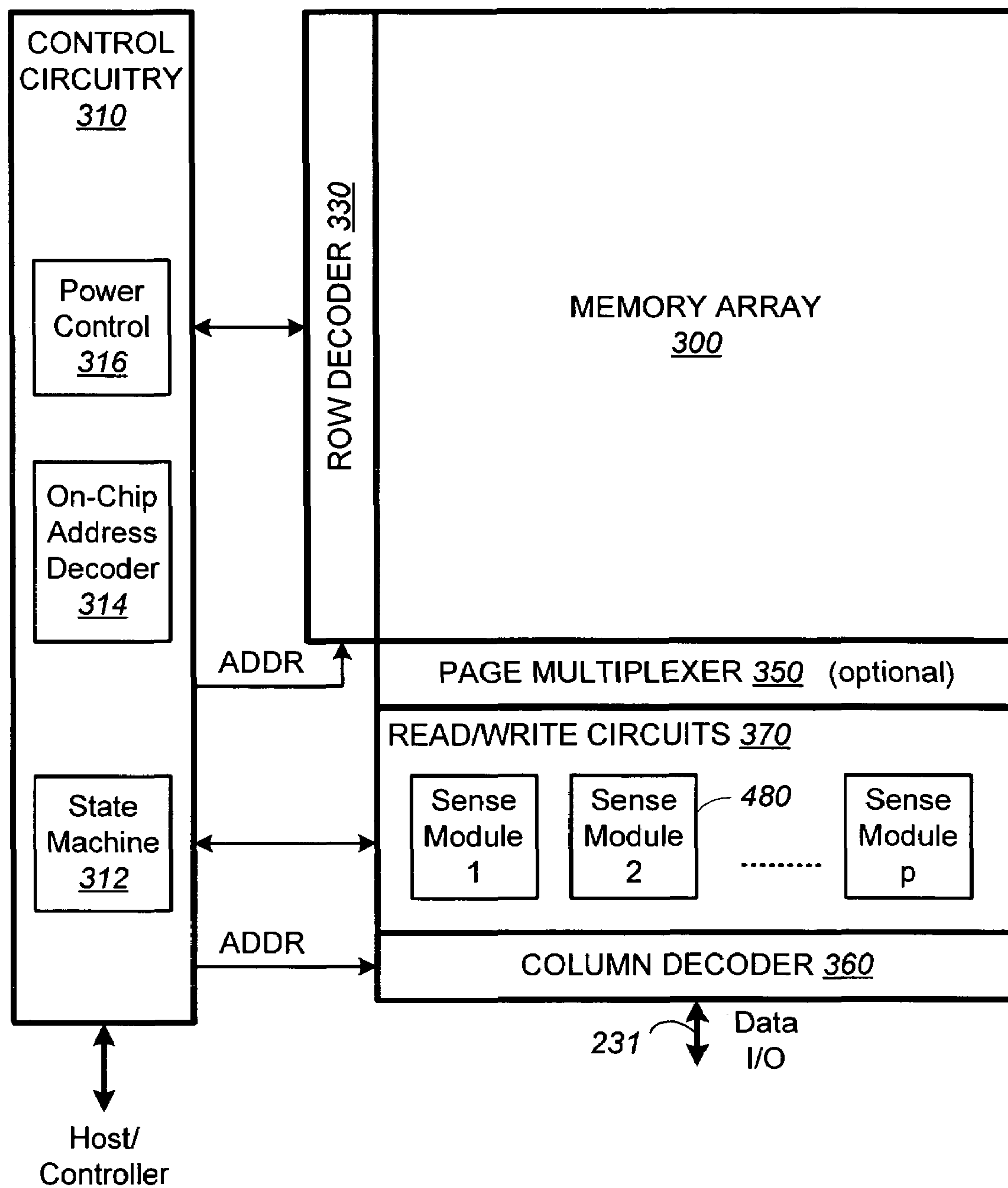
FIG. 6A
