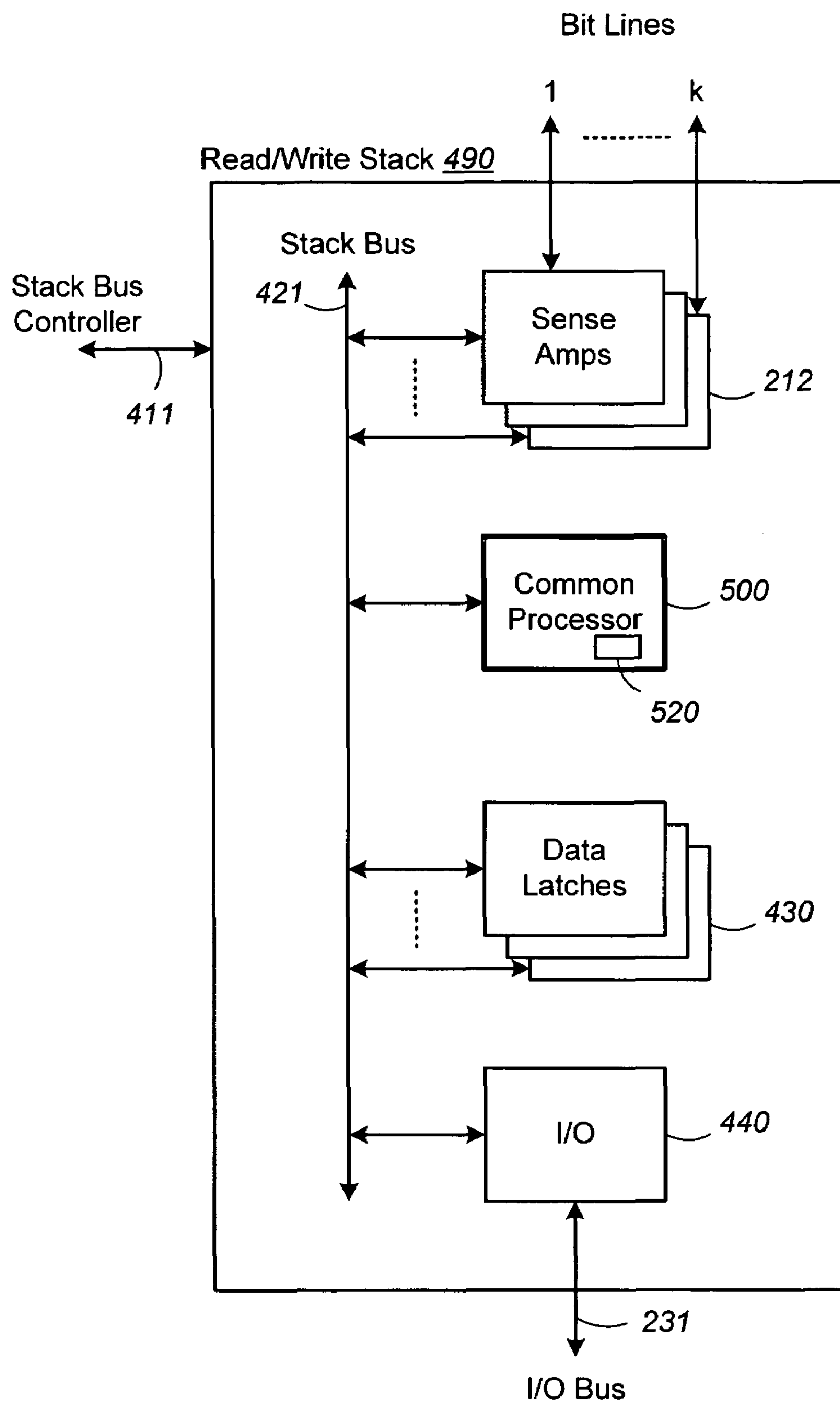
FIG. 6D
