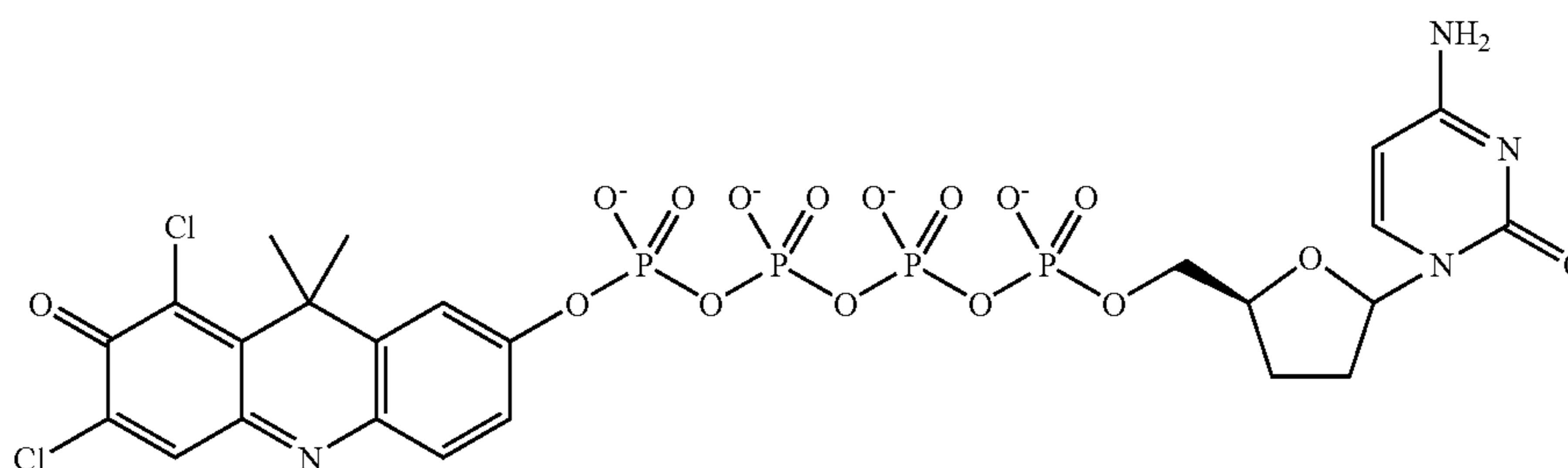
ddC4P-DDAO
