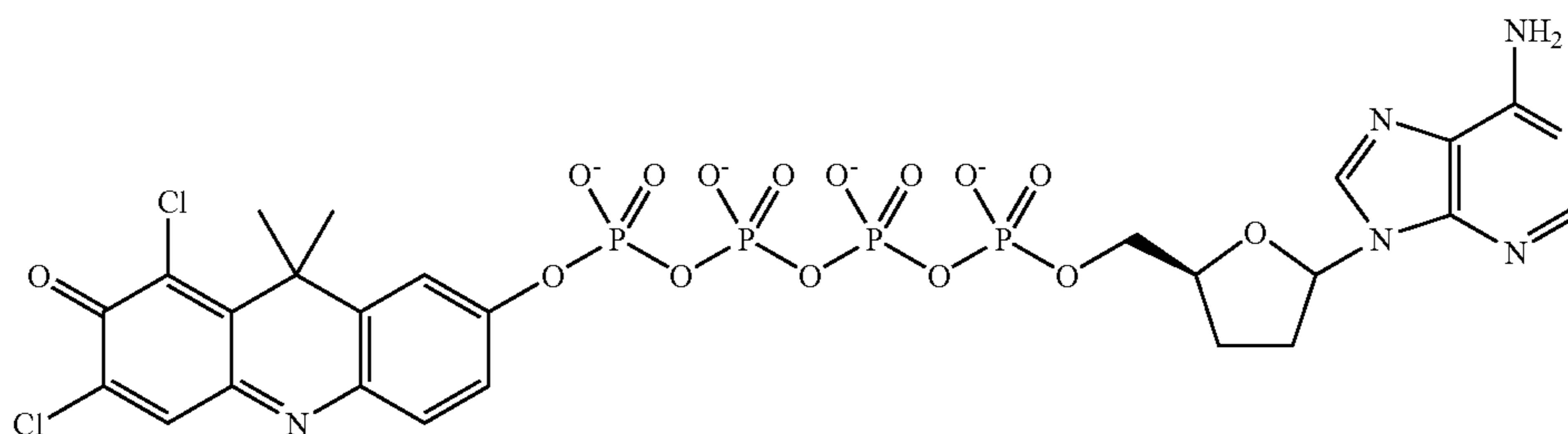
ddA4P-DDAO
