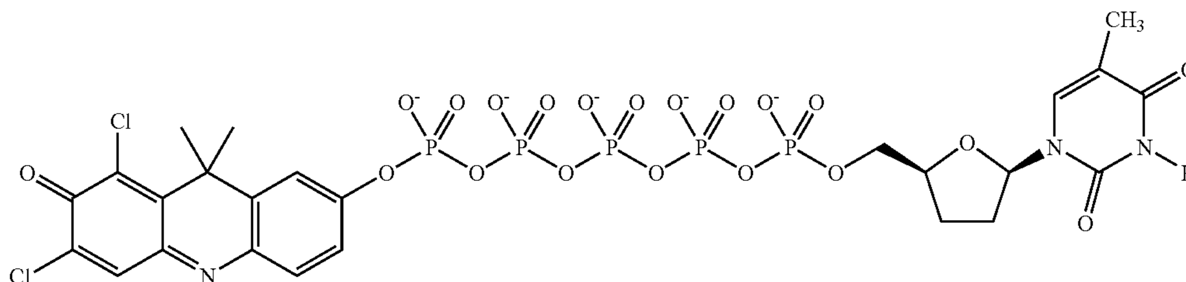
ddT5P-DDAO
