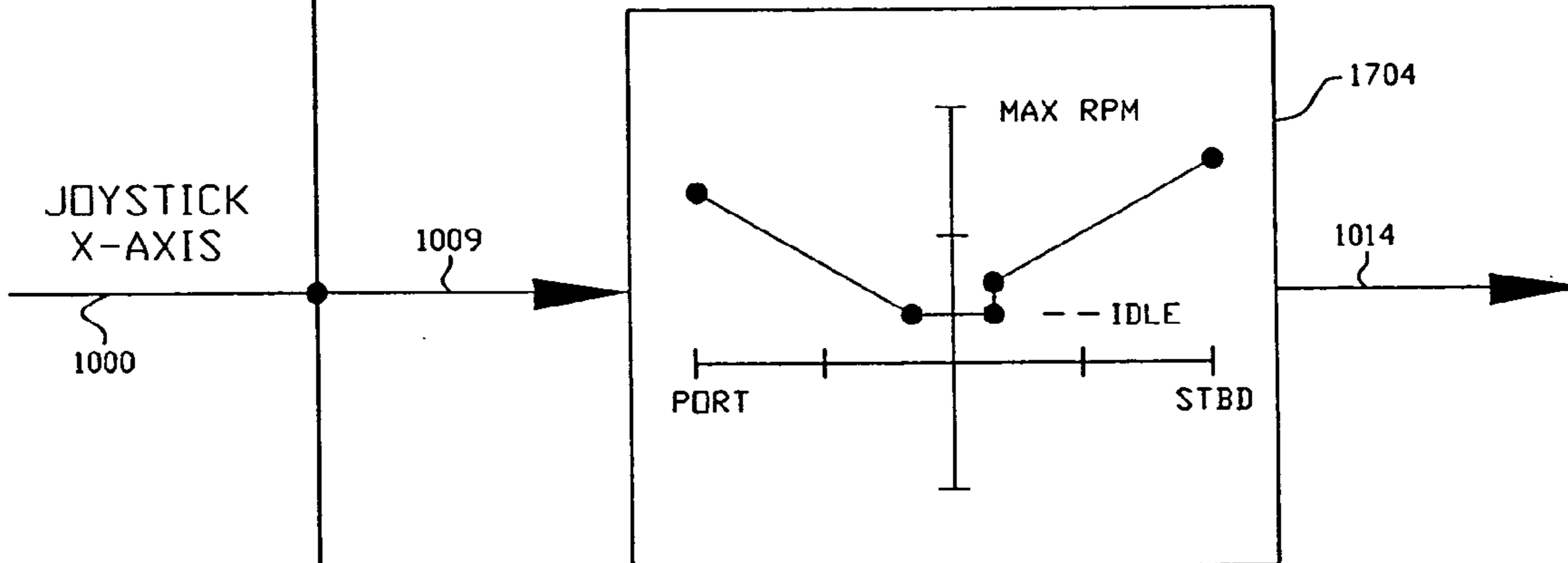
FIG. 15E STBD ENGINE RPM
