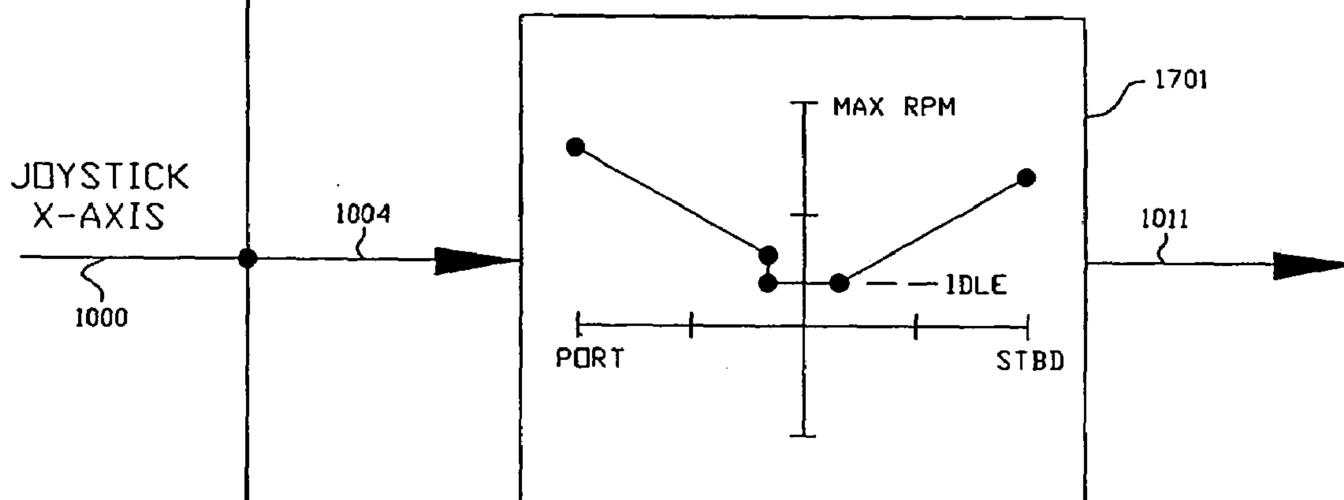
FIG. 14E PORT ENGINE RPM
