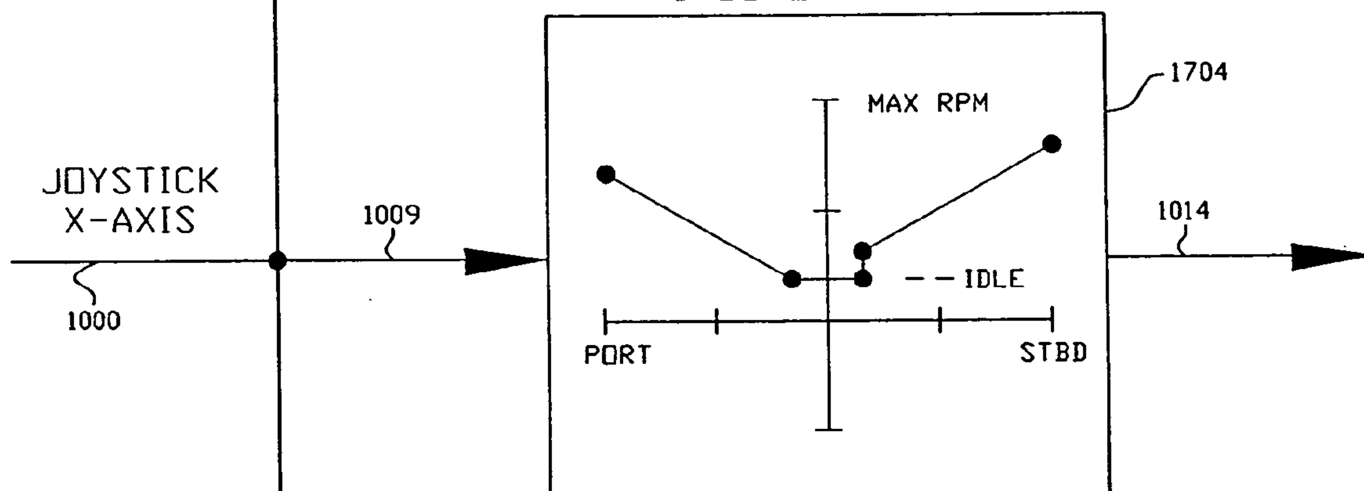
FIG. 15E STBD ENGINE RPM
