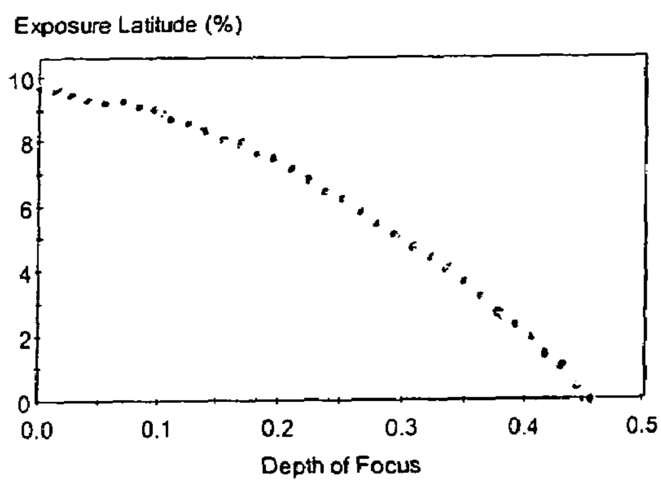
Exposure Latitude vs. DOF
