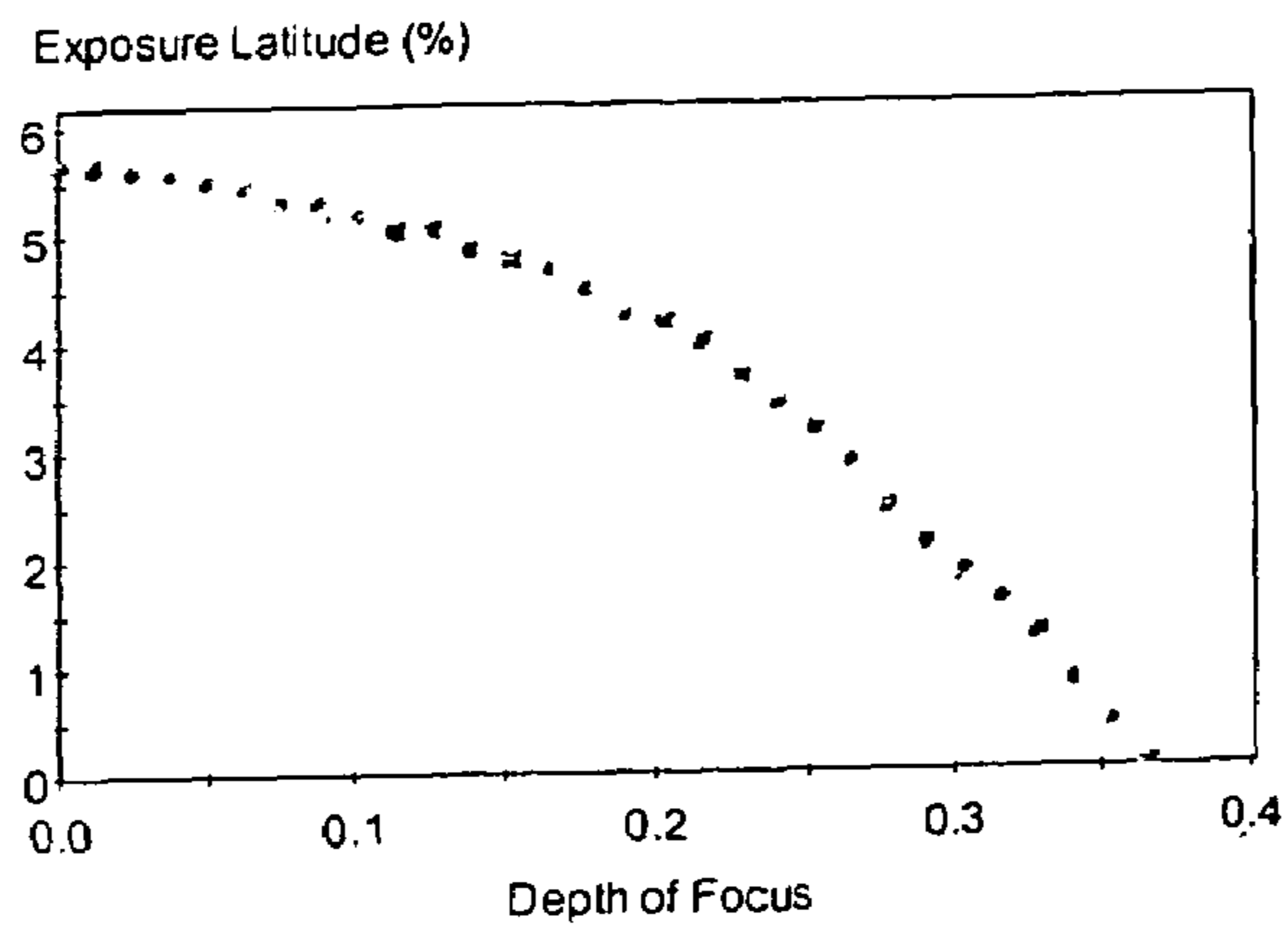
Exposure Latitude vs. DOF
