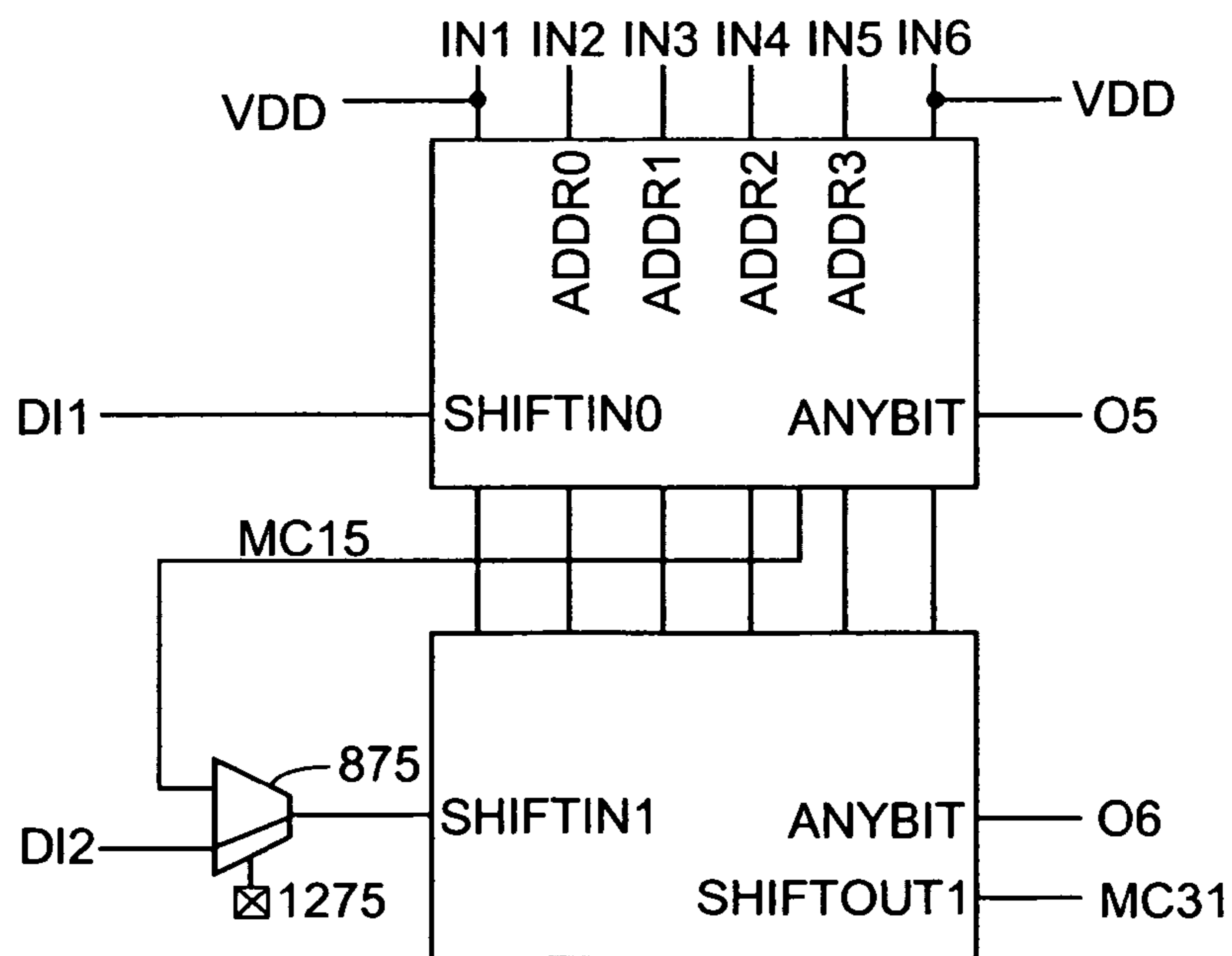
FIG. 13 (16x2 SRL)
