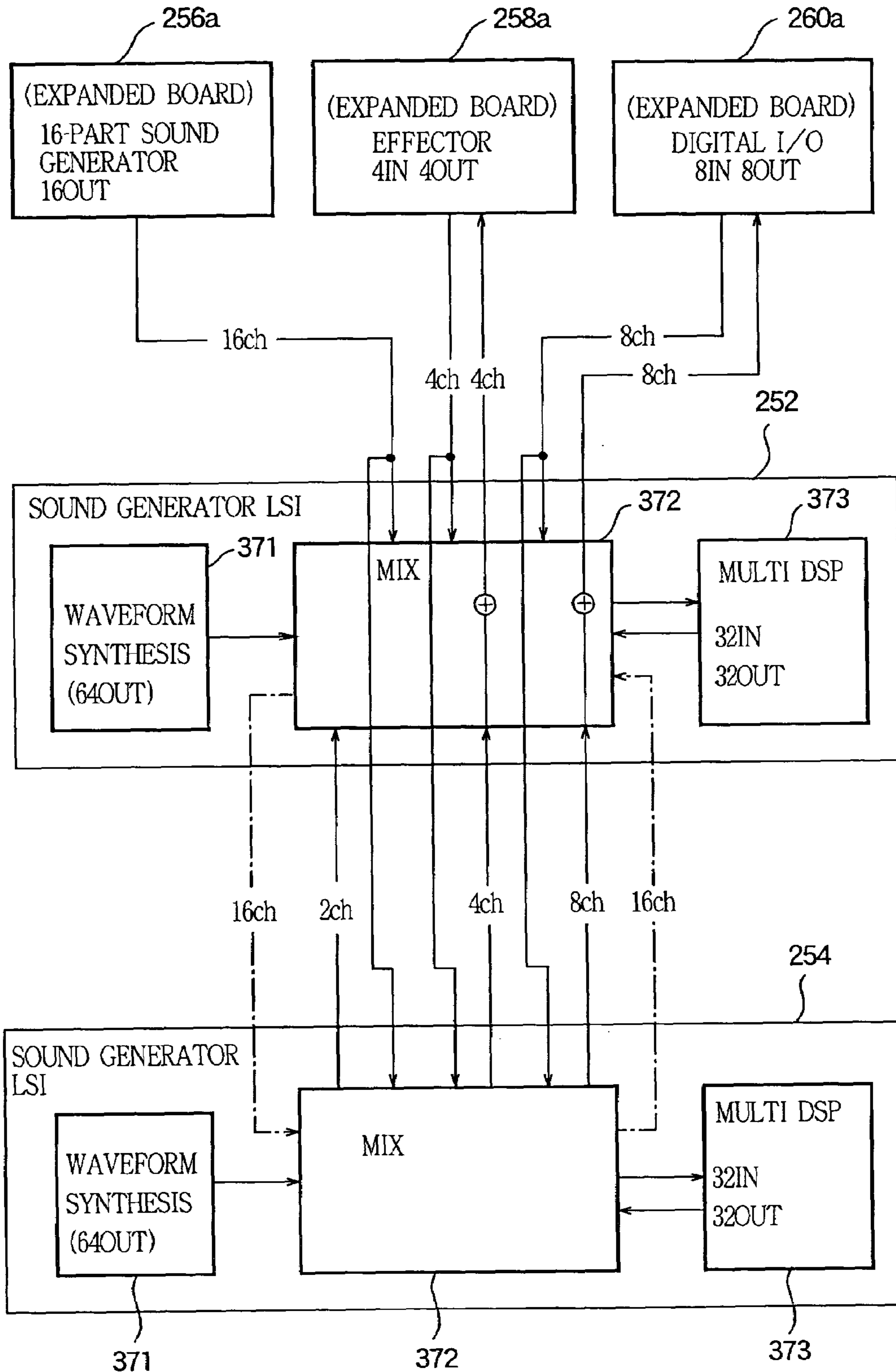
FIG. 13
