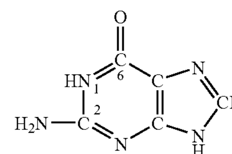
Cosimine (2-amino-6-oxypurine)
