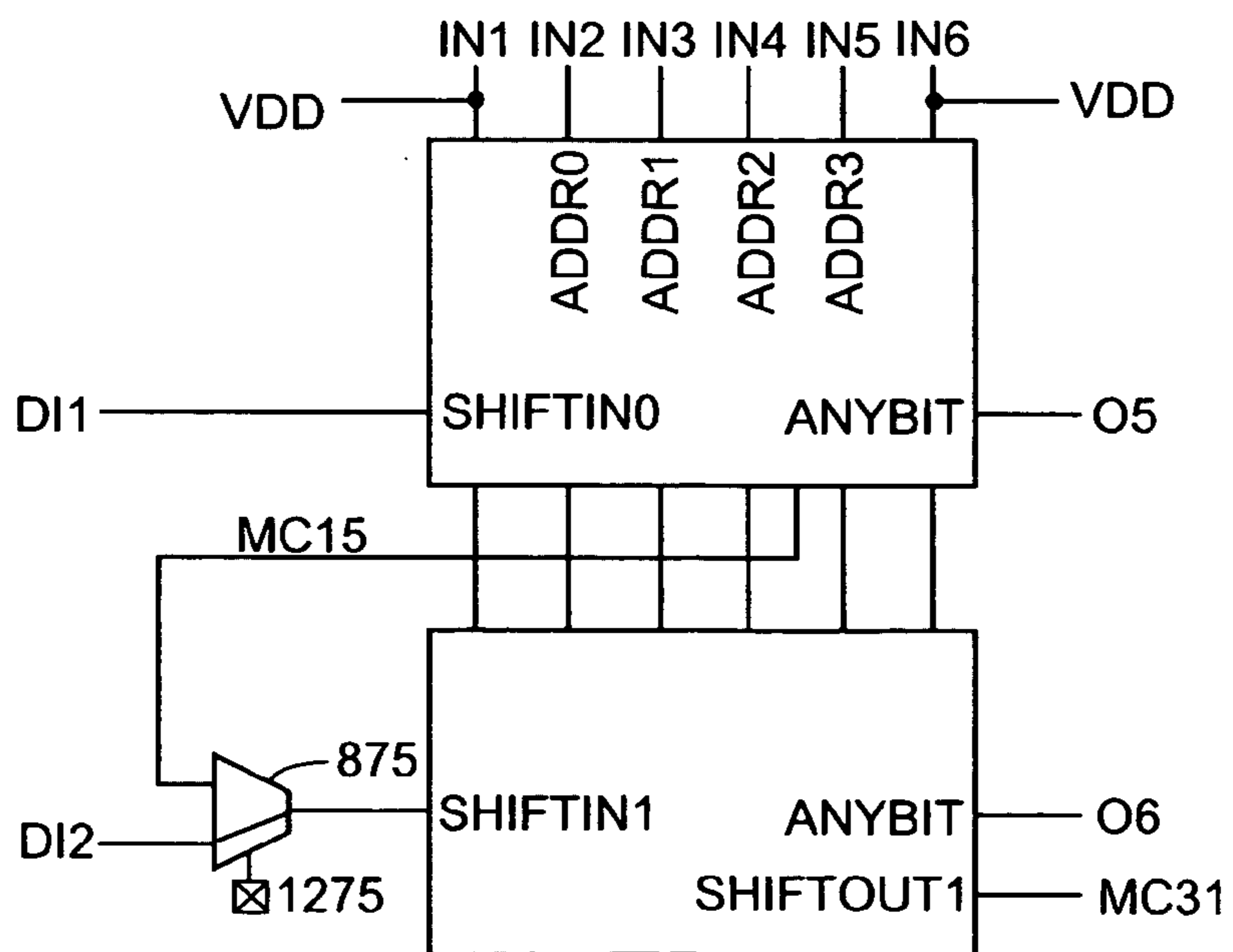
FIG. 13 (16x2 SRL)
