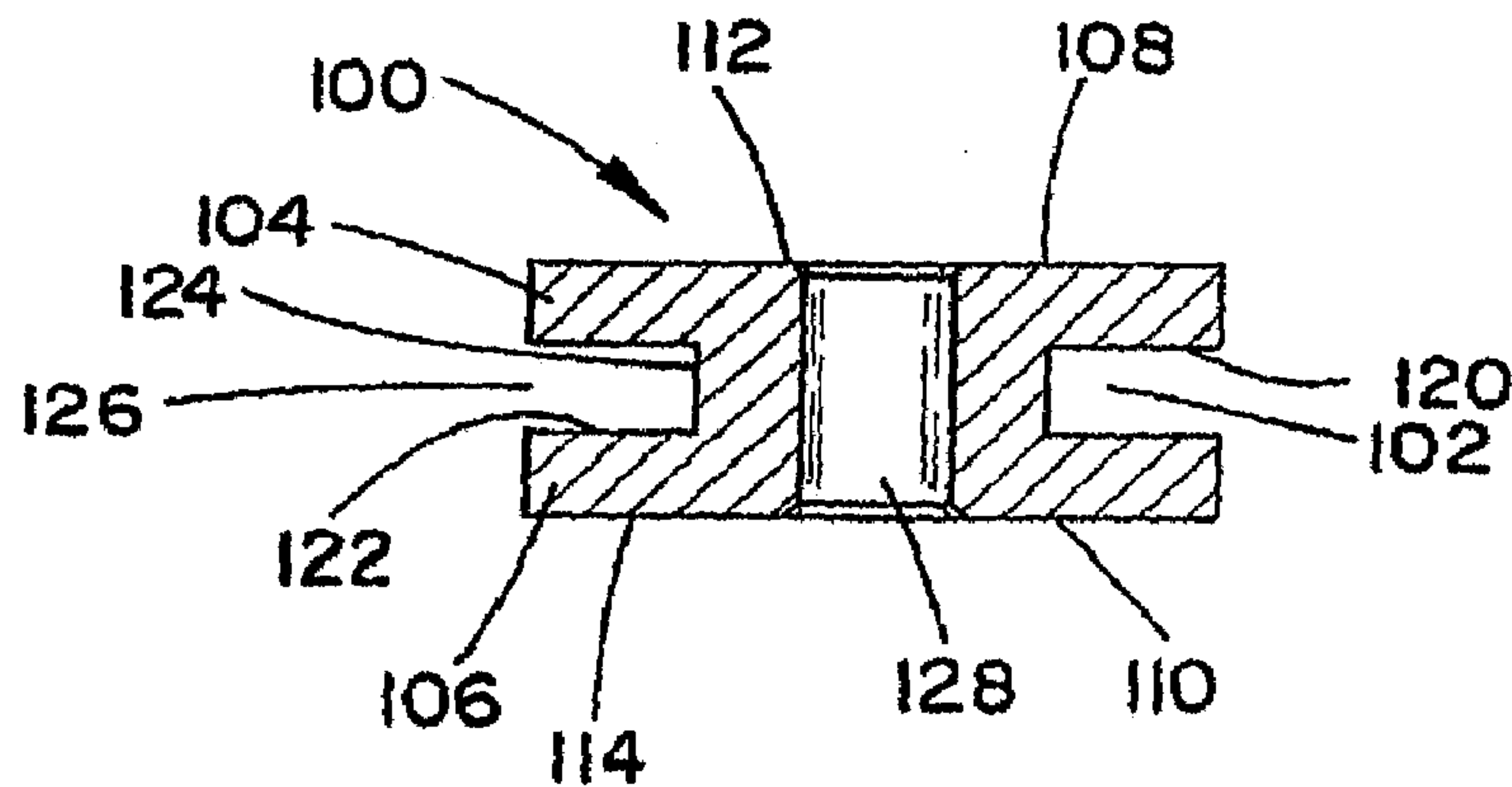
Section A-A
