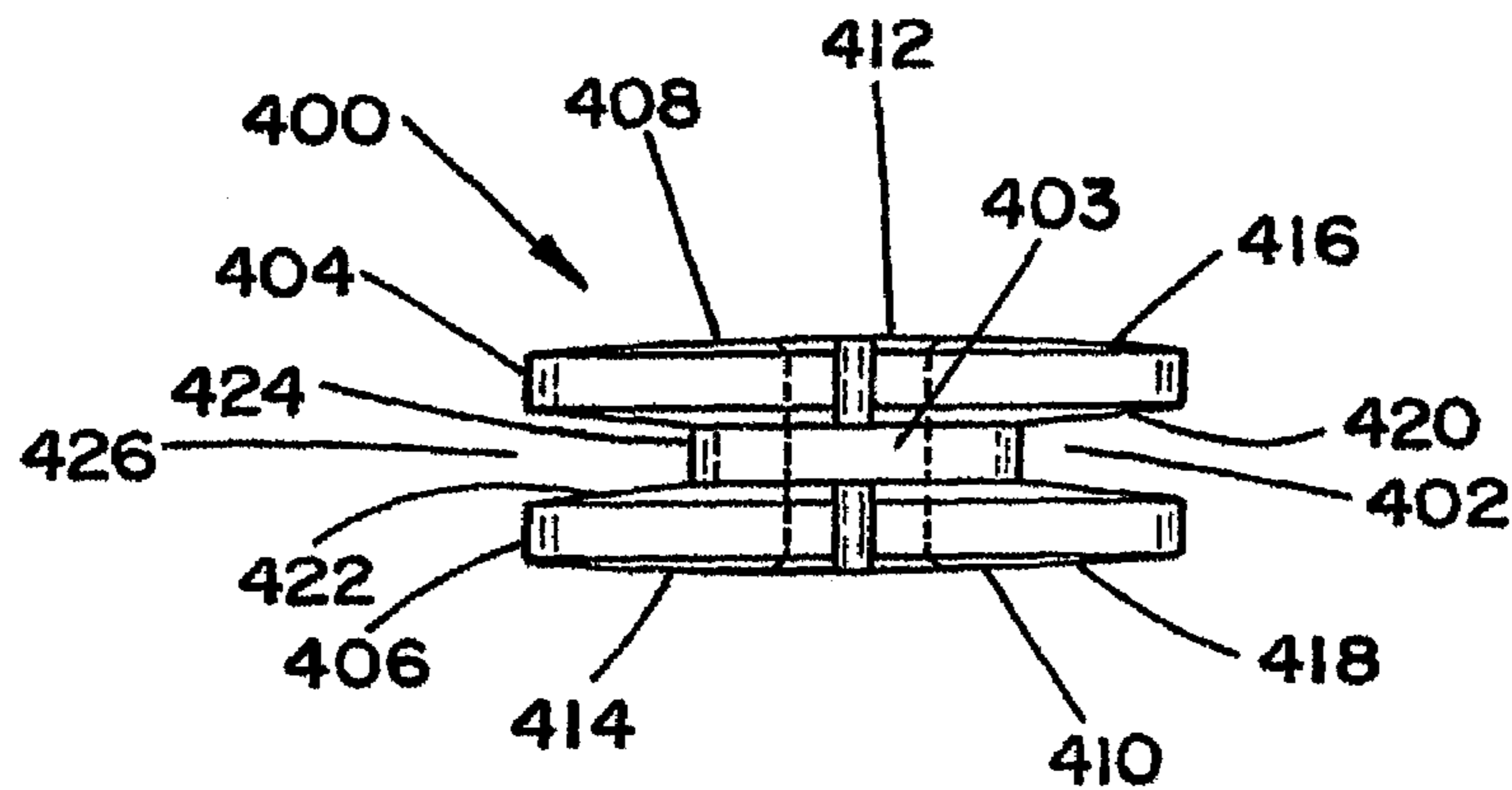
Section B-B FIG. 4b
