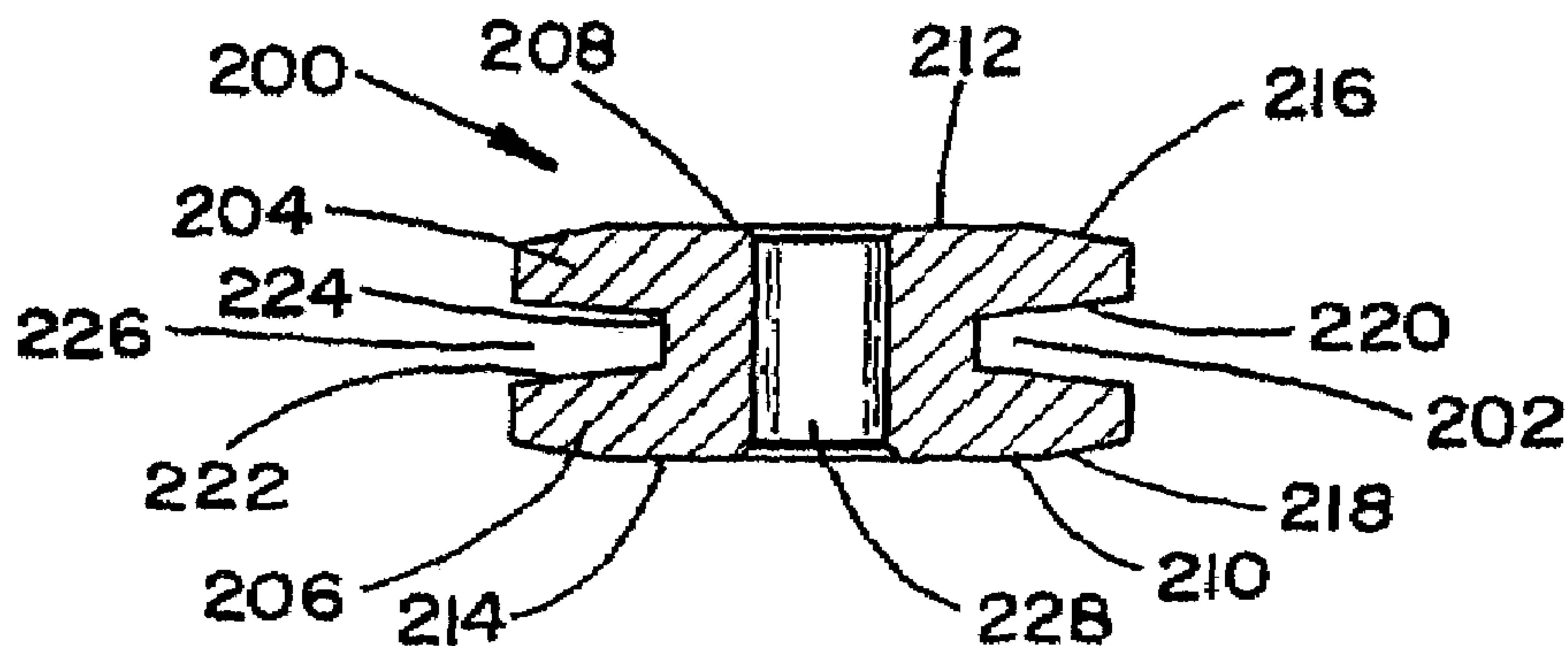
Section A-A
