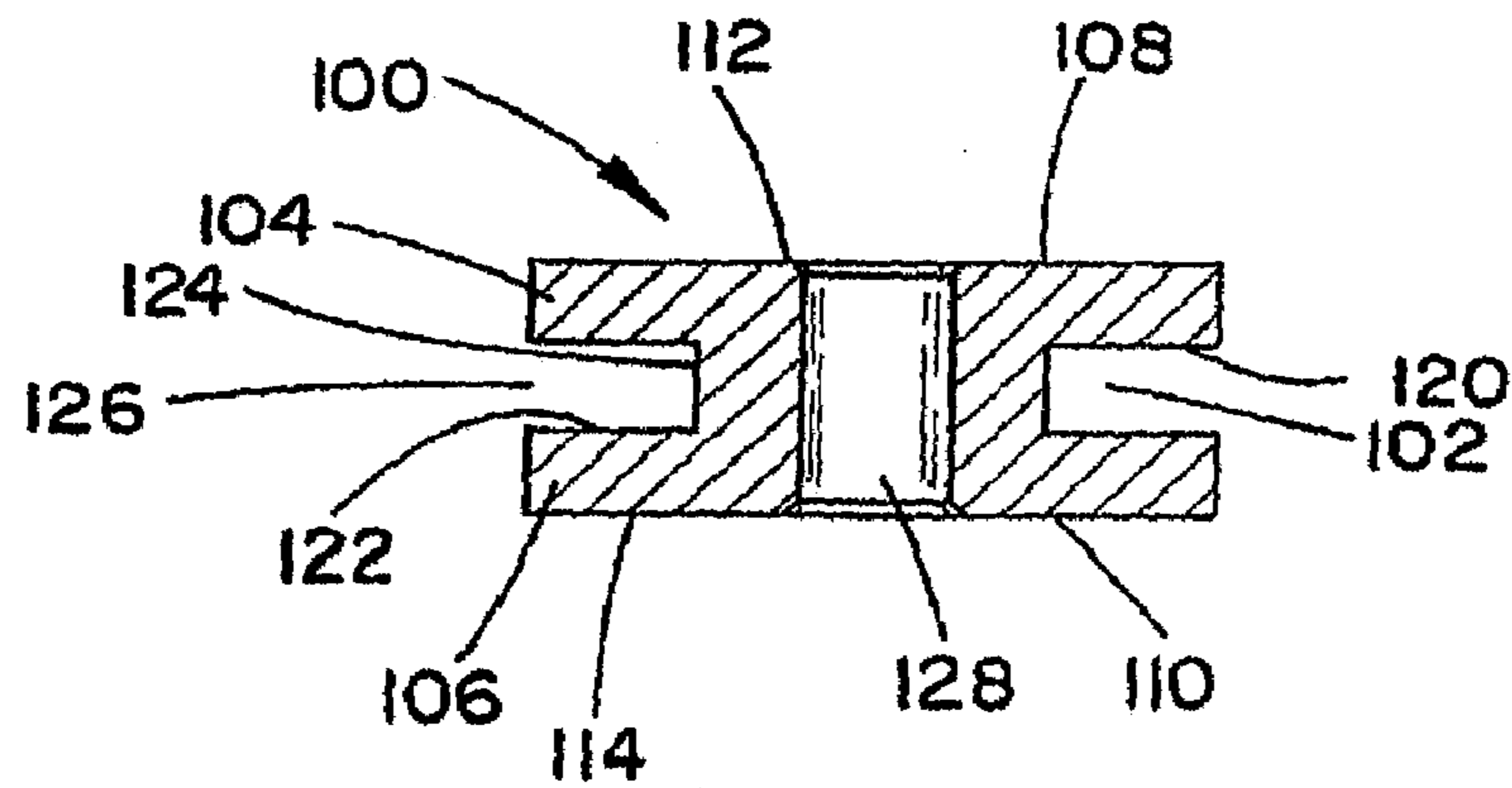
Section A-A FIG. 1c
