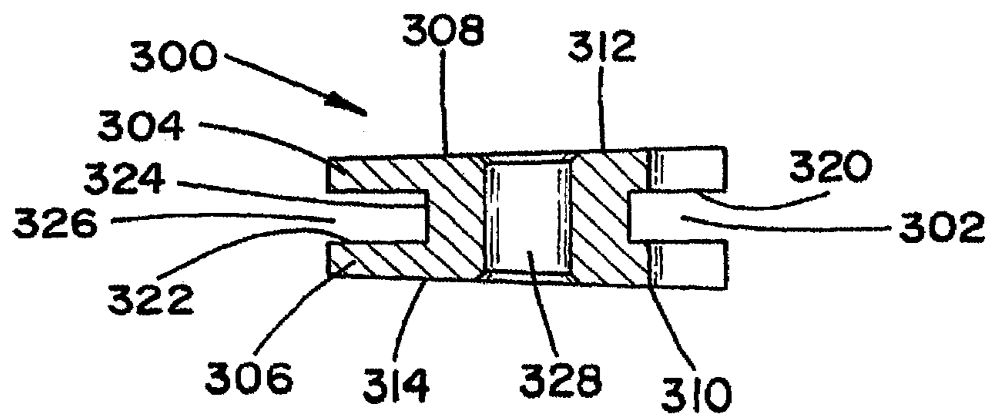
Section A-A FIG. 3c
