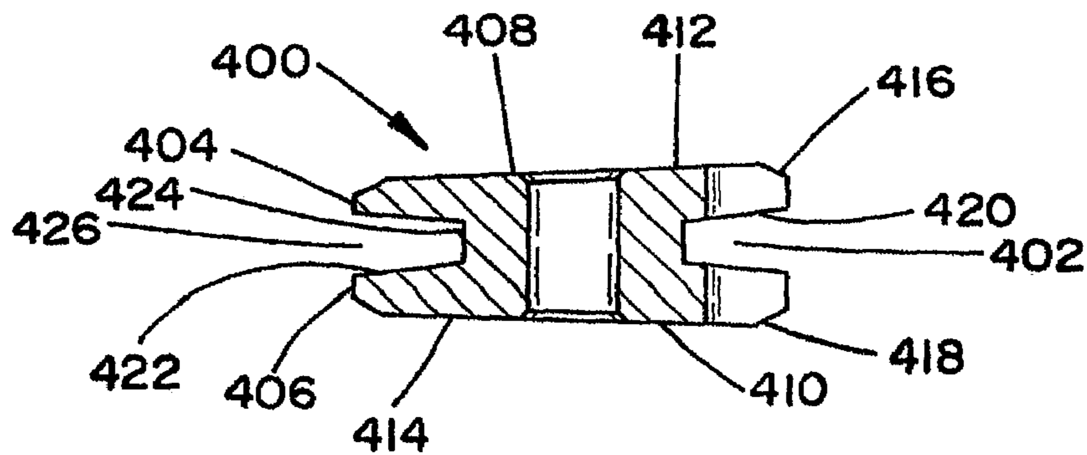
Section A-A FIG. 4c
