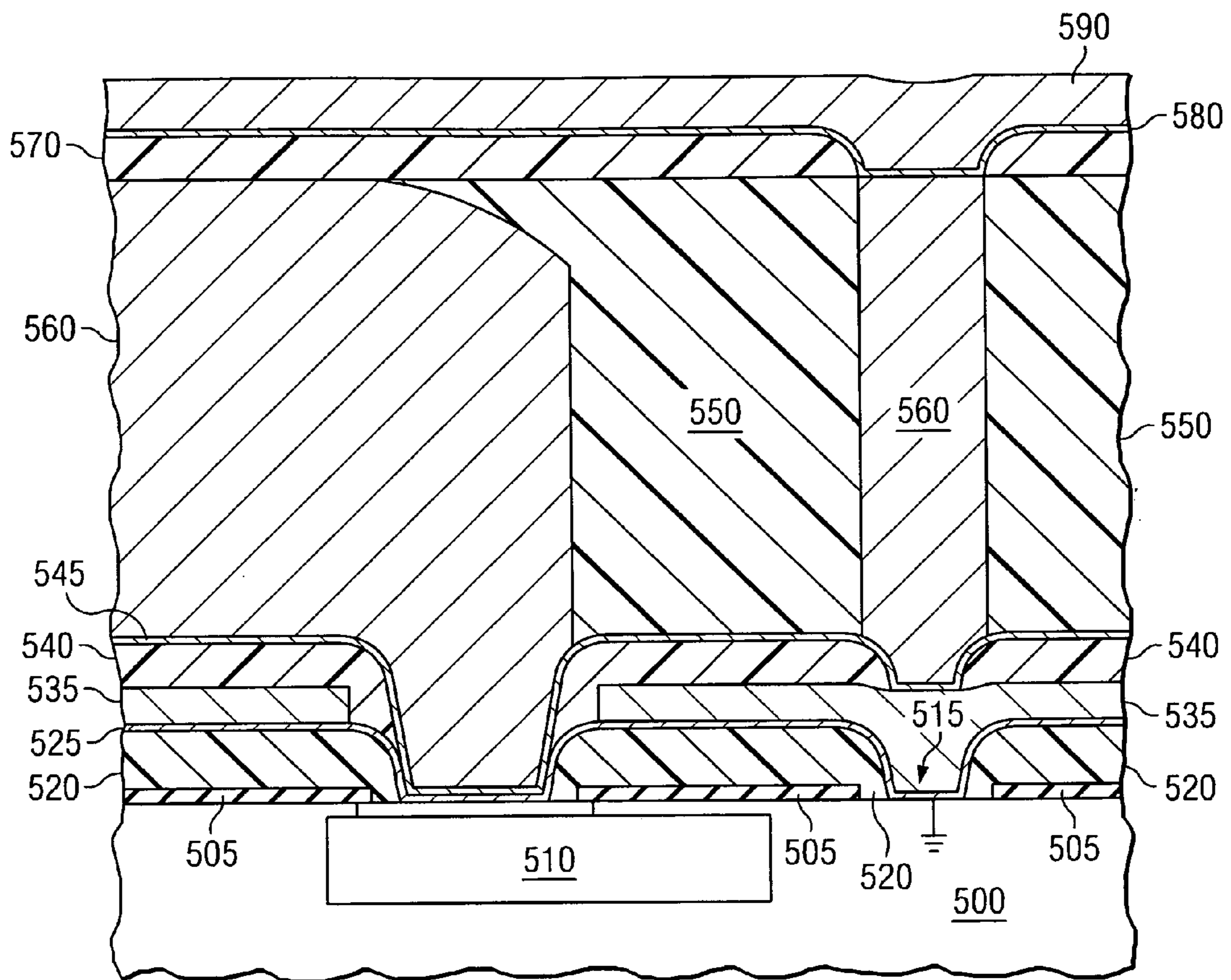
FIG. 5H
