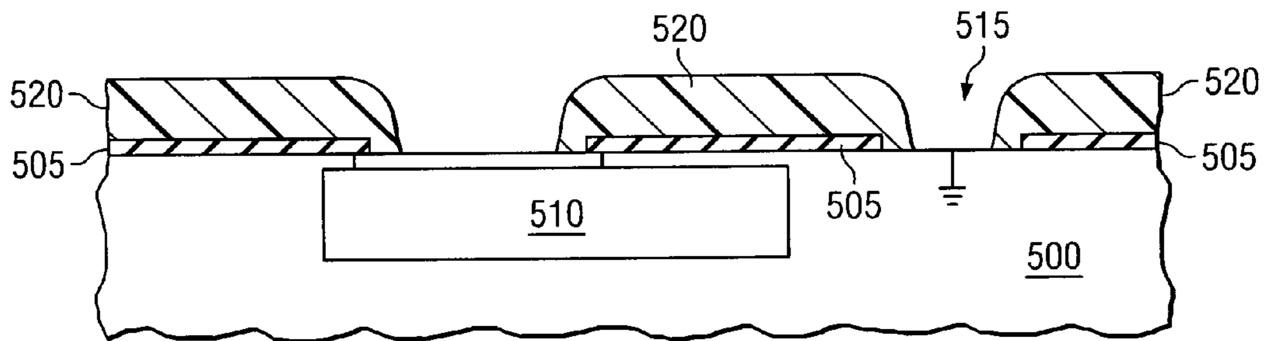
FIG. 5B
