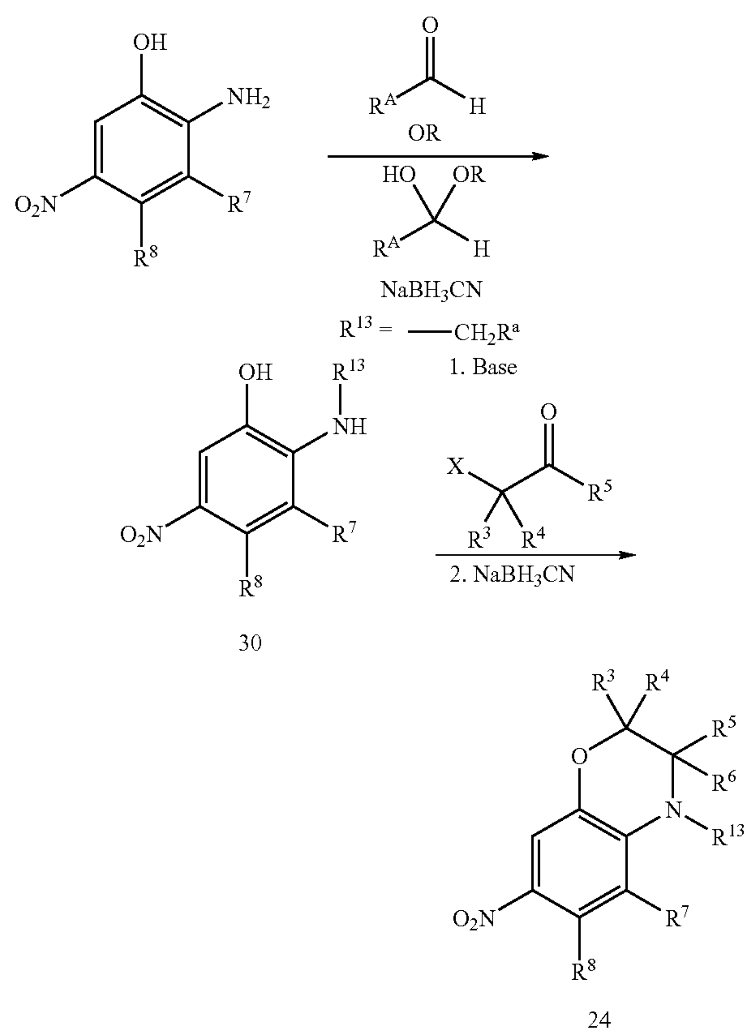
Scheme VI
