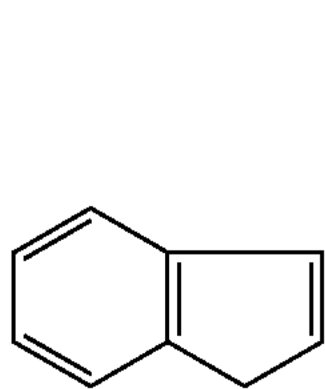
Indene
