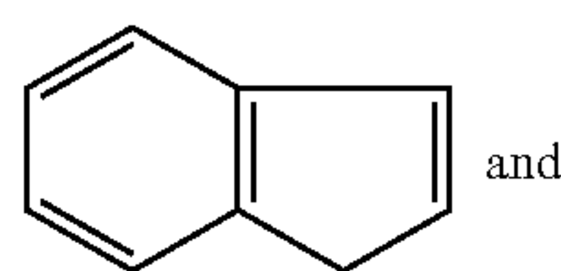
Indene
