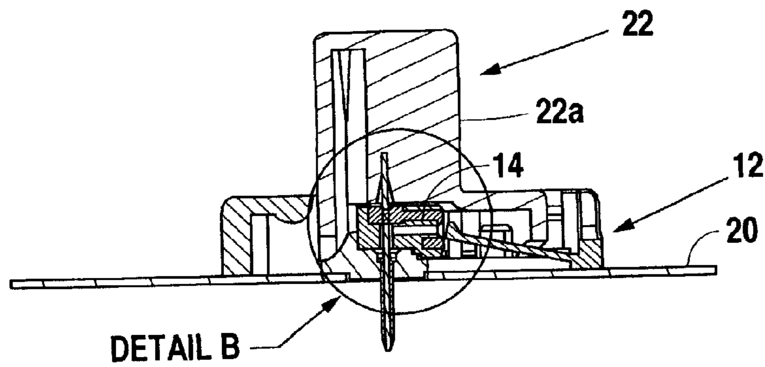
Fig. 3A ( SECTION A-A )
