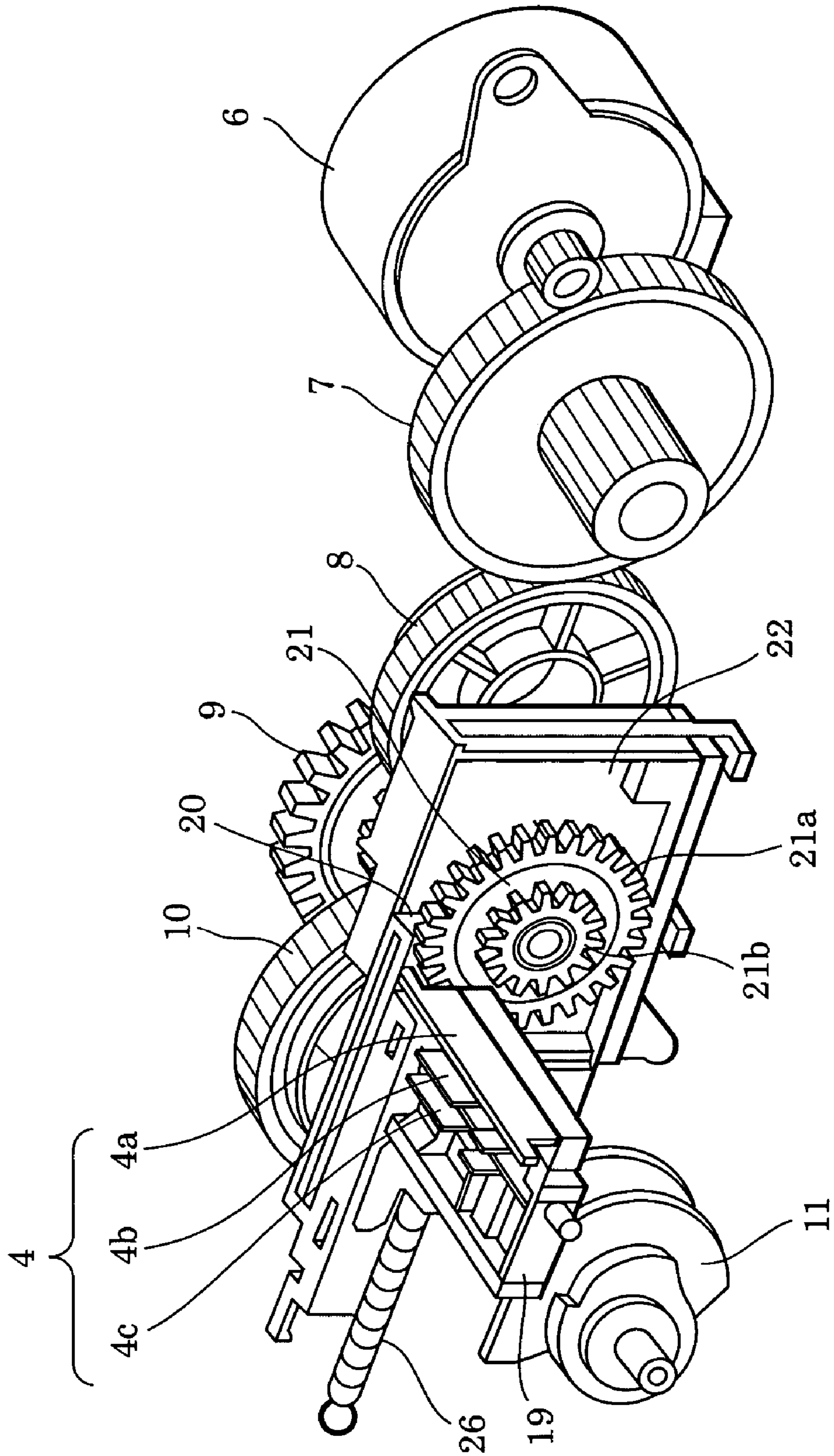
FIG. 5
