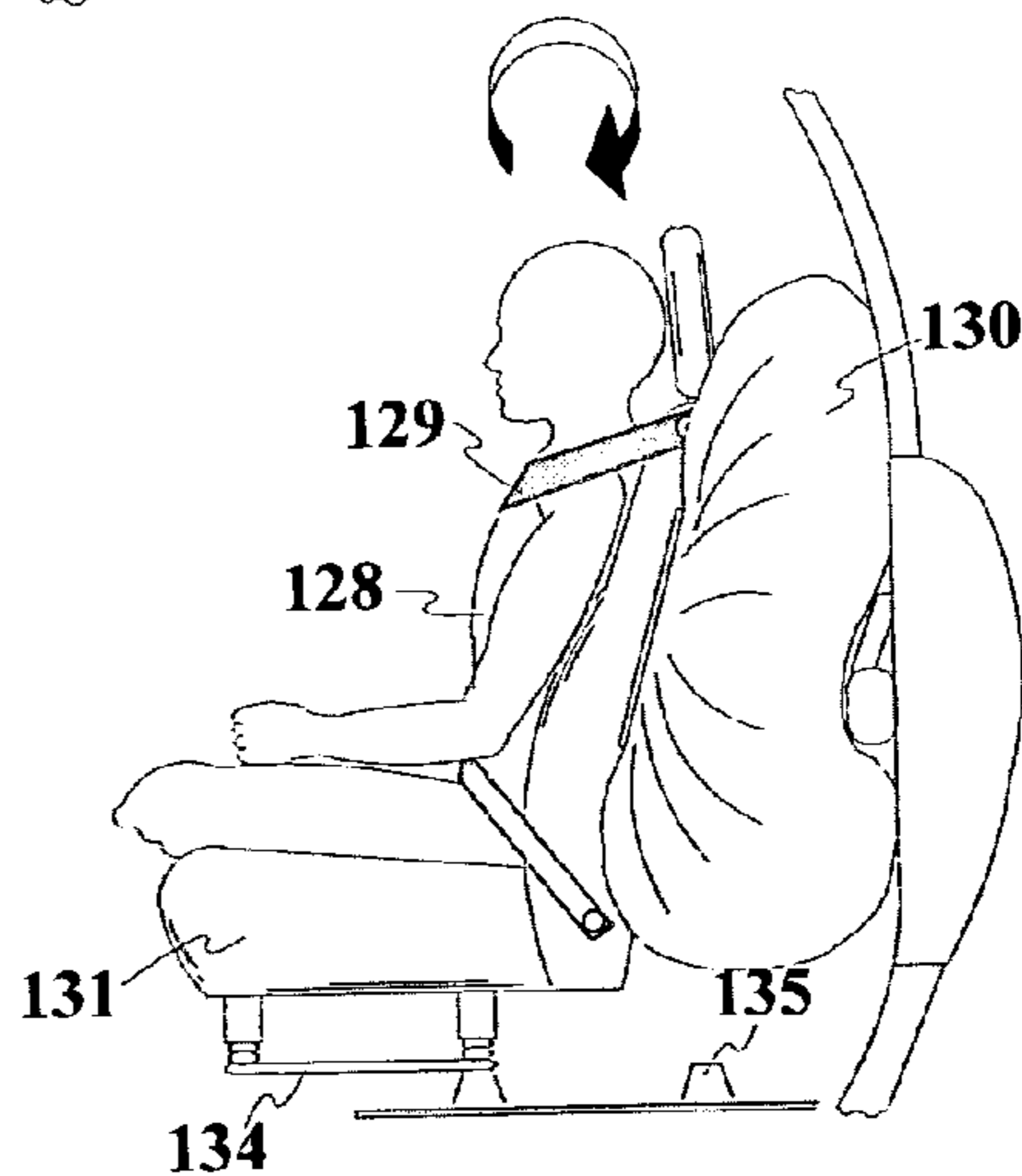
FIG. 25B
