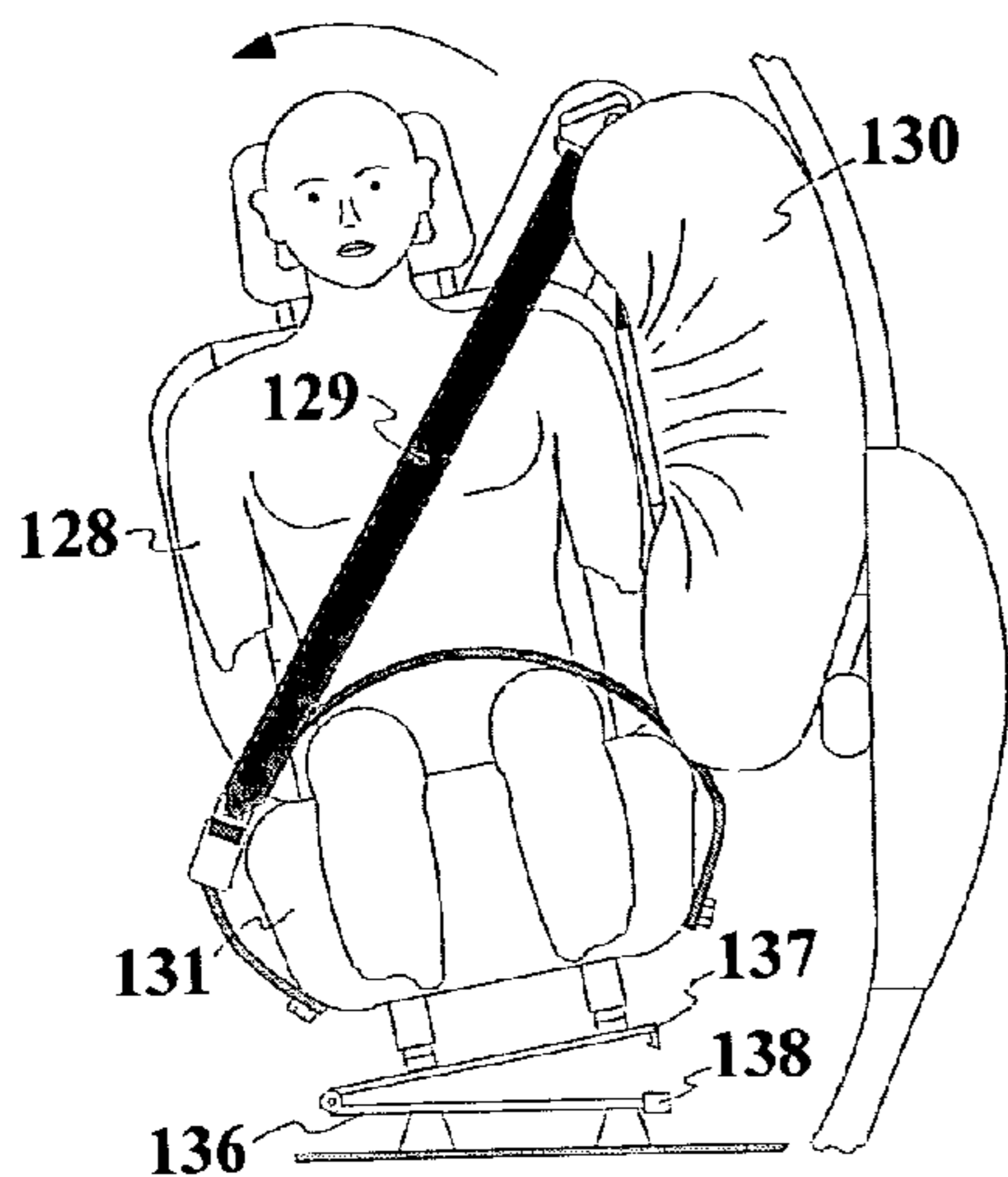
FIG. 25C
