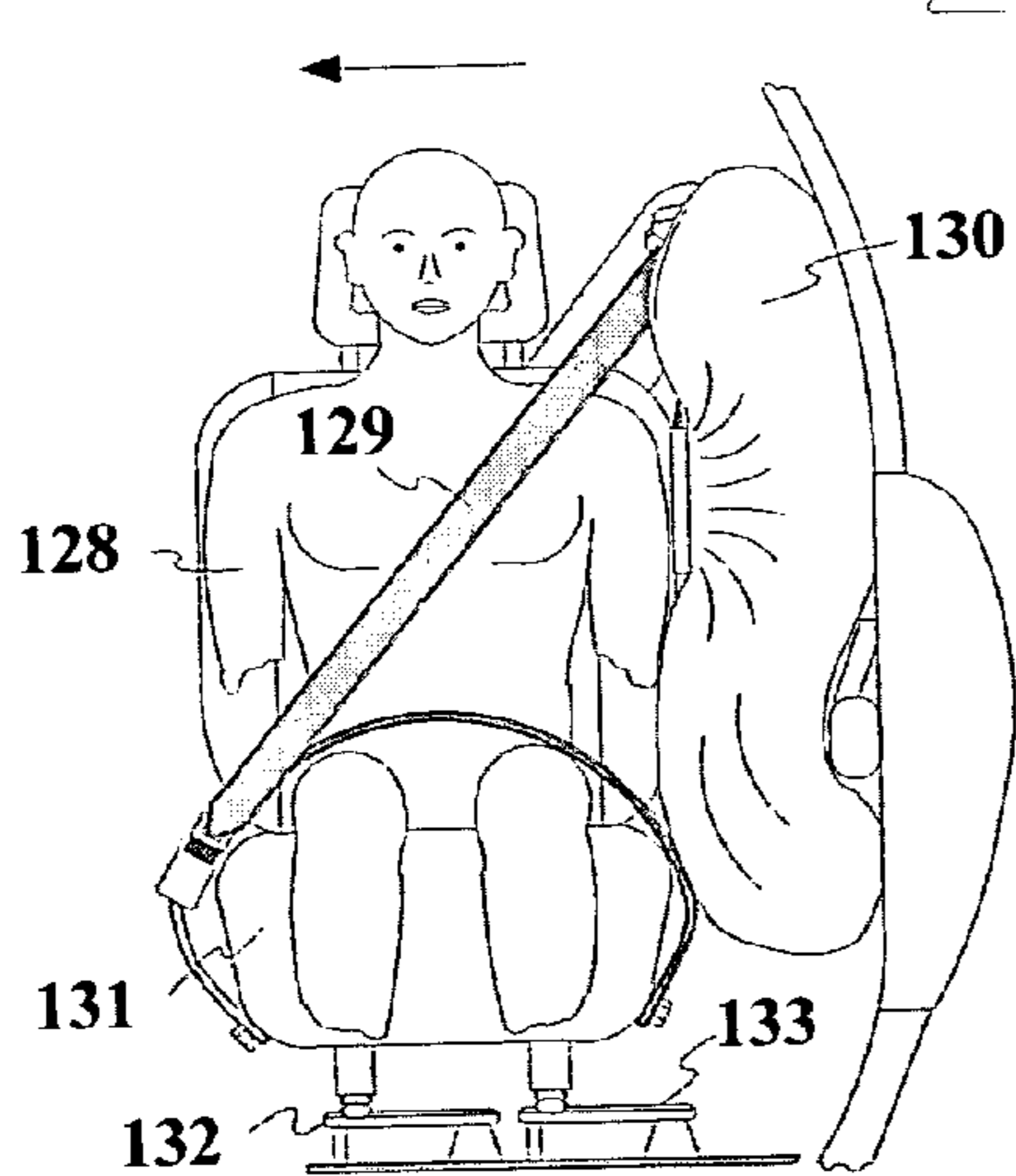
FIG. 25A
