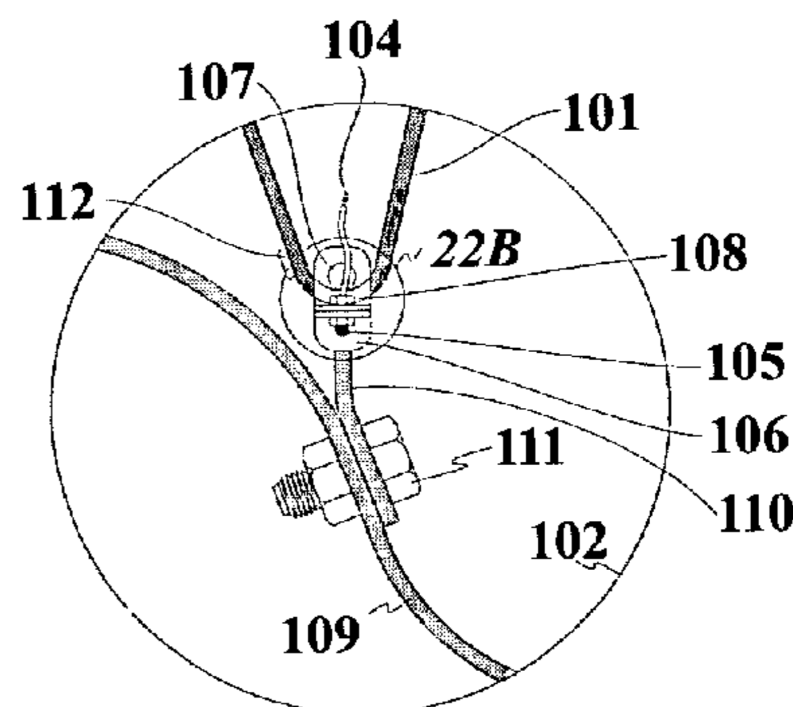
FIG. 22A
