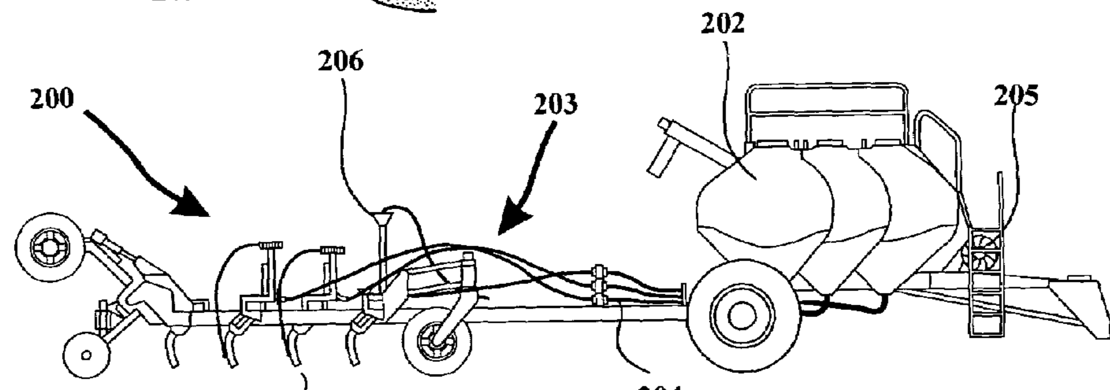
FIG. 39
