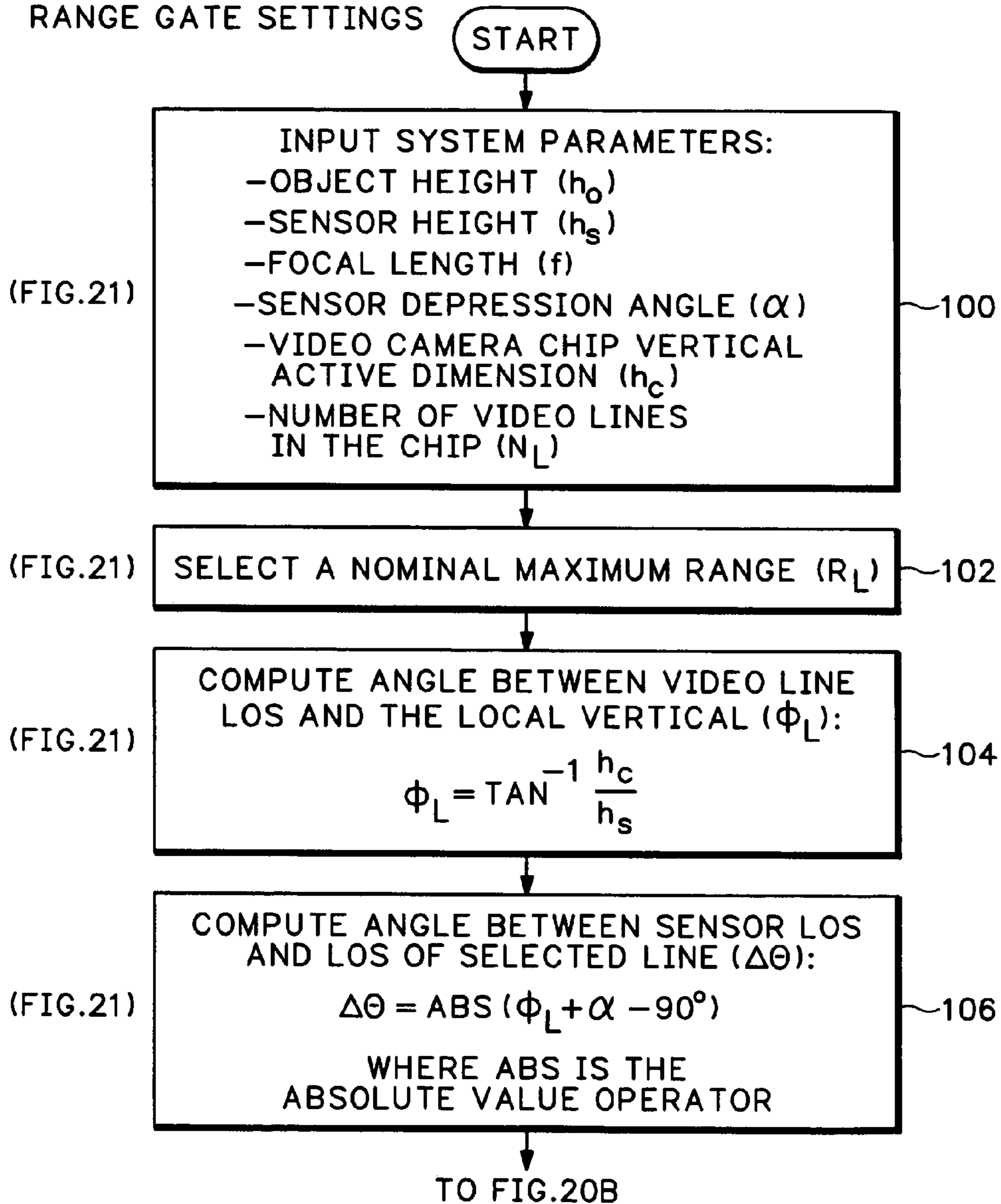
FIG. 20A
