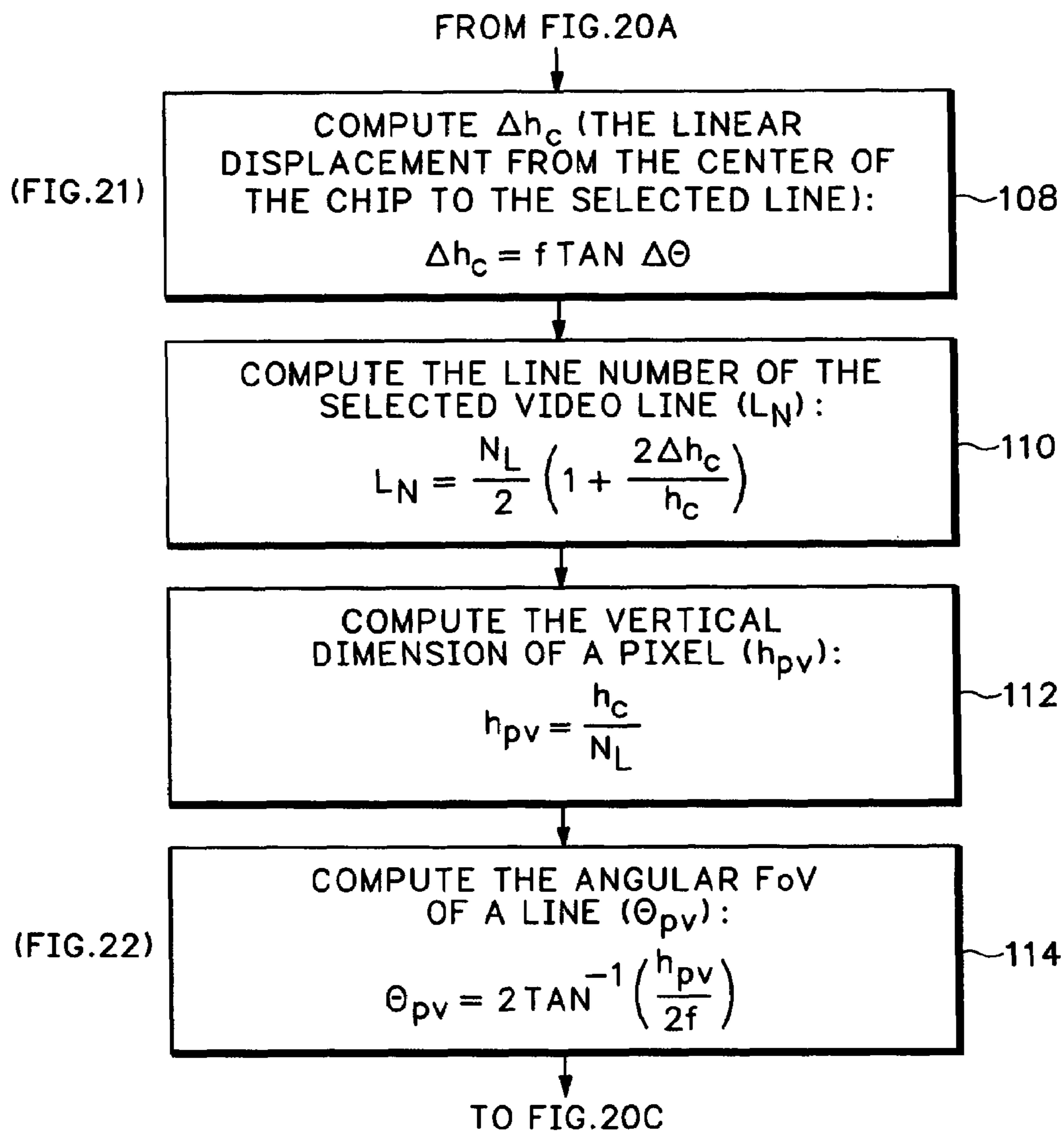
FIG.20B
