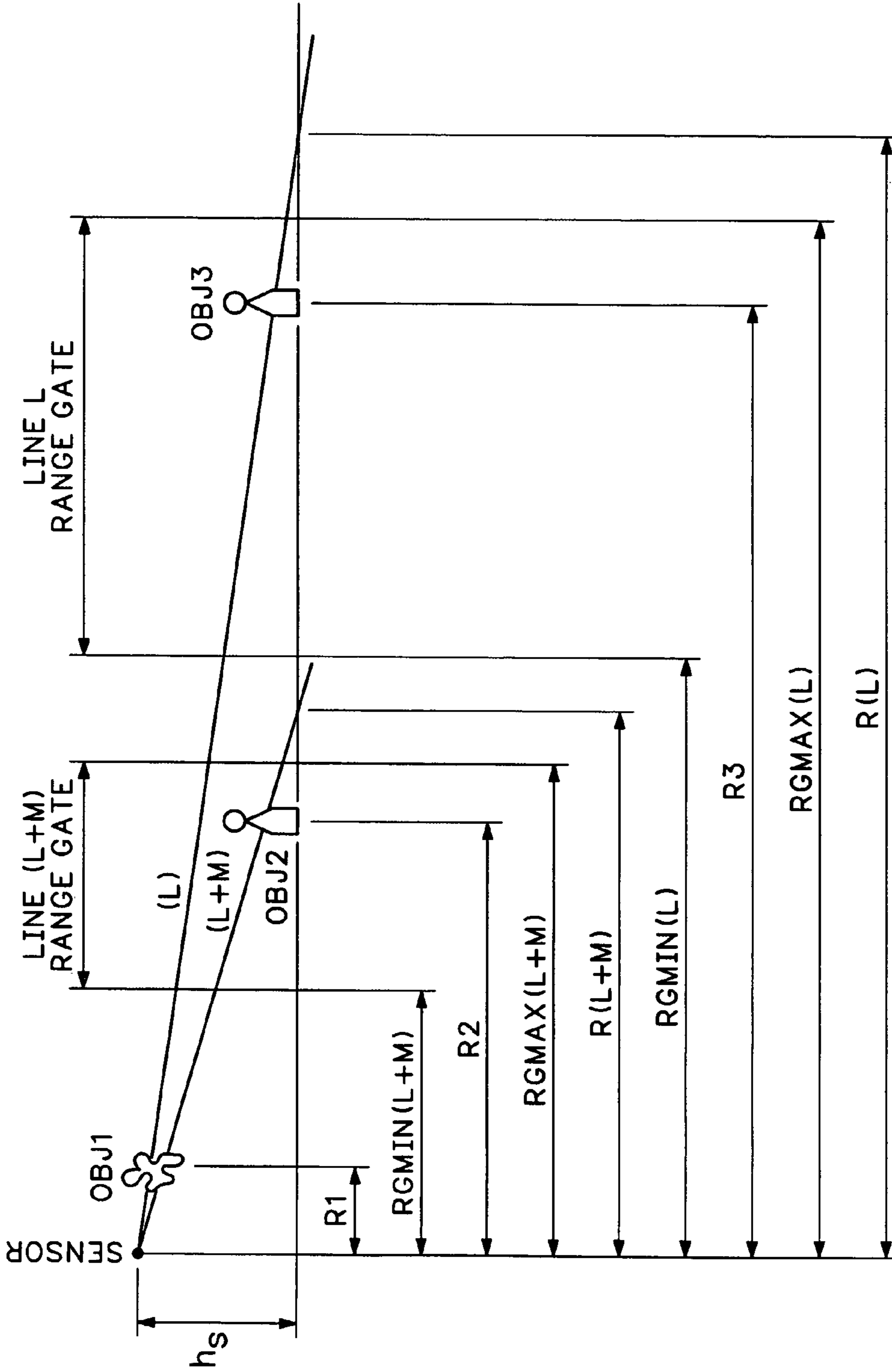
FIG.18
