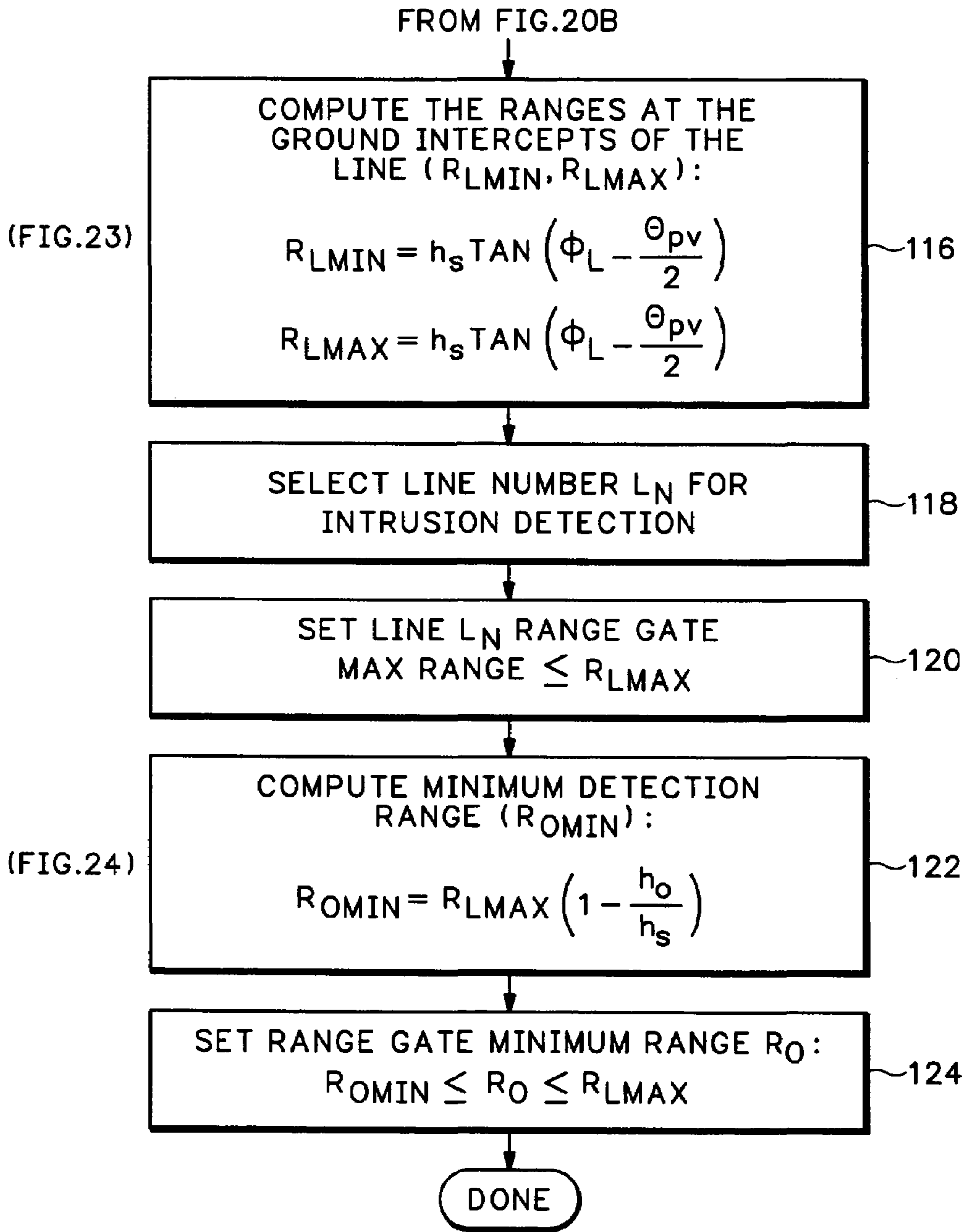
FIG.20C
