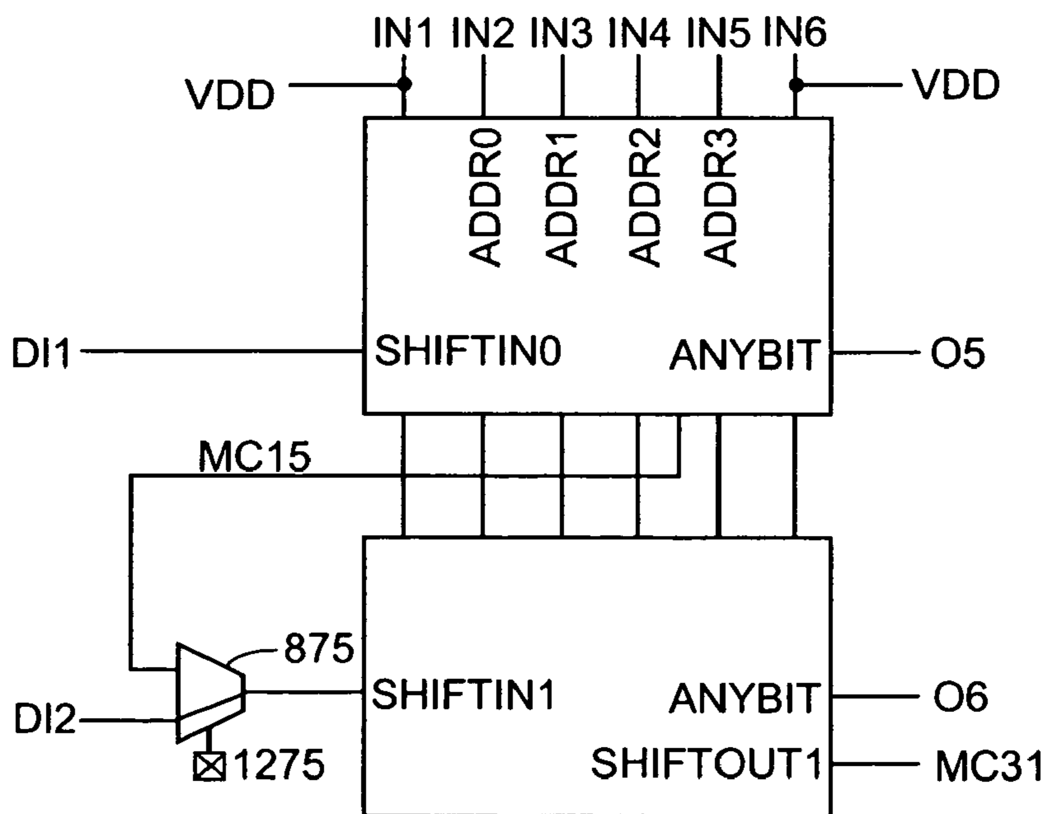
FIG. 13 (16x2 SRL)
