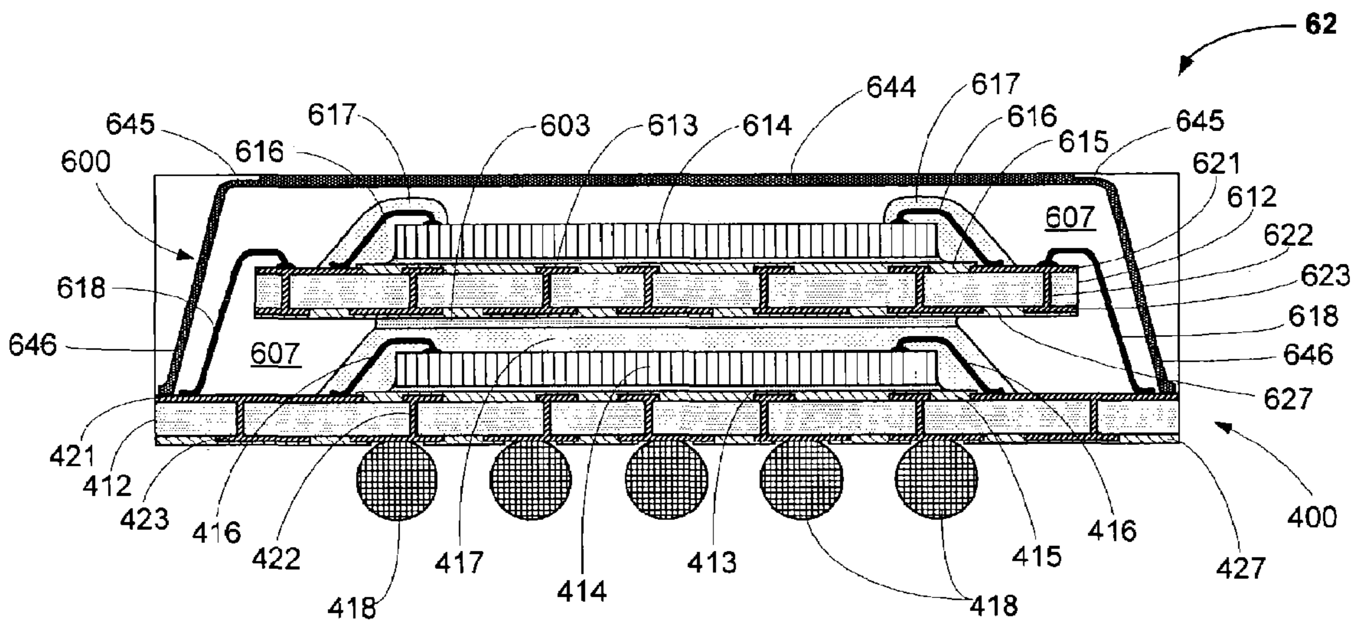
Fig. 6B
