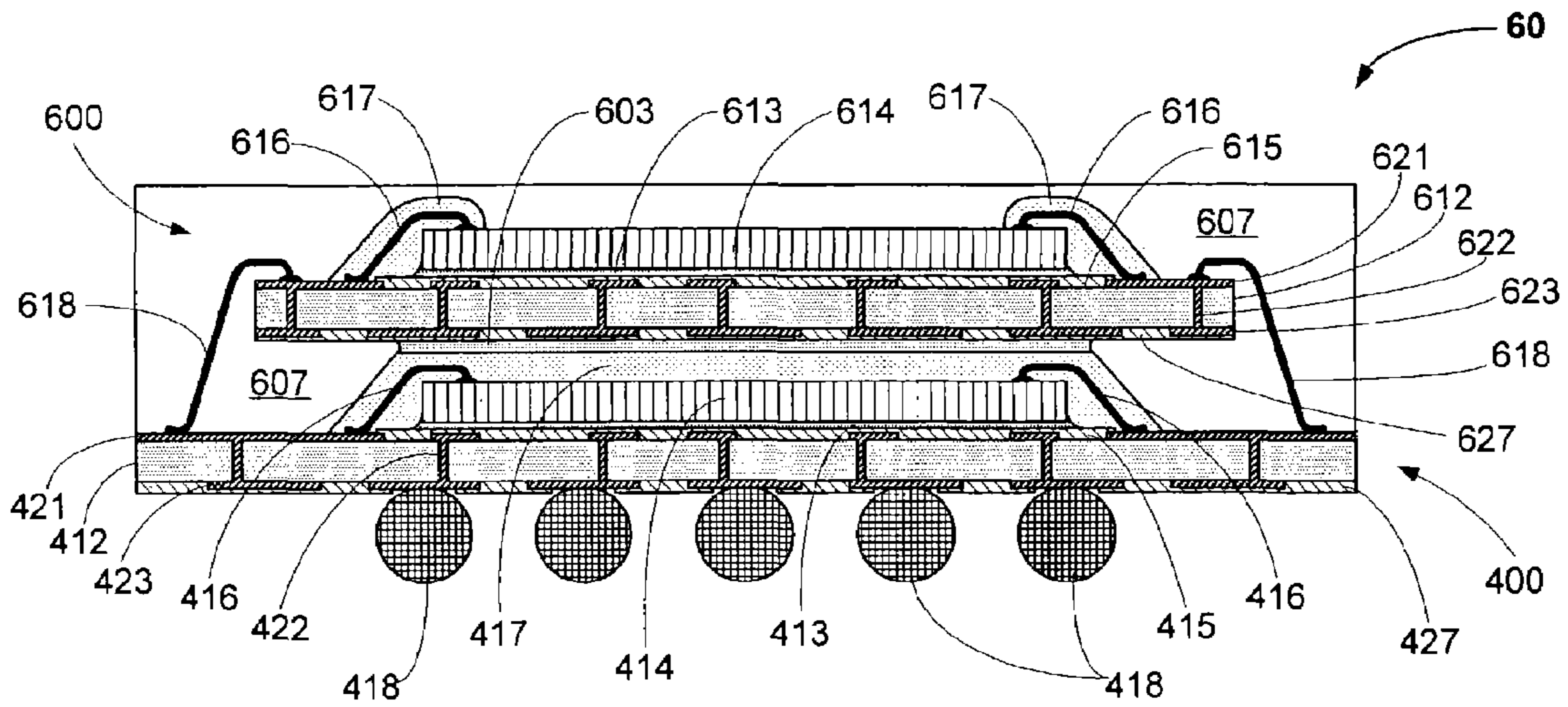
Fig. 6A
